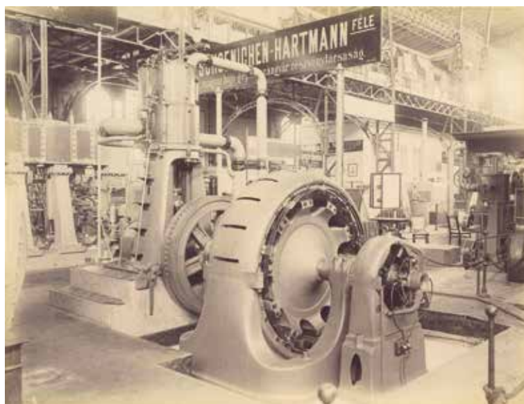
10. KÉP. A SCHOENICHEN-HARTMANN-FÉLE EGYESÜLT HAJÓ-, GÉP- ÉS KAZÁNGYÁR PAVILONJA AZ EZREDÉVES KIÁLLÍTÁSON, 1896
