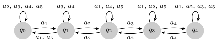
Fig. 3: The automaton \mathcal{V}_5
