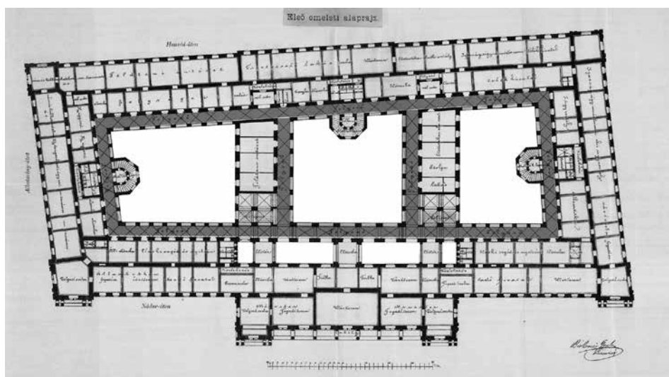
1. ábra. A Földművelésügyi Minisztérium épületének megvalósult I. emeleti alaprajza a belső udvarok (fehér) és a folyosók (sötétszürke) jelölésével. Forrás: Építő Ipar 11 (1887. december 18.) 51., képmelléklet
