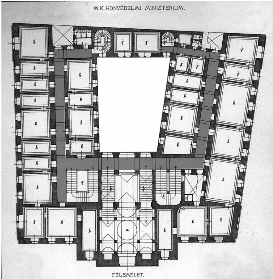
2. ábra. A Honvédelmi Minisztérium épületének félémeleti alaprajza a belső udvar (fehér) és a folyosók (sötétzürke) jelölésével. Forrás: Rozinay István: Budapesti építményei . Budapest 1883. t. 23.
