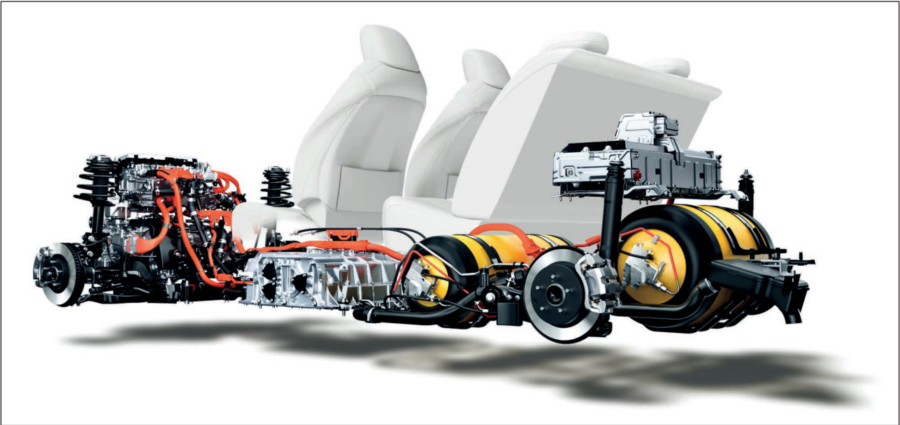
4. ábra. A Toyota Mirai hidrogéncellás szedán meghajtórendszerének ábrája
