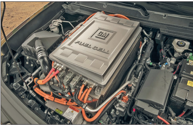
10. ábra. A Fort Carsonban tesztelt Chevrolet Colorado ZH2 terepjáró „erőműve”
