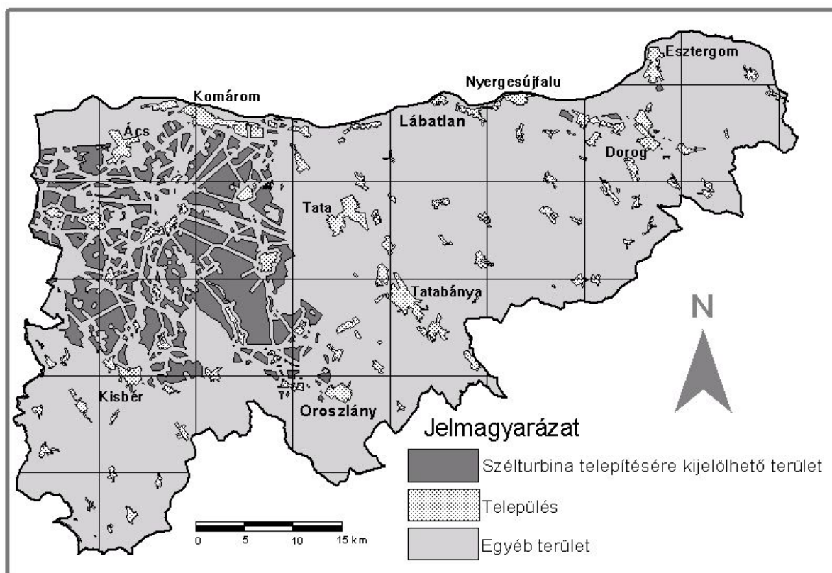
1.térkép: Jogszabályi szempontból szélturbina telepítésre alkalmas területek Komárom-Esztergom megyében (szerk: Kovács G. – Tóth J.)
