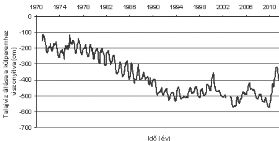
15. ábra A talajvízszint változása a 1416-os számú talajvízszint-észlelő kútban (Kecel, 1971–2012) Országos Vízháztartási Adattár adatai alapján
