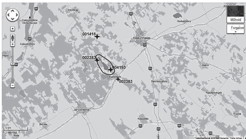
12. ábra A vizsgált talajvízszint-észlelő kutak elhelyezkedése a kiskunhalasi Fehértónál Figure 12. Situation of the examined water table monitoring wells near Fehértó of Kiskunhalas
