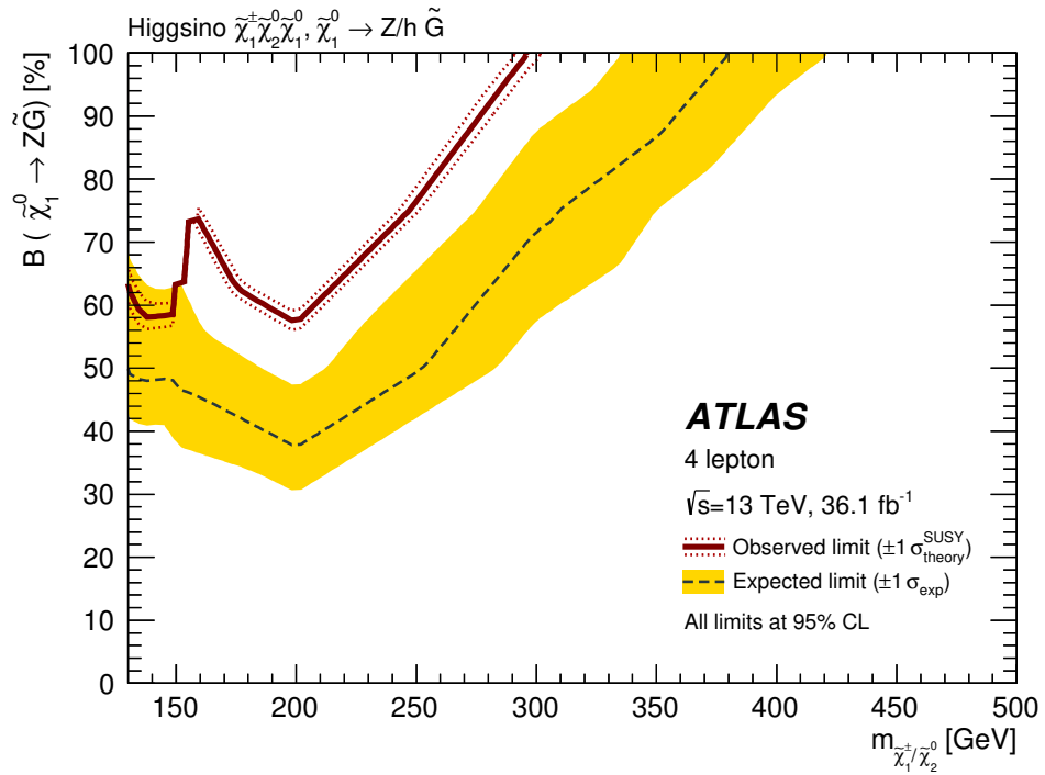
(a) RPC GGM higgsino
