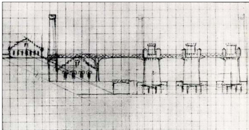
10. ábra. Péch Antal rajza a vajdahunyadi nagyvolvasztókról
