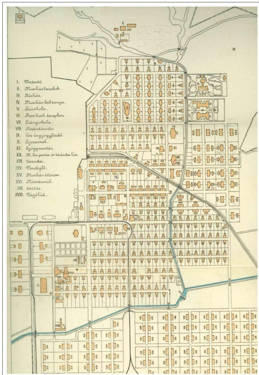
9. ábra. A gyári gyarmat (lakótelep) helyszínrajza [12]
