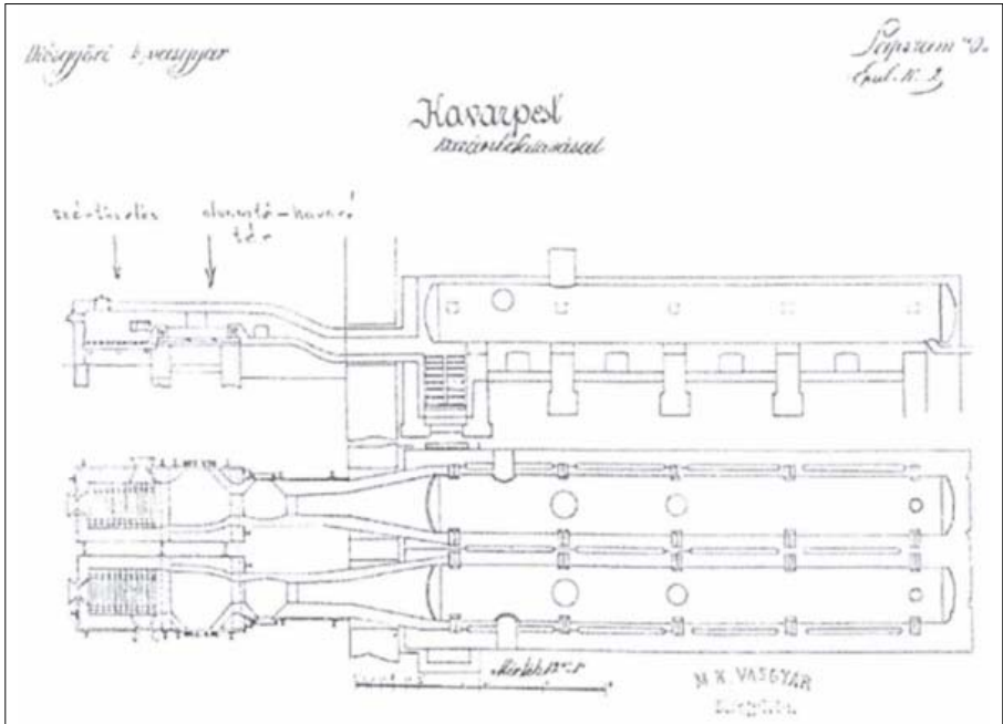
2. ábra. A diósgyőri „kavarpest” kavarókemence terve
