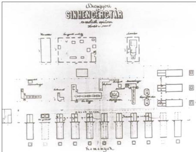
3. ábra. A diósgyőri sínhengergyár, az ún. Ó-hengermű telepítési rajza
