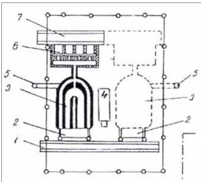
7. ábra. Az első diósgyőri Siemens–Martin-kemence telepítési vázlat. 1 – ingotárok, 2 – kemence, 3 – regenerátor, 4 – előmelegítő kemence, 5 – kémény, 6 – generátor, 7 – salakcsatorna
