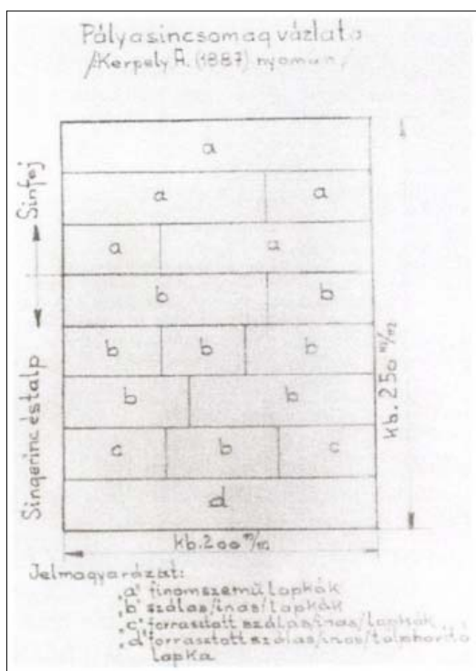
4. ábra. Síncsomag összeállítás Kerpely A. javaslata szerint
