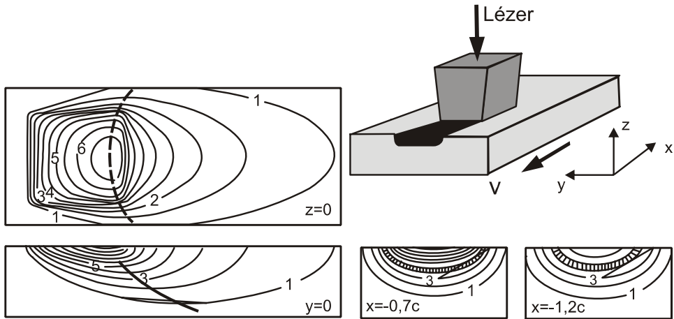
2.22. ábra Hőmérséklet-eloszlás lézeres felületedzésnél [Bergmann, 1994]
