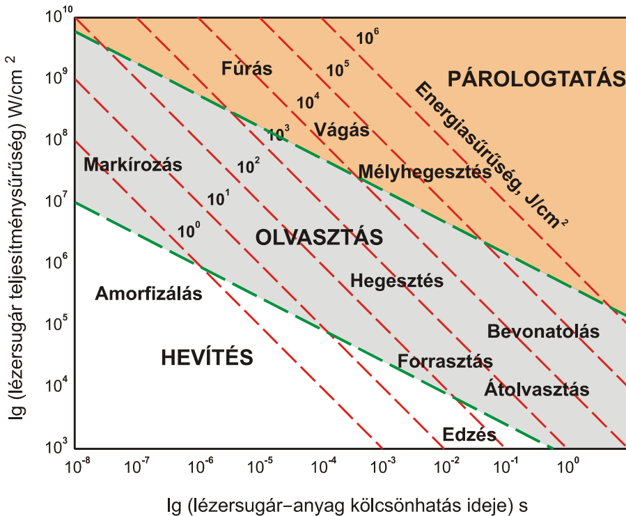
2.3.a. ábra A lézeres anyagtechnológiák alkalmazásának paramétertartományai [Steen, 1998; Grum, 2002; Búza, 2006]
