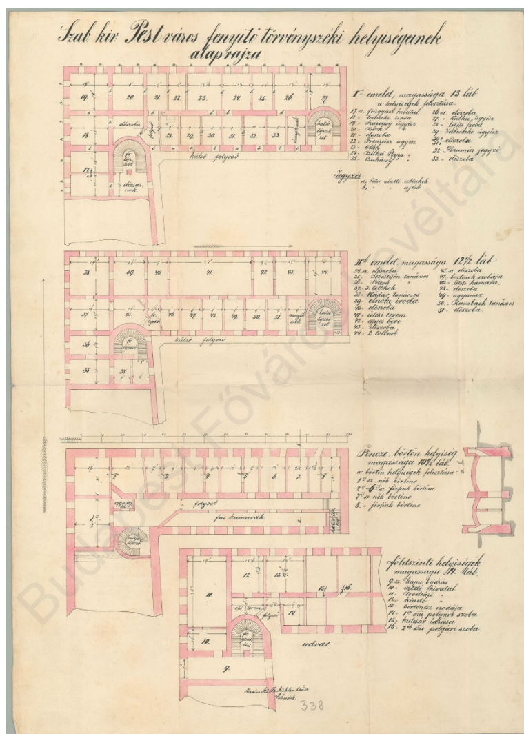
16. kép. A Tarcsalovits-laktanya átalakítás utáni berendezési terve, I-II. emeleti alaprajz (részlet). 1871. (BFL IV.1303.f XI. 334/1861. 338. p.)
