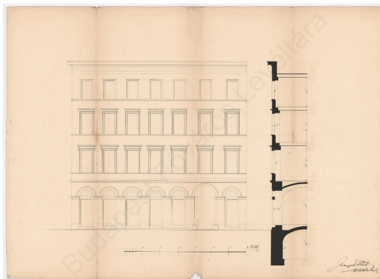
3. kép. A terézvárosi rendőrfőnökség épülete, homlokzat és metszet. Király u. 40., ún. Robicsek-ház, épült: 1844, tervezte: Hild József. ( BFL XV.17.b.311.10579 )
