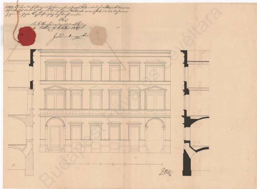
14. kép. A Tarcalovits-ház: a második emelet ráépítése utáni homlokzat és metszet. Épült: 1847, tervezte: Hild József. ( BFL XV.17.b.311.12021 )
