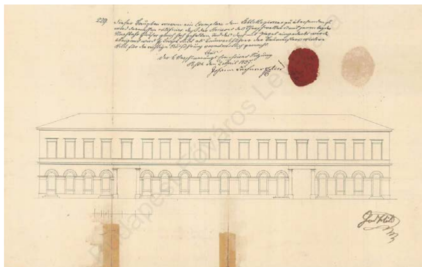
4. kép. A józsef-, és ferencvárosi rendőrfőnökség épületének homlokzata, volt Stáció utca 21., ún. Alter-ház, épült: 1837, tervezte: Hild József. ( BFL XV.17.b.311.509b )
