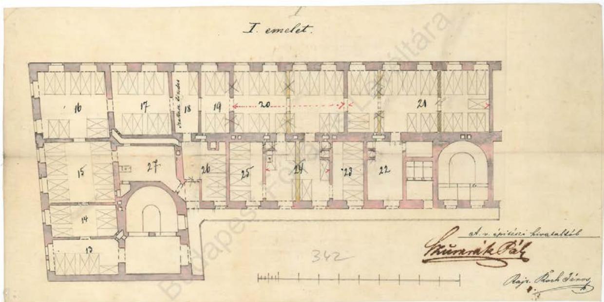
15. kép. A Tarcalovits-laktanya átalakítási tervei 1861-ből. I. emeleti alaprajz (részlet). ( BFL IV.1303.fXI. 334/1861. 342. p. )
