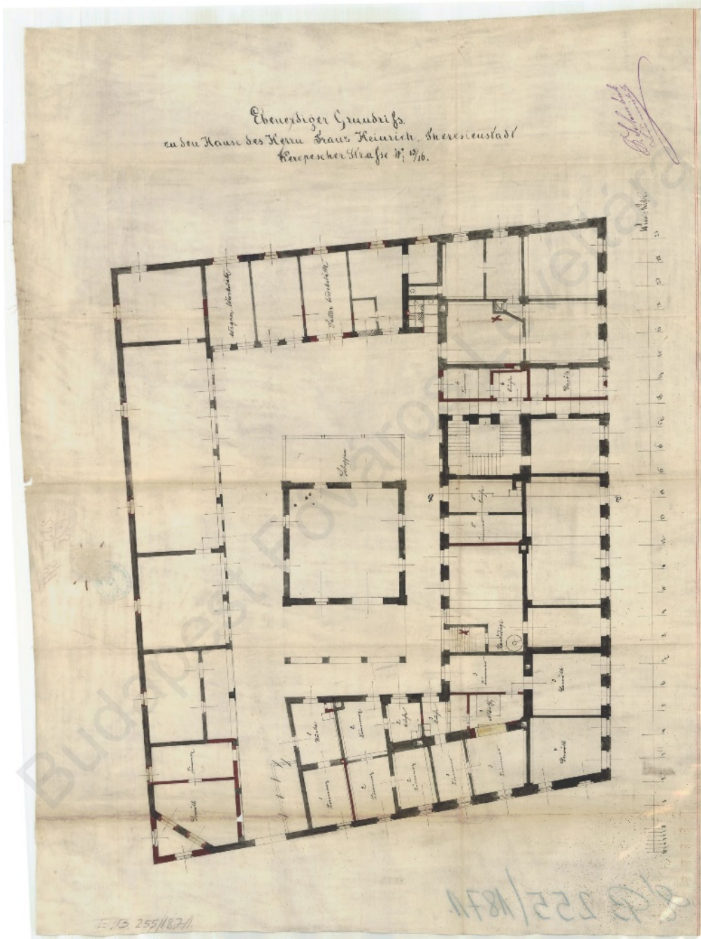
11. kép. A „Heinrich-ház” átépítése, földszinti alaprajz. Épült: 1871, tervezte: Schusbeck Pál. ( BFL XV.17.312. 255/1871 )
