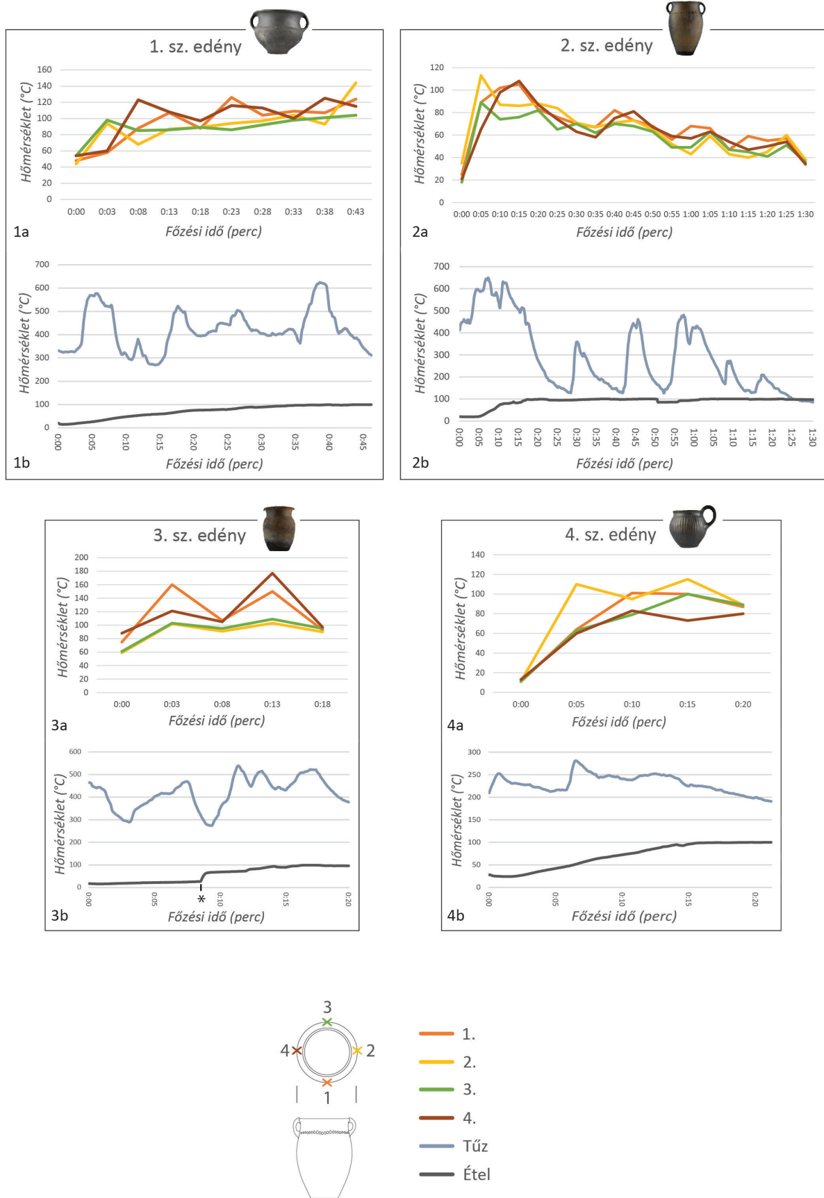
4. kép. 1a–4a, a külső edényfelület négy pontján mért felületi hőmérsékletek a főzési idő alatt (mérési gyakoriság: 5 perc); 1b–4b, a tűz és az étel hőmérséklete a főzési idő alatt (mérési gyakoriság: 5 másodperc; * – a hirtelen hőmérsékletváltozás a hőelem elmozdulásának köszönhető)
