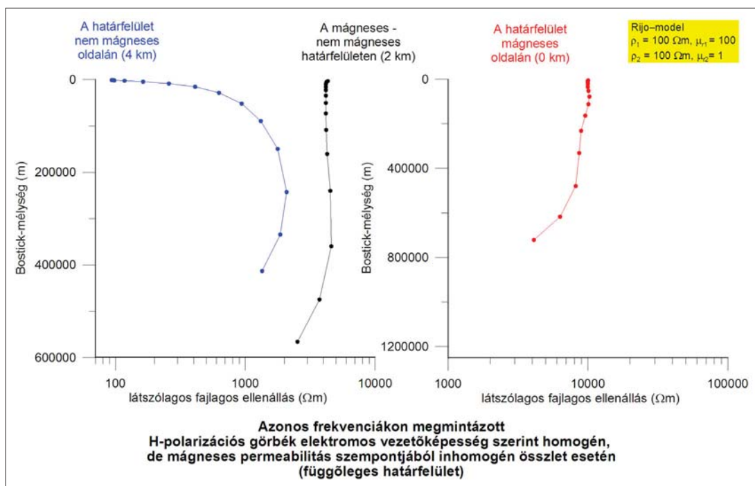
17. ábra Homogén vezetőképességű összetételben egy erősen mágneses test hatása a határfelület előtt, a határfelületen és a határfelület után H-polarizációban (logaritmus x tengely mentén, modell: 2. ábra)
