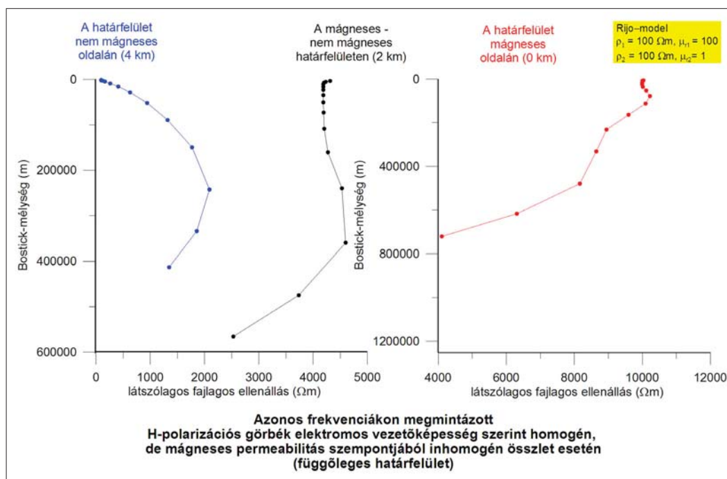
18. ábra Homogén vezetőképességű összetételben egy erősen mágneses test hatása a határfelület előtt, a határfelületen és a határfelület után H-polarizációban (lineáris x tengely mentén, modell: 2. ábra) Figure 18 The effect of a strongly magnetic body in a homogeneous conductivity ensemble, before, at and after the interface in H-polarization (along the logarithmic x axis, model: Fig. 2)
