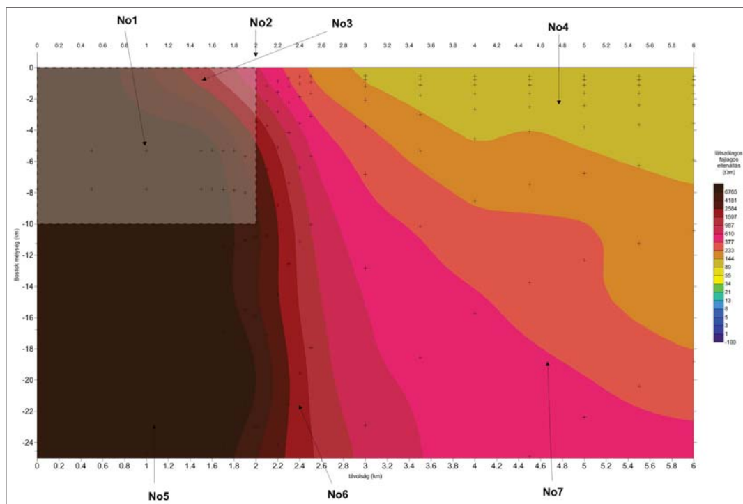
11. ábra | A direkt modellezésből kapott látszólagos fajlagosellenállás–mélységmetszet H-polarizációban (távolság–mélység szelvény, No1–No7 torzulások)
