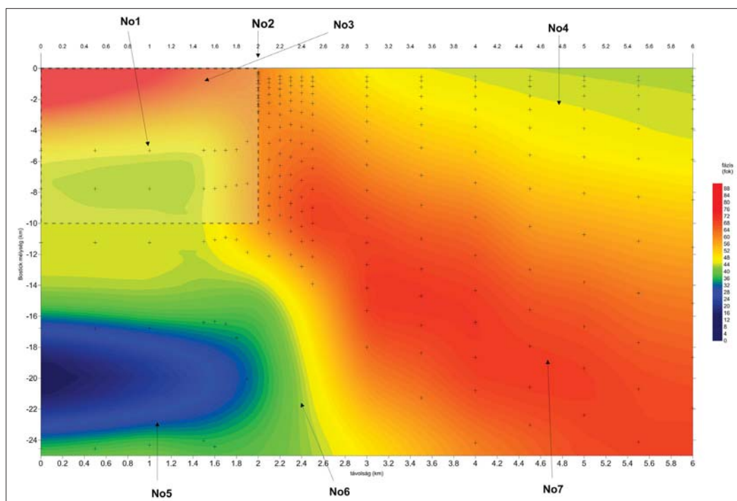
10. ábra | A direkt modellezésből kapott fázis–mélység metszet E-polarizációban (távolság–mélység szelvény, No1–No7 torzulások)
