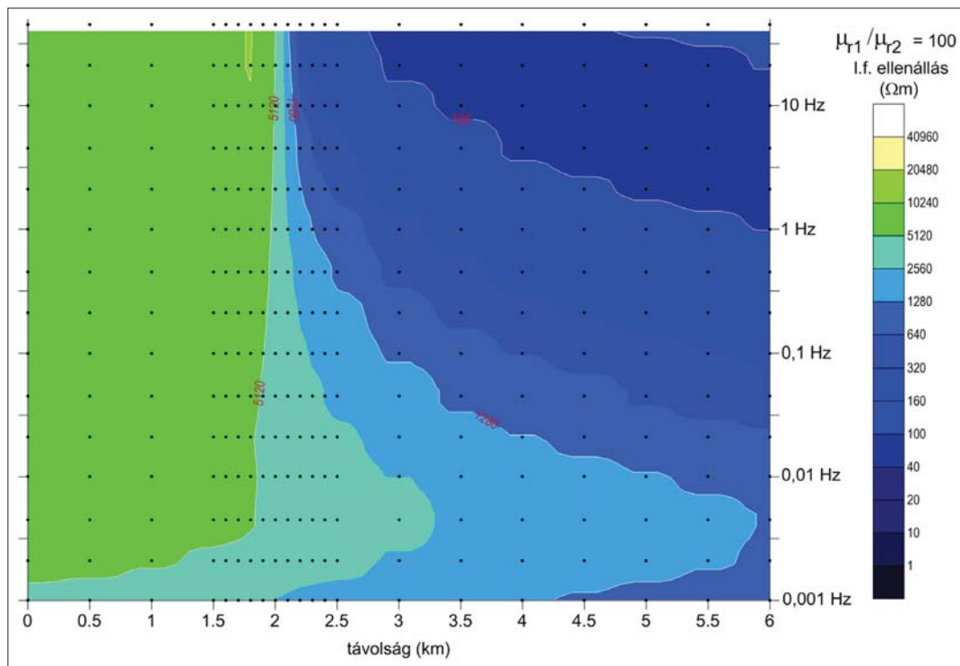
5. ábra A direkt modellezésből kapott H-polarizációs látszólagos fajlagosellenállás-szelvény (távolság–frekvencia). (A mintázást fekete pontok jelzik, amelyek a frekvencia szerint egységesen mintázzák meg a frekvenciateret.)
