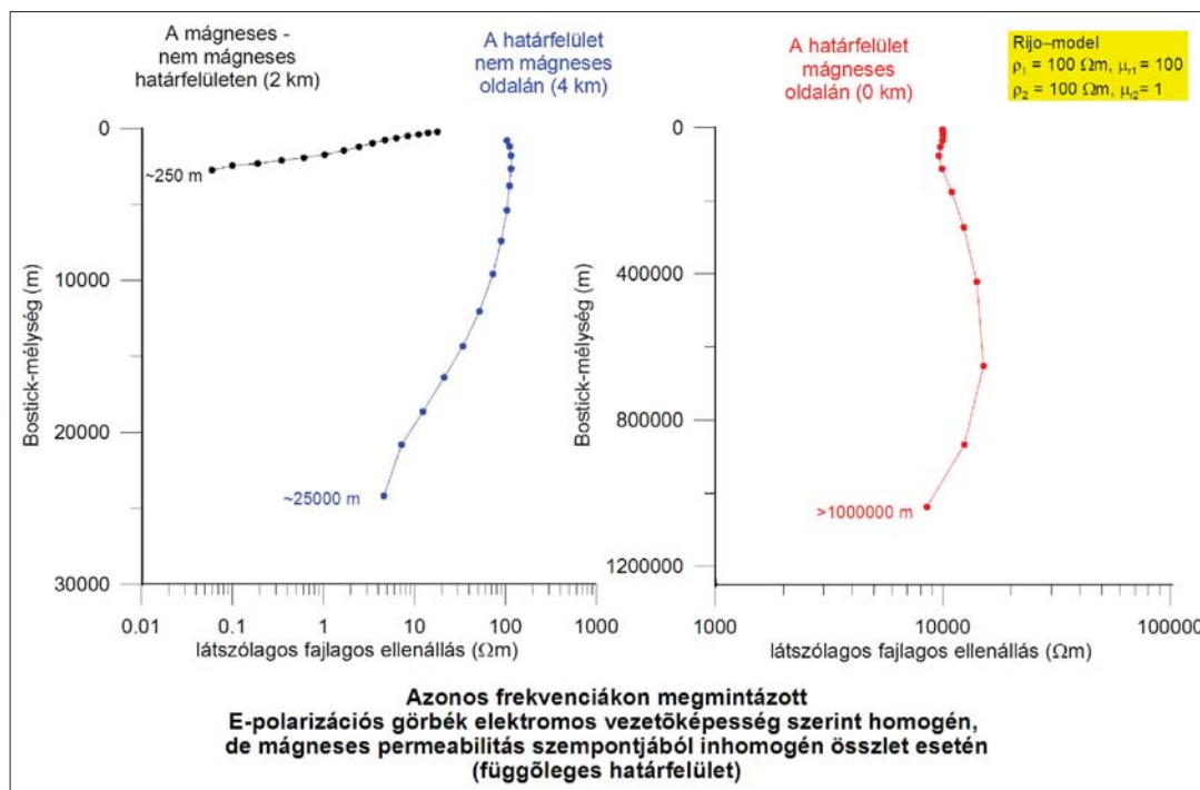
15. ábra Homogén vezetőképességű összetételben egy erősen mágneses test hatása a határfelület előtt, a határfelületen és a határfelület után E-polarizációban (logaritmus x tengely mentén, modell: 2. ábra)
