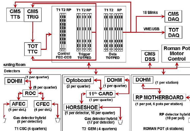
Fig. 28. The TOTEM trigger logic diagram.
