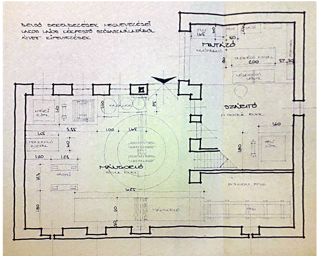
2. kép. A műhely alprajza a berendezésekkel
