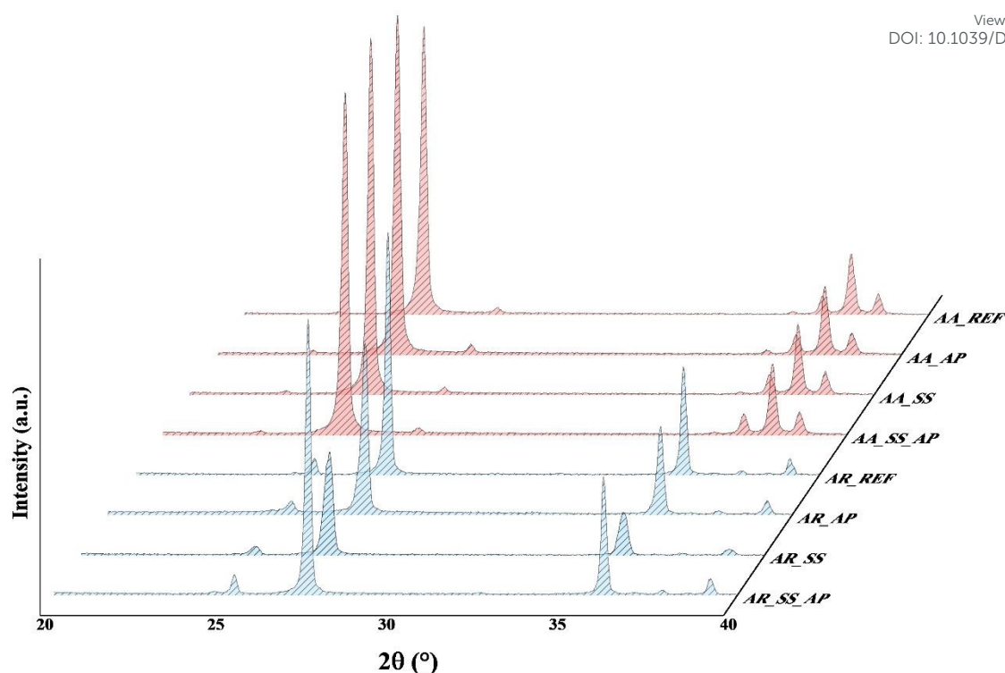
Fig. 3. XRD patterns of TiO 2 NPs
