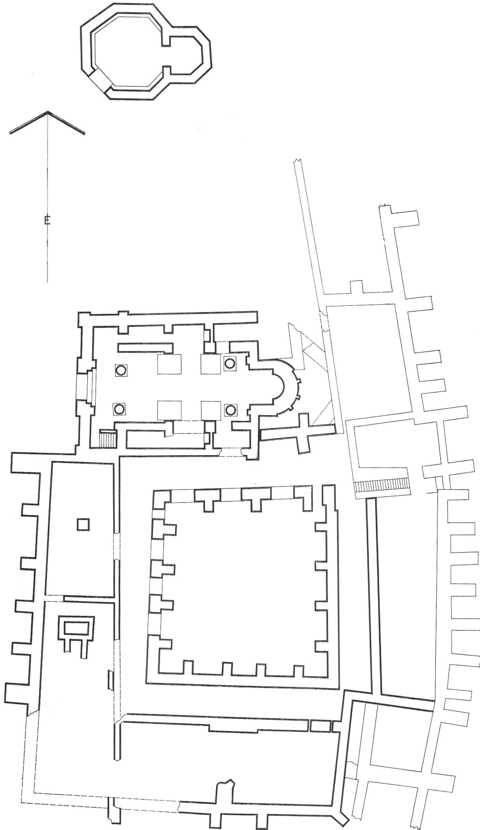
73. A kaposzentjakabi bencés apátság alaprajza. – Grundrisse der Benediktinerabtei von Kaposzentjakab.
