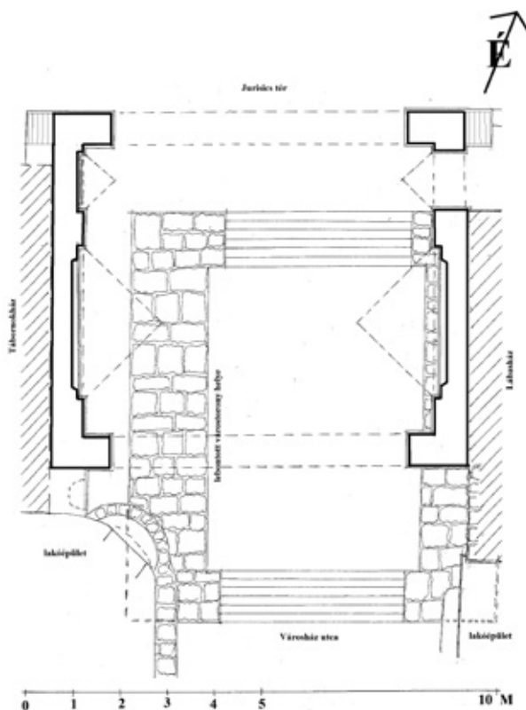
A burkolatban bemutatott Alsókapu-torony alaprajza. Felmérés és rajz: Ivicsics Péter 2023.
