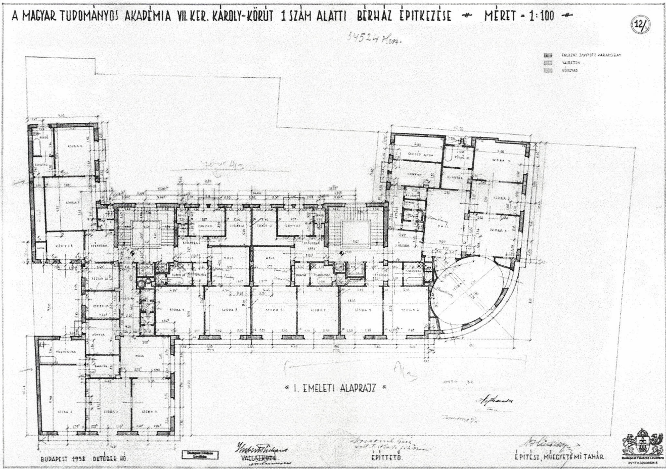
5. kép Hüttl Dezső: A Magyar Tudományos Akadémia bérházának engedélyezési terve. Első emeleti alaprajz, 1938 (BFL)
