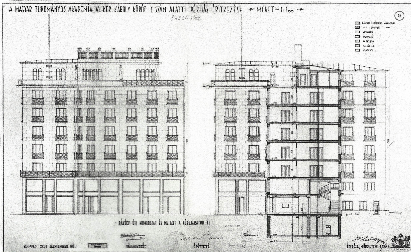
6. kép Hüttl Dezső: A Magyar Tudományos Akadémia bérházának engedélyezési terve. Rákóczi úti homlokzat és metszet a főbejáraton át, 1938 (BFL)
