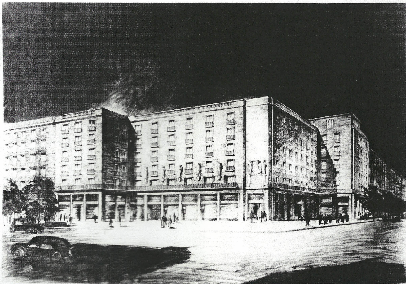
7. kép Kertész K. Róbert és Weichinger Károly: B jelű terv a Magyar Tudományos Akadémia bérházához. Távlati kép, ceruzarajz, 1937 (MTAKK)
