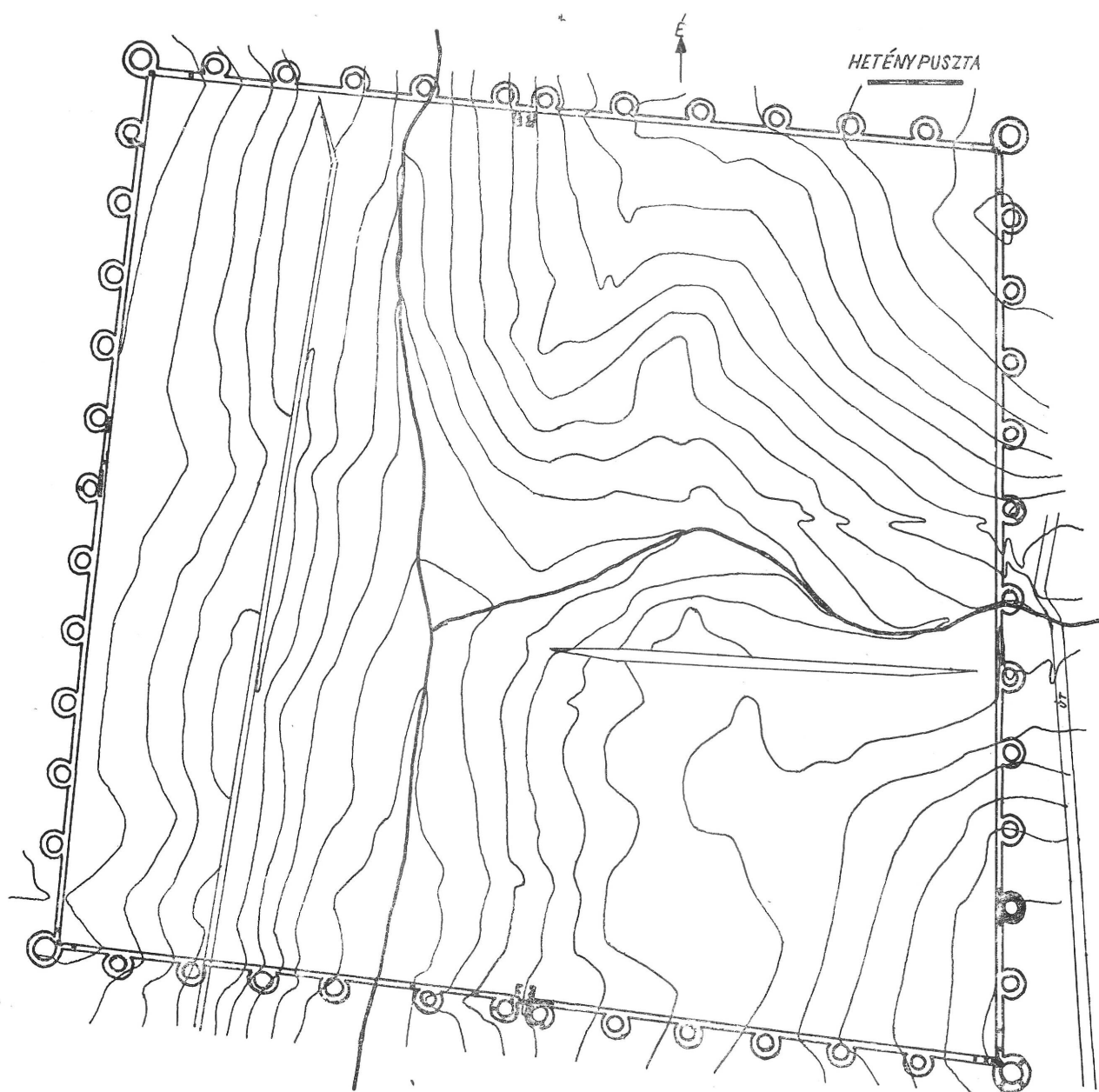
38. Kaspupa–Alsóhetény. A római erőd alaprajza. – Grundrisse der römischen Festung in Alsóhetény. 1:400
