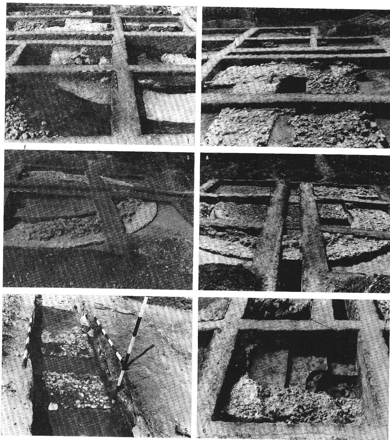
XVII. Kapospula–Alsóhetény. 1: az erőd déli kaputornya (43. sz. torony), 2: a déli kapu propugnaculuma a lekövezett úttal, 3: a keleti fal 35. sz. tornya, 4: a keleti fal 35. számú tornya, 5: a déli kapu első periódusban épített lekövezett útja, 6: a déli kapu patkó alakú 45. tornya. — Kapospula–Alsóhetény. 1: südlicher Torturm der Festung (Turm Nr. 43), 2: Propugnaculum des Südtors mit der gepflasterten Strasse, 3: Turm Nr. 35 in der Ostmauer, 4: Turm Nr. 35 in der Ostmauer, 5: die in der ersten Bauphase errichtete Strasse mit Steinpflastern beim Südtor, 6: hufeisenförmiger Turm Nr. 45 beim Südtor.
