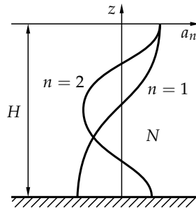
5.8. ábra. Állandó Brunt–Väisälä-frekvenciájú folyadék első két belső hullám normálmódusa: a_1(z) , a_2(z) . Az ábra a vezető rendben érvényes eredményt mutatja. A normálmódusok zérushelyei (5.54) szerint a vízszintes sebesség előjelváltását jelzik, az n -edik módusban tehát a közeg n+1 ellentétes irányban mozgó rétegre bomlik.
