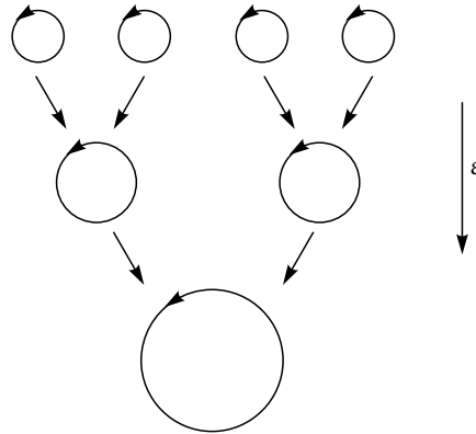
7.6. ábra. Az inverz energiakaskád. A kétdimenziós turbulenciában a kis örvények egyre nagyobbakká olvadnak össze. A rajtuk átfolyó \varepsilon energiafluxus állandó. Az ábra adott előjelű örvényeket mutat, az ellenkező forgásúak természetesen hasonlóan egyesülnek.
