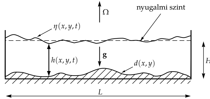
2.1. ábra. A forgatott, sekély homogén folyadék (a sarkok környékén vagy a laboratóriumban) és a fejezetben használt jelölések: a felület nyugalmi szinthez viszonyított alakját az \eta(x, y, t) függvény, az aljátétét a d(x, y) írja le. A folyadék átlagos H mélysége sokkal kisebb az L vízszintes kiterjedésnél.
