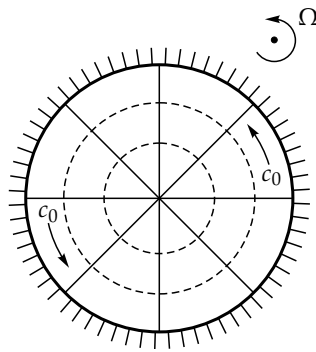
2.15. ábra. Kelvin-hullám haladása egy kör alakú medencében pozitív forgatás esetén (felülnézet). A folytonos vonalak az azonos fázisú helyeket kötik össze, a szaggatottak pedig az azonos amplitúdómaximumokat. Az amplitúdó a medence közepén a legkisebb, és a perem felé növekszik.
