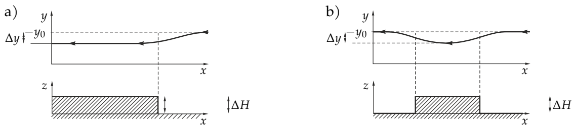
10.4. ábra. A domborzat hatása keletről érkező áramlásokra. a) Lépcső b) Véges domborzati elem
