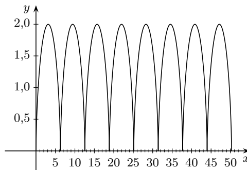
1.3. ábra. Mozgás az y irányba mutató, állandó a_0 gyorsulást okozó erő és a Coriolis-erő hatására, nyugalomból indítva, pozitív forgásirány esetén. A távolságot az a_0/(2\Omega)^2 dimenziótlán egységben mérjük. A pálya (csúcson) ciklois. [A cikloisok paraméteres egyenlete x = t - e \sin t , y = 1 - e \cos t , e = 1 -re csúcson, e > 1 -re hurkolt ciklois.]
