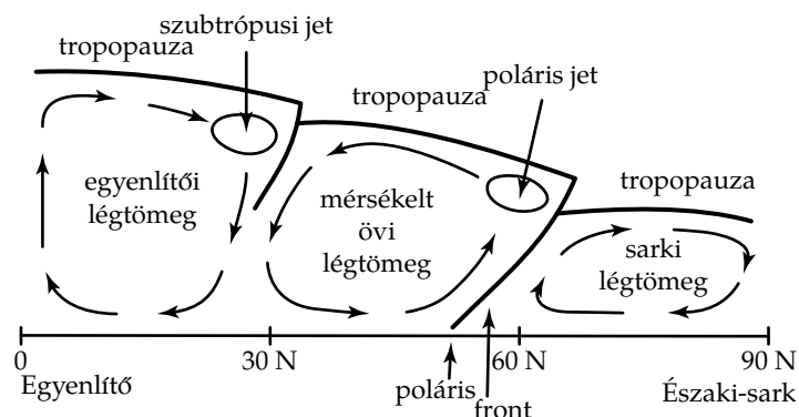
6.21. ábra. A globális légkörzés magasságfüggésének sematikus rajza az északi féltekén, benne három cellával és a jetekkel. Az egyenlítői cellát szokás Hadley-cellának is nevezni. G. Hadley (1685–1768) angol meteorológus, első vizsgálója annak, hogy a Föld forgása hogyan befolyásolja a légkör térbeli áramlását, aki még egyetlen, az Egyenlítőtől a sarkig terjedő cellát jósolt.
