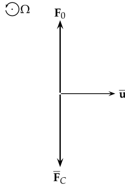
1.4. ábra. Az F_0 külső erő olyan mozgást alakít ki, amelyben az \bar{F}_C átlagos Coriolis-erő vele ellentétes lesz, és a hosszú idejű mozgás állandó \bar{u} átlagsebességű, a külső erőre merőleges irányban.
