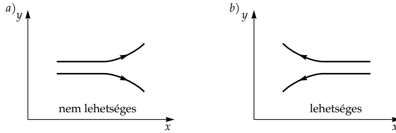
10.2. ábra. A potenciális örvényesség megmaradásával a sík aljzat felett nyugatról keletre történő áramlás eltérülése nincs összhangban (a). A keletről érkező áramlás viszont eltérülhet (b). A jelenség mindkét féltekén érvényes.
