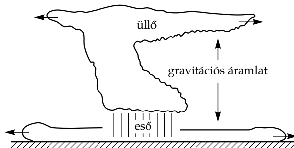
12.12. ábra. A zivatar előszele és a felhő üllőjének mozgása is gravitációs áramlat.
