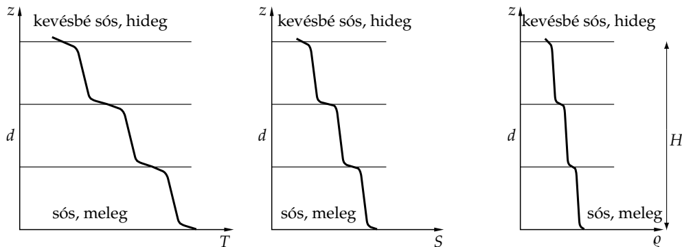
12.18. ábra. Rétegeképződés: Az eredetileg felfelé egyenletesen csökkenő hőmérséklet és sótartalom hatására a kettős diffúziós instabilitás miatt közel homogén vízszintes rétegek alakulnak ki, amelyekben turbulens termikus konvekció zajlik.
