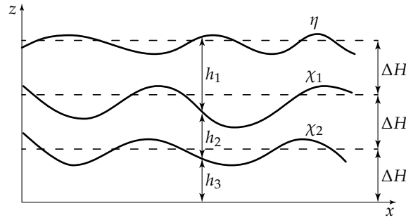
13.4. ábra. A folytonos rétegzettség dinamikájának megértéséhez használt háromrétegű közelítés geometriája. A 2. réteg tekinthető egy sokrétegű közelítés tipikus rétegének.
