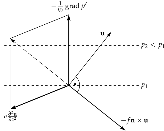
4.2. ábra. A nyomási, a viszkózus és a Coriolis-erő egyensúlya Ekman-rétegben a gyors forgatás határesetében. Az \mathbf{u} sebesség eltér a geosztrofikustól, és az alacsonyabb nyomás felé mutató komponense is van.
