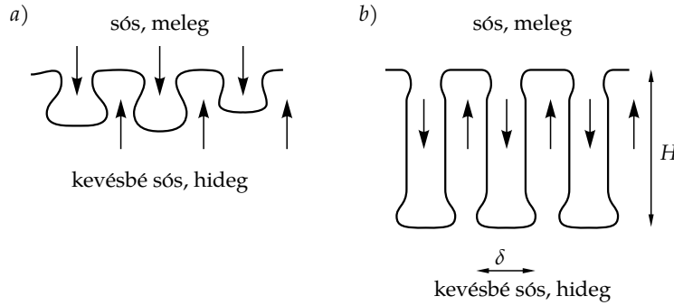
12.17. ábra. Ujjasodás a) A só-ujjak képződésének kezdeti fázisa b) Kifejlett állapot
