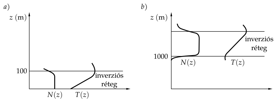
12.5. ábra. a) Talajközeli inverzió. A Brunt–Väisälä-frekvencia nagy, ezért az áramlások közel két-dimenziósak. Az energiacsere gyenge az egymás fölötti vízszintes rétegek között. b) Leáramlási inverzió. A planetáris határréteg jól kevert, benne a Brunt–Väisälä-frekvencia nincs értelmezve, az inverziós rétegben viszont hirtelen nagy a Brunt–Väisälä-frekvencia. A két réteg között energiacsere és anyagkicserélődés alig van.
