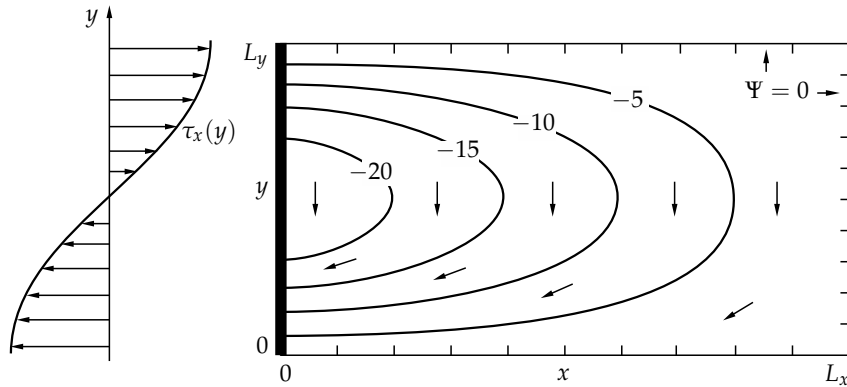
4.13. ábra. Óceáni medence és az uralkodó szelek által kifejtett nyírásból adódó egyszerű modell az északi féltekén. A (4.62) megoldással leírt áramvonalak mellé írt számok a \Psi mélységi áramlási függvény értékét adják Sverdrupban kifejezve ( 1 \text{ Sv} = 10^6 \text{ m}^3/\text{s} ). A vastag vonal erős nyugati part menti peremáramlatot jelöl, amely a növekvő y irányban (északra) áramlik.
