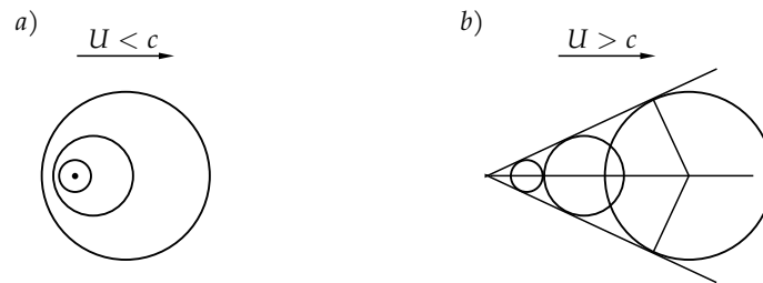
12.7. ábra. A vízszintes síkban pontszerű forrásból terjedő belső hullámok által elérhető tartomány U sebességű áramlásban. a) Szubkritikus, b) szuperkritikus áramlás. Az ábrán a c paraméter a belső lineáris hullámok terjedési sebessége.
