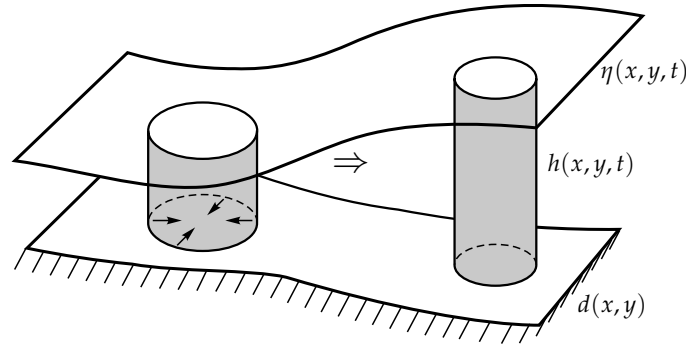
2.2. ábra. A sekély folyadék áramlása oszlopokban történik: mélyebb folyadékban az anyagmegmaradás miatt az oszlopok keskenyebbek lesznek.
