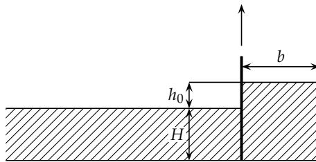
9.6. ábra. A folyadék kezdeti alakjának paraméterei balra haladó szolitonok keltésekor laboratóriumban. A felfelé mutató nyíl a rekesz falának kihúzását jelzi.
