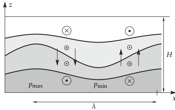
13.5. ábra. A \lambda = 2\pi/k_x , k_x > 0 hullámhosszú belső Rossby-hullám szerkezete folytonos rétegzettségű közegben ( n = 1 módus). A vonalak állandó sűrűségű felületeket jelölnek, a körök nagysága az y irányú sebesség abszolútértékével arányos, a bennük levő jelek az irányra utalnak. A nyilak a függőleges áramlás irányát mutatják abban a tartományban, ahol az a legerősebb.
