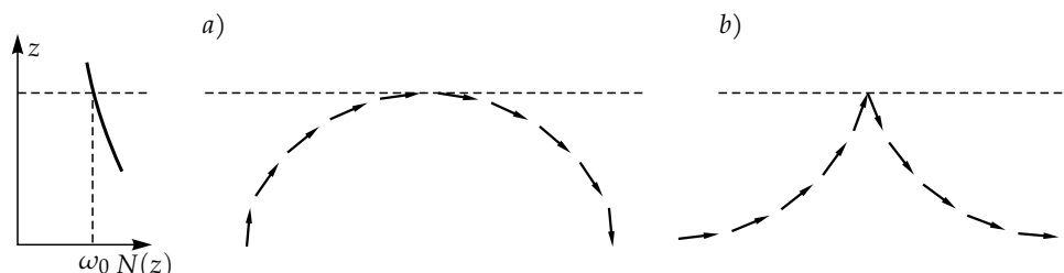
12.3. ábra. \omega_0 frekvenciájú belső hullám terjedési irányának változása felfelé gyengülő rétegzettség esetén. a) A hullámszámvektorok változása haladás közben. b) A csoportsebesség-vektorok változása haladás közben. Az N = \omega_0 szinten (szaggatott vonal) teljes visszaverődés történik.
