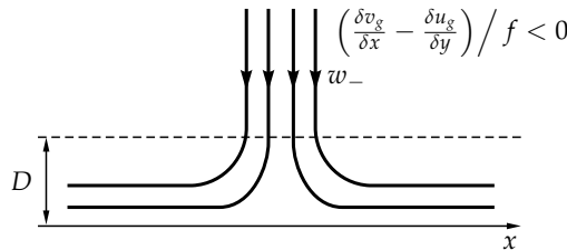
4.5. ábra. Az Ekman-pumpálás a határrétegből a folyadék belsejébe irányuló függőleges áramlás, amelynek erőssége a folyadék belsejében jelenlevő geosztrofikus áramlás örvényességével arányos. A leáramláshoz ( w_- < 0 ) anticiklonális geosztrofikus mozgás tartozik, a feláramláshoz ciklonális.
