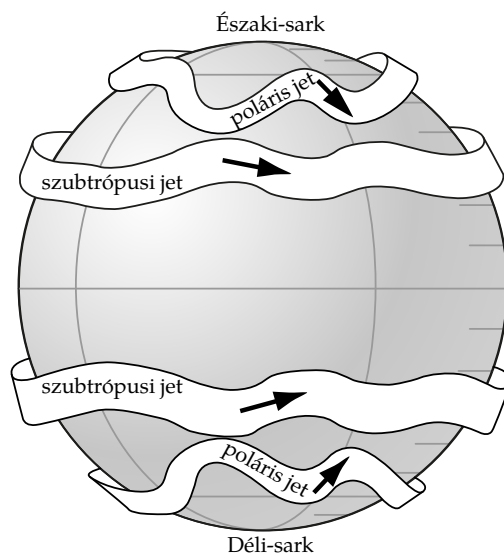
3.13. ábra. A földi magaslégkörben futó jetek sematikus képe
