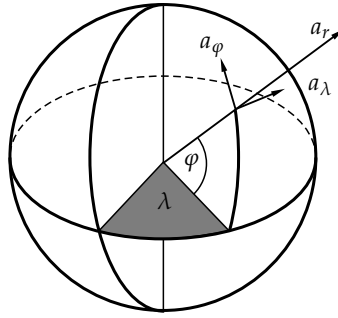
10.12. ábra. A gyorsulásvektor komponensei (álló) gömbi rendszerben
