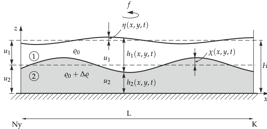
6.1. ábra. A Föld \varphi_0 szélességi köre érintősíkjában fekvő kétrétegű sekély folyadék. A koordináta-rendszer z tengelye a lokális függőleges irányba mutat, az x tengely a szélességi körökkel párhuzamos. A külső folyadékfelszín nyugalmi szinthez viszonyított alakját az \eta(x, y, t) , a \varrho_0 sűrűségű 1-es közeget a \varrho_0 + \Delta\varrho sűrűségű 2-es közegtől elválasztó belső felületét a \chi(x, y, t) függvény írja le. A folyadék átlagos H mélysége sokkal kisebb L vízszintes kiterjedésénél.
