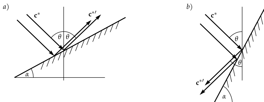
12.2. ábra. Belső hullám visszaverődése a vízszintessel \alpha szöget bezáró síklapon. A vonalak a csoportsebesség-vektor irányát mutatják. a) Lapos akadály a) Meredek akadály
