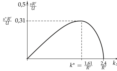
13.6. ábra. Az instabilitási ráta folytonos rétegzettségű közegben az f -sík-közelítésben. Az instabilitási tartomány és a leggyorsabban növekvő hullám k^* hullámszáma nem függ a termikus áramlás U sebességétől, a ráta azonban arányos vele.
