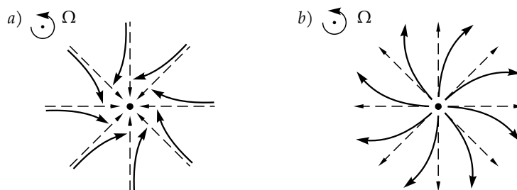
1.1. ábra. Forgatott rendszerben történő áramlások alaptulajdonsága. A le-, vagy feláramlás esetén az adott szinten történő össze- vagy szétáramlás nem maradhat sugárirányú a folyadékre- szecskékre ható Coriolis-erő miatt. Ez a hatás kis Rossby-szám esetén különösen jelentős. Pozitív forgásirány mellett az összeáramlás pozitív cirkulációt vagy örvényességet hoz létre (a), szét- áramlás pedig negatívát (b).
