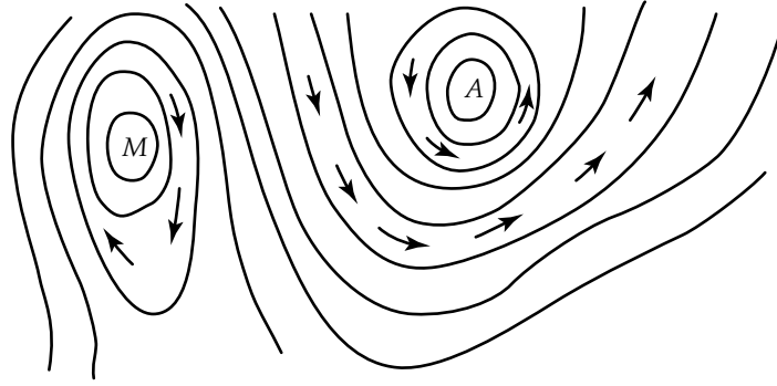
1.11. ábra. Általános geosztrofikus áramlás sematikus képe pozitív forgásirány esetén. A folytonos vonalak izobárok, a kis nyilak az áramlás sebességvektorát adják meg néhány helyen. A szomszédos izobárok folyómederként terelik az áramlást, más szóval az izobárok áramvonalak. Az A és M betűk alacsony, illetve magas szélsőértékű nyomási központokat jelölnek.
