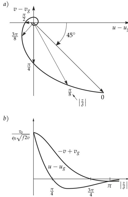
4.7. ábra. Áramlás a felső Ekman-rétegben az északi féltekén keleti irányba mutató nyírási vektor \tau_x > 0 , \tau_y = 0 esetén, (4.38) alapján: a) A különböző magasságokban kialakuló sebességeltérés vektorai. A spirál mellé írt számok a \delta egységekben mért mélységet mutatják. b) A sebességeltérés kelet–nyugati és észak–déli komponenseinek magasságfüggése. A határrétegbeli sebesség a D = \pi\delta mélységben (a határréteg peremén) jó közelítéssel megegyezik a folyadék belsejében jelenlevő \mathbf{u}_g geosztrofikus sebességgel.
