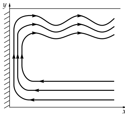
10.7. ábra. Zárt óceáni medencében kialakuló áramlás sematikus rajza a nyugati partvonal körül az északi féltekén
