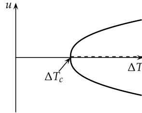
5.20. ábra. A konvekciós áramlás erősségének függése a hőmérséklet-különbségtől a \Delta T < 2\Delta T_c ( Ra < 2Ra_c ) tartományban. A függőleges tengelyen az adott helyre jellemző áramlási cella tipikus u sebessége látható. A szaggatott vonal instabil állapotot jelöl.
