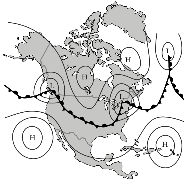
6.16. ábra. Tipikus frontvonalat, baroklin hullám felszíni képe és a front körüli ciklonok sora. A ciklonok közötti távolság néhányszor 1000 km nagyságrendű.
