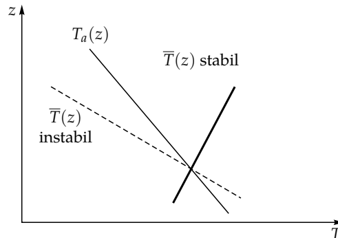
12.20. ábra. A \bar{T}(z) hőmérsékletprofil stabilitásának feltétele ideális gázban. A hőmérsékletnek az adiabatikus profilénál (vékony vonal) lassabban kell csökkennie (vastag vonal), és növekedhet is a magassággal. A szaggatott vonal instabil rétegzettséghez tartozik.
