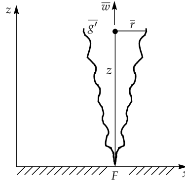
14.2. ábra. A kis méretű forrásból felszálló turbulens csóva legfontosabb paramétereit. A turbulens besodródás miatt a csóva felfelé vastagodik, a benne mozgó folyadékelemek lassulnak és sűrűsödnek.
