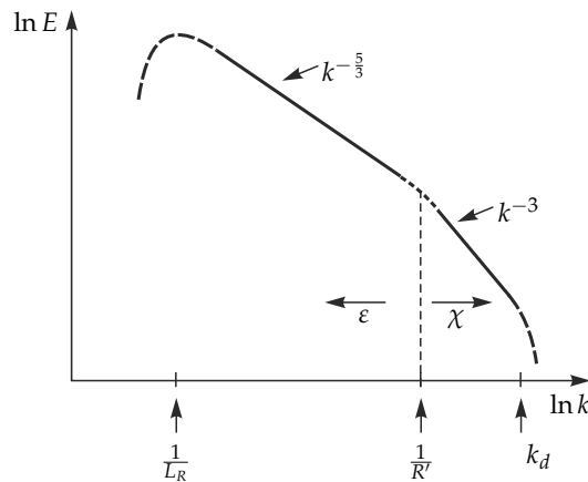
7.8. ábra. A geosztrofikus turbulencia energiaspektruma a \beta -síkon. k_0 \approx 1/R' és k_d \sim (\chi/\nu^3)^{1/6} a baroklin instabilitás energiabetáplálási hullámszáma, illetve a disszipációs hullámszám. Az inverz energiakaszkád az 1/L_R hullámszámig tart.
