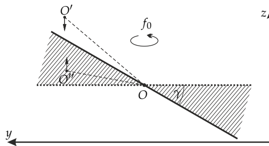
6.13. ábra. A baroklin instabilitás lehetősége termikus áramlásban. A folytonos rétegzettségű közegben a \gamma szöggel döntött sűrűségfelület (folytonos vonal) és a vízszintes sík (pontosított vonal) közötti (sátozott) tartományba eső elmozdulás a kiindulási helyzettől történő távolodást eredményez. A kiindulási helyzet az O-O'' elmozdulásra nézve instabil (az O-O' -re stabil).
