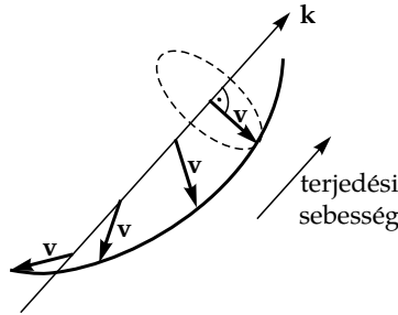
1.14. ábra. A sebességvektorok térbeli elrendeződése tehetetlenségi hullámban. Egy adott helyen a \mathbf{v} sebességvektor végpontja körpályán (szaggatott vonal) mozog.
