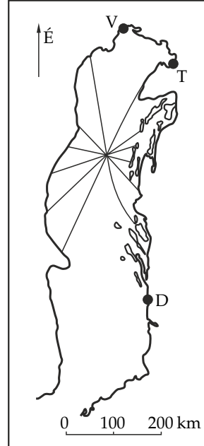
3.7. ábra. Az árapályhullám haladása az Adriai-tenger északi medencéjében. A vonalak a dagály óránkénti helyzetét jelzik, a körüljárási ciklonális (pozitív). A medence érintett tartománya közelítőleg egy 150 km széles, 400 km hosszú téglalap. A 100 m átlagos mélységgel számolt Rossby-sugár kb. 300 km, összemérhető a lineáris mérettel. A V, T és D pontok Velencét, Triesztet és Dubrovnikot jelölik.
