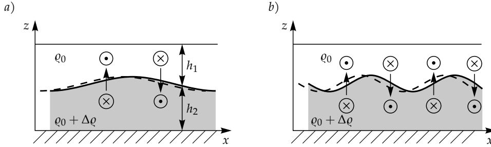
6.12. ábra. Belső Rossby-hullám kialakulása kétrétegű közegben, f_0 > 0 . (a) Lokalizált felső felszíni kidudorodás körüli kvázi-geosztrofikus áramlás a felső közegben ciklonális, az alsóban ellentétes irányú. A potenciális örvénység megmaradása következtében ez mindkét közegben leáramlást kelt a keleti (jobb) oldalon és feláramlást a nyugatin, amely a kidudorodást nyugati irányba tolja (szaggatott vonal). (b) Hullámalakú, y -ban eltolásinvariáns felső felszíni forma mozgása
