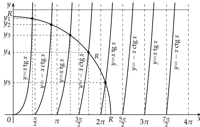
9.8. ábra. A V_0 mélységű potenciálgödör sajátenergiáira kapott egyenlet grafikusán ábrázolva. A megoldások a görbék metszéspontjai.
