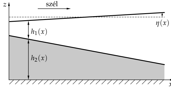
5.11. ábra. Az állandó szélnyírás következtében a tavak felszíne megdől. A belső elválasztó réteg (a termoklin zóna) ezzel ellentétes irányban és jóval nagyobb mértékben lejt.
