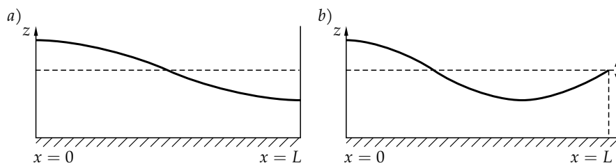
12.6. ábra. Állóhullámok (seichek) medencékben. a) Zárt medence, a leghosszabb állóhullám ( j = 1 ). b) Nyitott medence peremén ható gerjesztés hatására kialakuló állóhullám ( j \approx 2 ). Az ábrák felületalakot mutatnak, amely lehet akár a belső elválasztó felületé, akár a külső felszíné.
