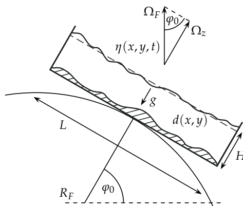
3.5. ábra. A földi áramlások derékszögű leírásához használt rendszer, valamely \varphi_0 szélességi (és tetszőleges hosszúsági) koordinátájú pont érintősíkjában. A sekély folyadékban lényeges Coriolis-hatásért felelős szögsebesség a Föld szögsebességének helyi \Omega_z függőleges komponense.
