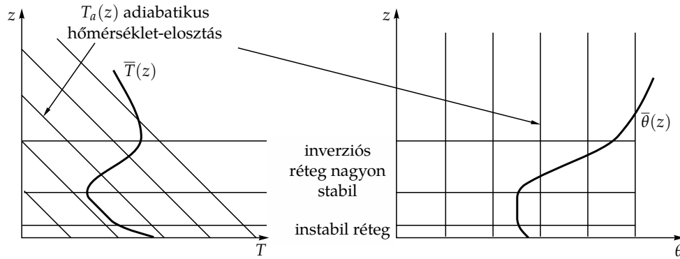
12.21. ábra. Az ideális gáz \theta potenciális hőmérsékletére történő áttérés a T, z sík olyan transzformációja, amely az adiabatákat függőleges egyenesekbe viszi át. Az inverziós réteget mindkét ábrázolásban jelöltük.
