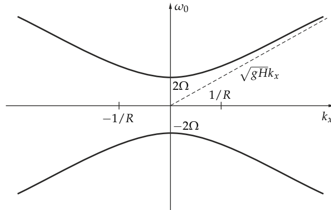
2.12. ábra. A tehetetlenségi gravitációhullám (Poincaré-hullám) diszperziós relációja (folytonos vonal) a hullámszám k_x komponensének függvényében ( k_y = 0 ). A szaggatott vonal a következő fejezetben tárgyalt Kelvin-hullám diszperziós relációja, ha az az x tengely mentén húzóódó peremmel párhuzamosan halad, amely tőle jobbra esik az északi féltéken.
