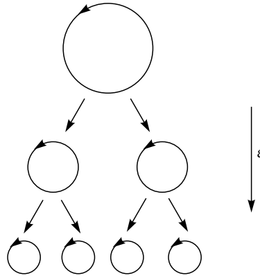
7.3. ábra. A direkt energiaskazkád. A háromdimenziós turbulenciában a nagy örvények egyre kisebbekre esnek szét. A rajtuk átfolyó \varepsilon energiafluxus az l_d disszipációs hosszának megfelelő legkisebb örvényméret eléréséig állandó. Az ábra adott előjelű örvényeket mutat, az ellenkező forgásúak természetesen hasonlóan bomlanak.
