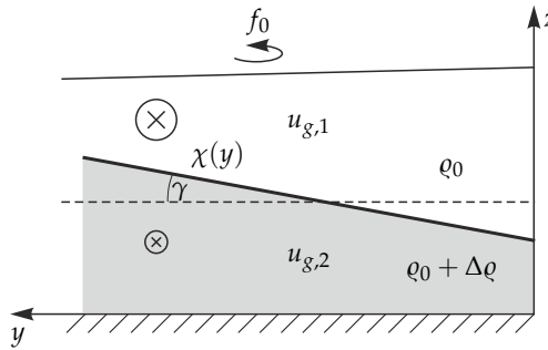
6.4. ábra. Geosztrofikus áramlás kétrétegű közegben. A belső elválasztó felületnek a közelebbi pólus irányában történő egyenletes emelkedése olyan stacionárius áramlással van egyensúlyban, amely keletre történik, és a felső (melegebb) rétegben gyorsabb, ott a sebesség nagyságát jelző kör nagyobb sugarú. A benne levő kereszt utal arra, hogy az áramlás a rajz síkjából kifelé mutat, a sebességvektort jellemző nyílnek mintegy a „tollazatát” látjuk, hátulról.
