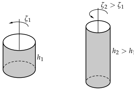
2.3. ábra. A potenciális örvényesség megmaradásának jelentése: mélyebb folyadékban az oszlopok forgása felgyorsul, összhangban az impulzusnyomaték megmaradásával.
