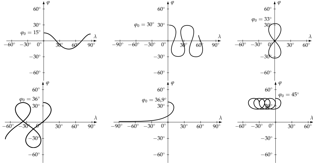
3.3. ábra. Az u_0 = 0,1 és v_0 = 0 dimenziótlan sebességgel megadott \varphi_0 szélességi szögű helyzetből keleti irányban meglökött testek pályái pozitív forgásirány esetén, a \lambda, \varphi síkon ábrázolva. A \varphi_c kritikus helyzetnek az ötödik ábra felel meg. Az utolsó ábra mutatja, hogy a síkon tehetetlenségi körmozgásnak megfelelő mozgás nagy gömbi méretben nyugatra sodródó spirálozássá változik.
