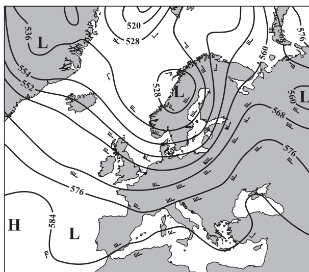
3.8. ábra. Tipikus meteorológiai térkép közepes magasságokban. A folytonos vonalak jó közelítéssel izobárok. A zászlókat alkotó minden egyes hosszabb vonalka 10 csomós (18,5 km/órás) szélesebbséget jelent, a rövidebbek fele ekkora sebességet (a kis háromszög 50 csomó). A H és L betűk magas, illetve alacsony nyomású központokra, anticiklonokra, illetve ciklonokra utalnak. A folytonos vonalak pontos jelentése: azokat a helyeket kötik össze, amelyekben az 500 hPa nyomás azonos magasságra esik (átlagos értékük 5,5 km körüli). A rájuk írt számok a z(p = 500 \text{ hPa}) magasságot jelölik deciméterben kifejezve, azaz a térképet nyomási koordinátában (10.1. fejezet) adják meg. Mivel a nyomásváltozás a vízszintes síkban gyenge, ezek a szintvonalak hasonlóan futnak, mint az azonos magassághoz tartozó izobárok.
