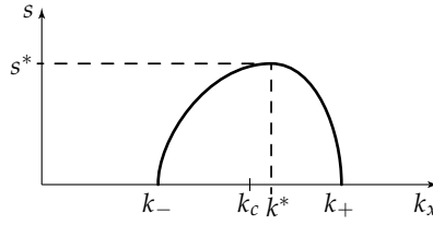
12.14. ábra. Sematikus ábra az instabilitási ráta függésére a k_x hullámszámtól adott \Delta U > U_c áramlási sebességre. A k < k_- tartományban a sűrűségkülönbség, k > k_+ -ra a felületi feszültség stabilizál.
