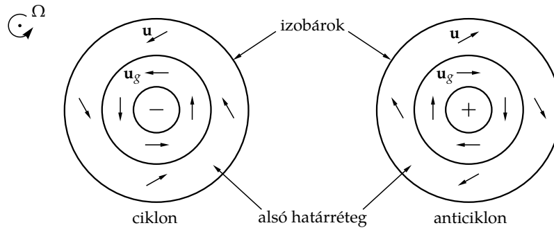
4.4. ábra. A szélsősebesség átlagos iránya ciklonok és anticiklonok alsó légrétegeiben az északi féltekén. A belső körgyűrű nyilai a magasban uralkodó geosztrofikus áramlást jelzik.
