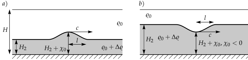
5.12. ábra. A belső szoliton az elválasztó felület kidudorodásával jár. Ez felfelé történik, ha az alsó réteg keskenyebb a felsőnél (a), és lefelé, ha az alsó réteg a vastagabb (b).
