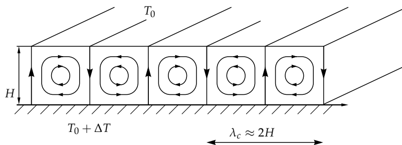
5.18. ábra. Stacionárius konvekciós áramlás. Közvetlenül a kritikus hőmérséklet-különbség (kritikus Rayleigh-szám) elérése után a peremektől távol szabályos, hengeres áramlási cellák alakulnak ki, ha a geometria (az oldalsó peremekkel együtt) y irányban eltolásinvariáns.
