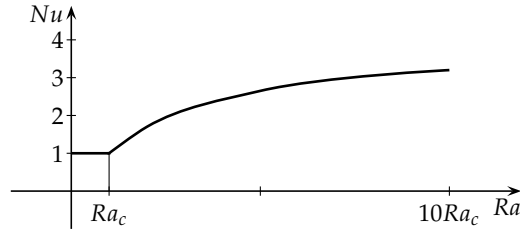
5.21. ábra. A Nusselt-szám függése a Rayleigh-számtól, az első instabilitást jóval meghaladó értékeig. A mérési eredményeket összefoglaló sematikus rajz
