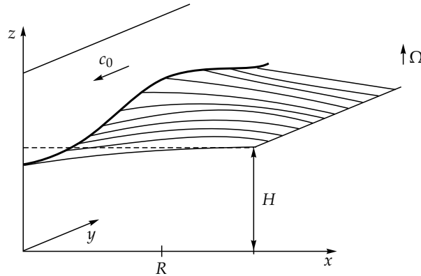
2.14. ábra. Kelvin-hullám egy y tengellyel párhuzamos partvonal mentén pozitív forgatás esetén. A hullám c_0 sebességgel halad, és amplitúdója a falra merőlegesen a Rossby-sugárnyi távolságon csökken e -ad részére.
