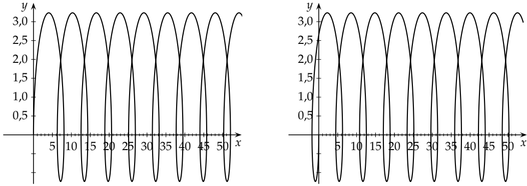
1.5. ábra. Mozgás az y irányban ható állandó erő és a Coriolis-erő hatására, y irányú kezdősebességgel. A dimenziótlan v_0 2\Omega / a_0 kezdősebesség a bal oldalon 2, a jobb oldalon -2 . Jól látszik, hogy a görbék, hurkolt cikloisok, azonosak, csak eltoltak a fázisok eltérő előjelének megfelelően.
