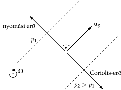
1.9. ábra. Erőviszonyok a geosztrofikus áramlásban: a Coriolis-erő a nyomási erővel ellentétesen egyenlő. Rájuk merőleges a kialakuló kétdimenziós geosztrofikus áramlás \mathbf{u}_g sebességvektora. A magasabb nyomás pozitív forgatás esetén a sebességvektor jobb oldalára esik.
