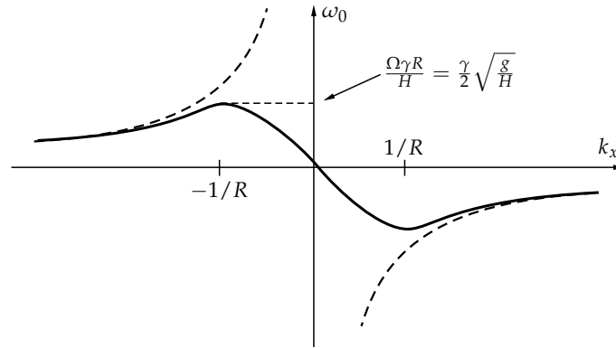
2.9. ábra. Az x irányban haladó ( k_y = 0 ) szabad felszínű Rossby-hullám diszperziós relációja a k_x hullámszámkomponens függvényében. A szaggatott görbe a zárt felszínű Rossby-hullám diszperziós relációja. A diszperziós reláció tetszőleges k_y mellett is hasonló, csak a szélsőértékek k_y -től is függenek.
