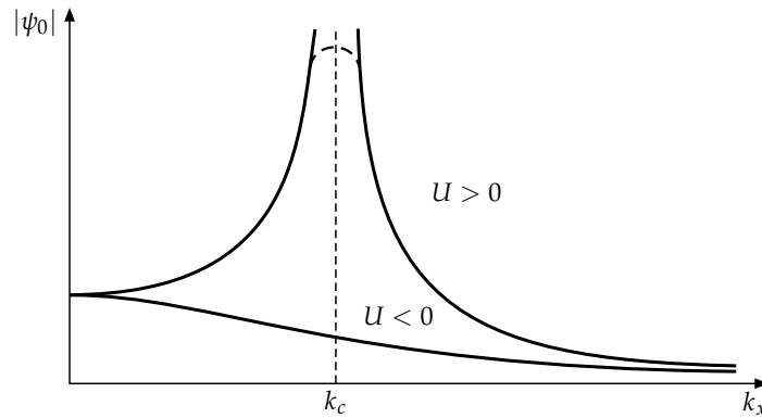
3.15. ábra. Hegységrendszer felett kialakuló stacionárius Rossby-hullám \psi_0 amplitúdója U sebességű háttéráramlásban a domborzat k_x hullámszámának függvényében az északi féltekén
