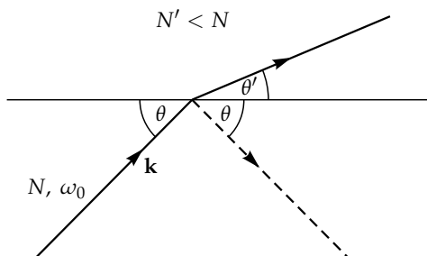
12.1. ábra. A belső hullám terjedési iránya (hullámszámvektorának iránya) megváltozik két különböző Brunt–Väisälä-frekvenciájú közeg határán. A gyengébb rétegzettségű közegben a hullám a vízszintes felé törik. A szaggatott vonal a visszavert hullám terjedési irányát mutatja. A csoportsebesség-vektorok \pi/2 - \theta , \pi/2 - \theta' szöget zárnak be a vízszintessel.
