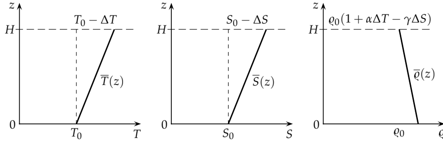
12.16. ábra. Az alapállapotú hőmérséklet-, sótartalom- és sűrűségprofil (felül meleg és sós közeg, de lefelé növekvő sűrűség), amely áramlással nem társul. Az előjel-konvenció szerint \Delta T, \Delta S < 0 . Ez az állapot instabillá válik egy kritikus pontban, ahol beindul az áramlás.
