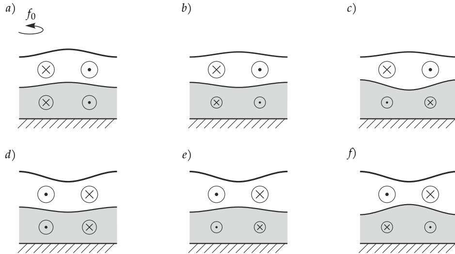
6.5. ábra. Geosztrofikus áramlás kétrétegű közegben a külső és belső felszíni alak viszonyának függvényében. A kis körökben levő pont (kereszt) a rajz síkjába (abból kifelé) mutató áramlási irányra utal, és ezt a konvenciót a későbbiekben is követjük. A külső felszín kiemelkedése alatt az áramlás mindig anticiklonális (a)–(c), de az alsó rétegben lassabb, ha a belső felszín változása ellenkező előjelű mint a külsőé (b), sőt előjelét is megváltoztathatja (c). Hasonló a helyzet a külső felszín behorpadása esetén is (d)–(f). Az ábra tekinthető az x, y síkon közel forgásszimmetrikus elrendezések oldalnézetének, de az y irányban eltolásinvariáns felszíni alakokhoz tartozóknak is.
