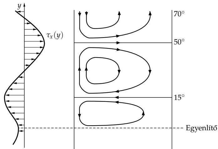
4.14. ábra. Az óceáni körök sematikus rendszere és a nyírás átlagos függése a szélességtől
