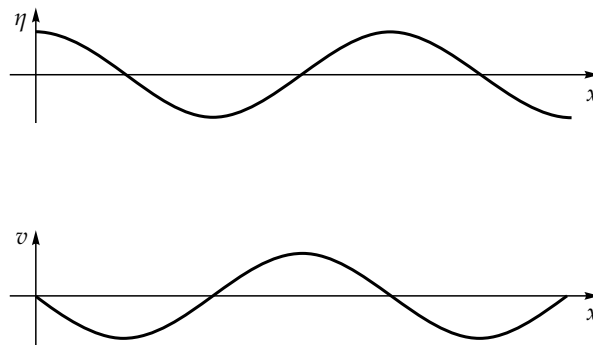
2.10. ábra. A felszíni alak és a v komponens egy x irányban terjedő szabad felszínű Rossby-hullámban. A zárt felszínű esetben \eta szerepét a p' dinamikai nyomás veszi át.
