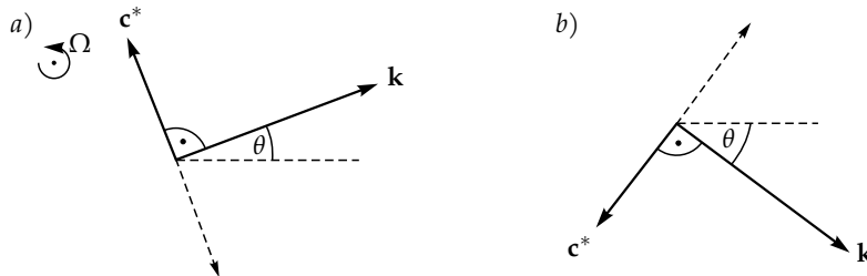
1.15. ábra. Tehetetlenségi hullámok \mathbf{c}^* csoportsebességének és \mathbf{k} hullámszámvektorának viszonya pozitív forgatási szögsebesség mellett. A szaggatott nyíl a negatív frekvenciához tartozó csoportsebesség.
