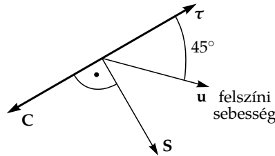
4.8. ábra. Az \mathbf{S} Ekman-transzport, a \boldsymbol{\tau} nyírási vektor és az \mathbf{u} felszíni áramlási sebesség egymáshoz viszonyított iránya az északi féltekén a felső határrétegben, egységnyi térfogatra vonatkoztatva. A \mathbf{C} vektor az Ekman-transzport által okozott sebességnövekményre ható Coriolis-erőt jelöli a teljes határrétegben, amely merőleges magára az Ekman-transzportra.
