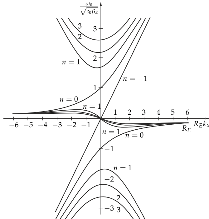
10.11. ábra. Az egyenlítői hullámok (10.90)-nel leírt diszperziós relációja az északi féltekén n = -1, 0, 1, 2, 3 -ra. A Poincaré- és Rossby-hullámokhoz az n = 1, 2, \dots indexek tartoznak. (A 2 és 3 indexű Rossby-hullám diszperziós görbéje mellé helyhiány miatt nem írtuk ki az indexet.) Az n = 0 módus a kevert hullám. A Kelvin-hullám az n = -1 választásnak felel meg.
