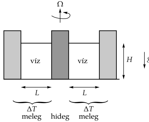
6.18. ábra. A baroklin instabilitás kimutatásának forgóhengeres kísérleti elrendezésének kereszt-metszete és a rendszer jellemző paraméterei
