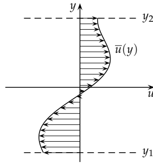
10.8. ábra. Általános kétdimenziós \bar{u}(y) áramlási profil, amelynek stabilitását vizsgáljuk kis perturbációkra kétdimenziós áramlásban.
