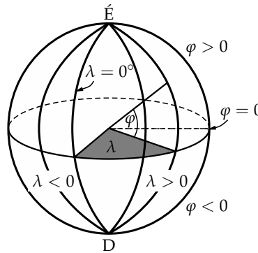
3.1. ábra. A földrajzi koordináták. \varphi a földrajzi szélességet, \lambda a földrajzi hosszúságot jelöli.
