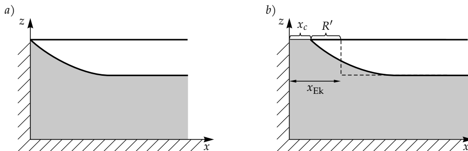
13.3. ábra. Part menti feláramlás fázisai hosszú idő óta egyenletesen fújó szél esetén. Az elválasztó felület a t_0 pillanatban eléri a felszínt a partvonal mentén (a), a frontvonal az x_c távolságig a t_c pillanatban jut el (b).
