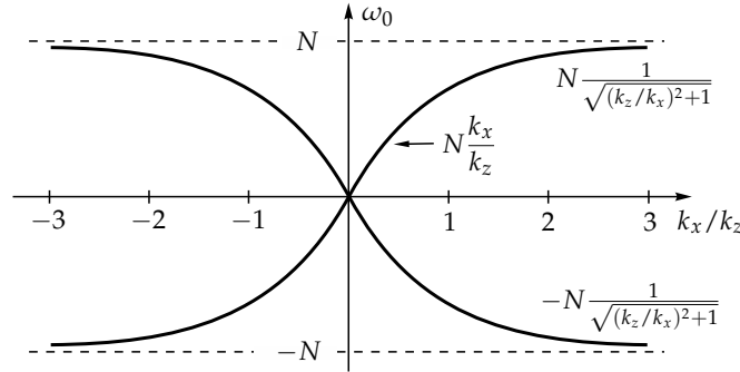
5.3. ábra. A belső hullámok \omega_0(k_x/k_z) diszperziós relációja ( k_y = 0 ). N -nél nagyobb frekvenciájú belső hullámok nem létezhetnek. A nyílhoz tartozó alak az origó környékén érvényes. A N \rightarrow 2\Omega , k_x \leftrightarrow k_z ( \cos \theta \rightarrow \sin \theta ) cserével a tehetetlenségi hullámok diszperziós relációját kapjuk (1.13. ábra).
