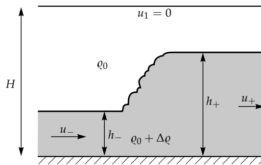
12.9. ábra. Stacionárius belső hidraulikus ugrás és jellemzői a redukált sekélyfolyadék-modellben. A vízlépcső helye nem változik, miközben az alsó közeg áramlik!
