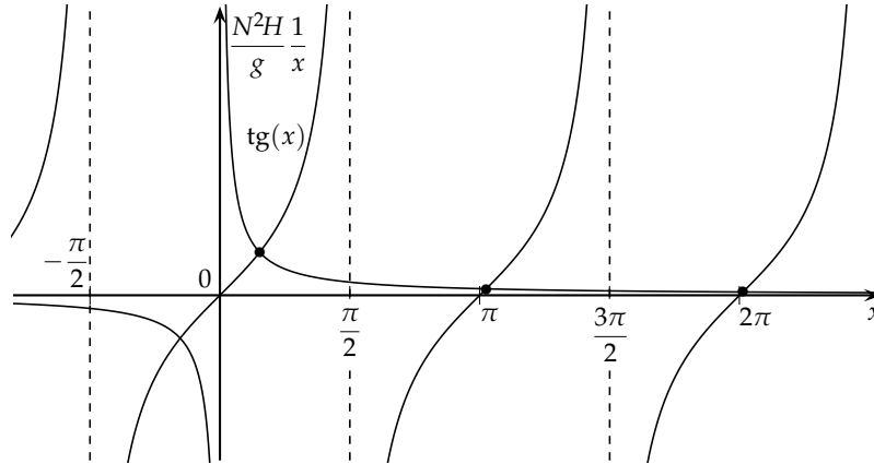
5.7. ábra. A szabad felszíni mozgáshoz tartozó normálmódusok sajátérték-problémájának grafikus alakja. A fekete metszéspontoknak megfelelő x_n = NH/c_n megoldások megadják a lehetséges sebességeket.
