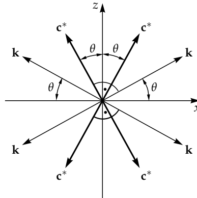
1.16. ábra. Pontszerű, |\omega| < 2|\Omega| frekvenciájú forrásból induló tehetetlenségi hullámok és csoportsebességeik lehetséges irányai. Hullámterjedés a \mathbf{k} vektorok irányába lehetséges, energiaterjedés viszont a rájuk merőleges \mathbf{c}^* irányokban történik.
