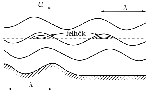
5.6. ábra. Hegy mögötti hullámok sematikus képe. Ha a középső levegőréteg nedves, és a hullámhegyek elérik a kicsapódási szintet (szaggatott vonal), akkor a hegyvonulattal párhuzamos felhősávok, vagy lencsefelhők alakulnak ki.
