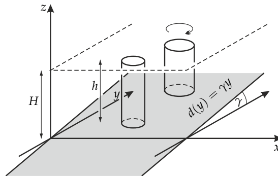
2.6. ábra. Topografikus Rossby-hullám kialakulásához szükséges döntött aljzat. A pozitív y irányba mozduló folyadékoszlop örvényessége csökken \Omega > 0 esetén.
