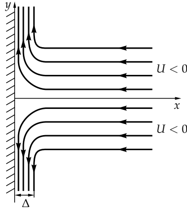
10.5. ábra. Nyugati óceáni partnak futó U sebességű ideális áramlás által keltett erős peremáramlat az északi féltekén
