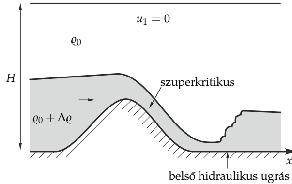
12.8. ábra. A meredek domborzati lejtőn lezúduló folyadék szuperkritikussá gyorsul, és a sík felszínre való kifutás után belső hidraulikus ugrás képződik.
