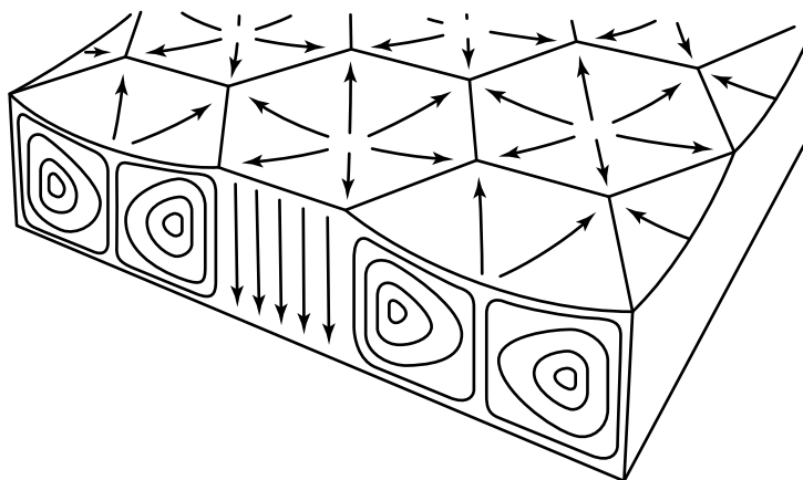
5.19. ábra. Stacionárius konvekciós áramlás. Közvetlenül a kritikus hőmérséklet-különbség (kritikus Rayleigh-szám) elérése után szabályos, hatszöges szerkezetű áramlási cellák is kialakulhatnak. A hatszög alapú hasáb szemközti oldalai közötti távolság \lambda_c .
