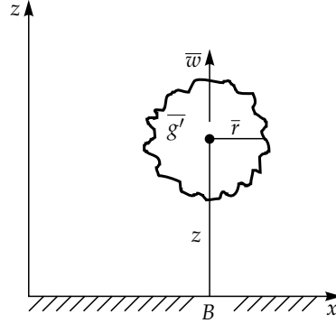
14.1. ábra. Az emelkedő termik legfontosabb átlagos paraméterei. Az emelkedési sebesség csökken, mert felszállás közben egyre több sűrű anyag kerül a termikbe turbulens besodródás révén.
