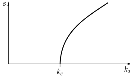
5.15. ábra. A k_x hullámszámú perturbáció s instabilitási rátájának sematikus rajza a Kelvin-Helmholtz-instabilitásban. A k_c kritikusnál kisebb hullámszámú perturbációk stabilak, ott az áramlást a sűrűségkülönbség stabilizálja.
