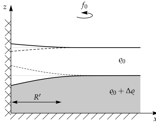
6.3. ábra. Belső Kelvin-hullám kétrétegű közegben. A hosszú szaggatott vonalak a felületek alakját jelzik a folytonos vonalnak megfelelőnél fél periódussal később. A hullám a -y irányban halad a belső hullámok c_1 sebességével, az x tengely mentén pedig lecseng az R' belső Rossby-sugárnak megfelelő távolságon.
