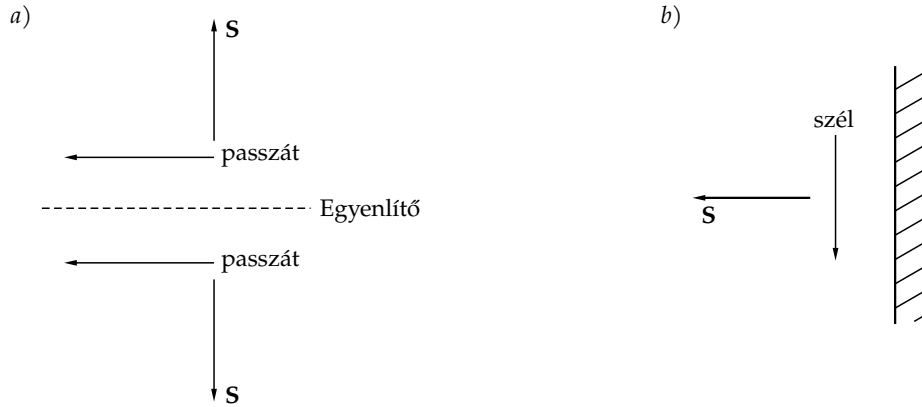
4.9. ábra. A szelek és az Ekman-transzport, vagyis a határrétegbeli átlagos sebesség irányának viszonya. a) Egyenlítői övezet, b) Észak–déli futású partvonalak az északi féltekén
