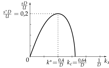
10.10. ábra. A 10.9. ábra alapáramlásának s instabilitási rátája.
