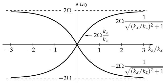
1.13. ábra. Az (x, z) síkban terjedő ( k_y = 0 ) tehetetlenségi hullámok \omega_0(k_z/k_x) diszperziós relációja. |2\Omega| -nél nagyobb frekvenciájú hullámok nem létezhetnek. A nyílhoz tartozó alak csak az origó környékén érvényes.
