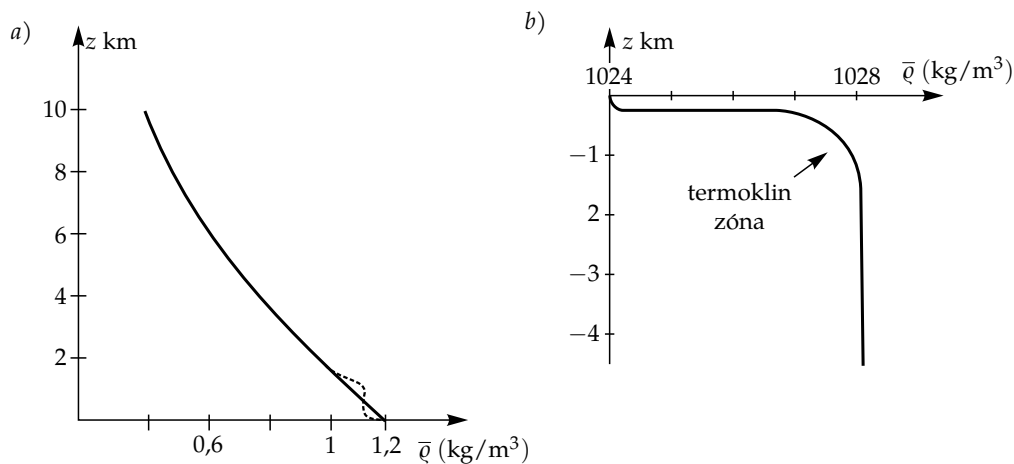
5.1. ábra. Az alsó légkör, a troposféra (a) és az óceánok (b) tipikus átlagos sűrűségeloszlása. A légkör alsó határrétege időnként jól kevertté válik. Ebben a planetáris határrétegben a sűrűség közel állandó (pontosított vonal). Jól kevert közeg az óceánok felső határrétegének ún. keveredési rétege is. Alatta gyors sűrűségnövekedés következik be az ún. termoklin zónában, majd a sűrűség közel állandóvá válik.
