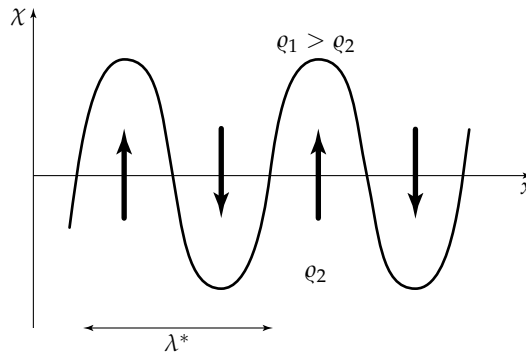
12.15. ábra. Sematikus ábra a Rayleigh–Taylor-instabilitás kezdeti jellegéről. Az idő múlásával az ujjak szabálytalanná válnak, és turbulens keveredés alakul ki. A végeredmény az, hogy a nehéz folyadék kerül alulra.
