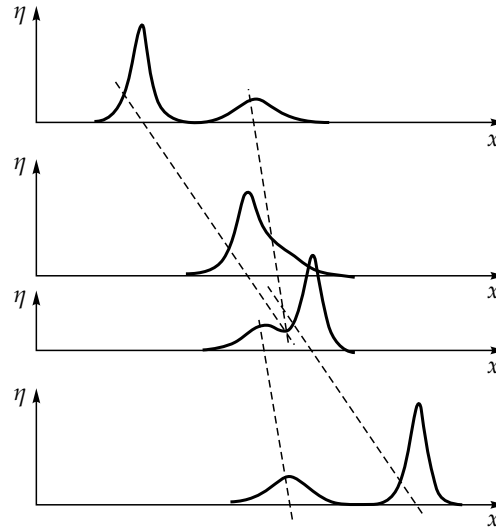
9.2. ábra. Két szoliton kölcsönhatása. Mindkét szoliton jobbra halad az x tengely mentén, ezért a nagyobb utoléri a kisebbet, és kétszoliton-állapotba kerülnek. Ennek felbomlása után elegendő hosszú idővel eredeti alakjuk és sebességük helyreáll. Az egymás alatti ábrák egyre későbbi időpontoknak felelnek meg. A szaggatott vonalak a kezdeti és végállapot sebességének megfelelő elmozdulást mutatják. Az ütközés pillanatában ezek nem esnek egybe, amely mutatja, hogy fáziseltolódás történt.
