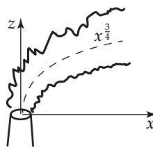
14.3. ábra. A turbulens csóva tipikus alakja állandó erősségű szélben x^{3/4} alakú fekvő parabola, amely gyakran megfigyelhető a kéményekből kiáramló füst formájában. Erősebb szélben a parabola laposabb.
