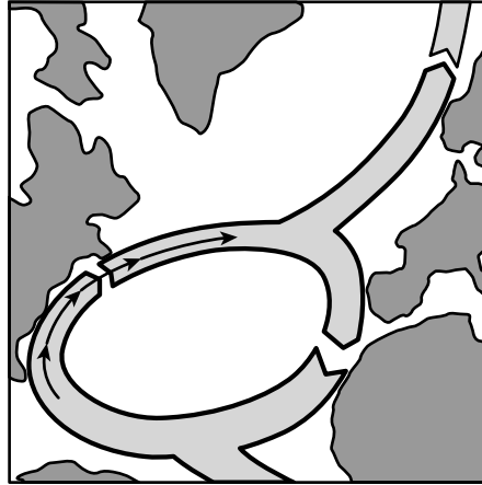
3.9. ábra. Az Észak-atlanti kör sematikus ábrája. Ez, mint az össze többi nagy kör is, óceáni anti-ciklon. A vékony nyílazott vonal a kör Golf-áramlatnak nevezett szakaszára utal.
