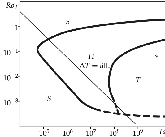
6.19. ábra. Forgóhengeres mérések eredményének sematikus áttekintése a Ta Taylor-szám és az Ro_T termikus Rossby-szám logaritmussai által definiált paramétersíkon. (A vonalak szaggatottsága a kísérleti eredmények bizonytalanságára utal.) Az S-sel jelölt tartományban a termikus áramlás stabil és forgásszimmetrikus. A H tartományban a termikus áramlás instabillá vált, de nagy amplitúdójú baroklin hullámok stabilizálódnak. A T jelű tartományban az áramlás szabálytalan, a geosztrófikus turbulencia jegyeit mutatja. A szövegben említett laboratóriumi adatpár a csillaggal jelölt pontnak felel meg.
