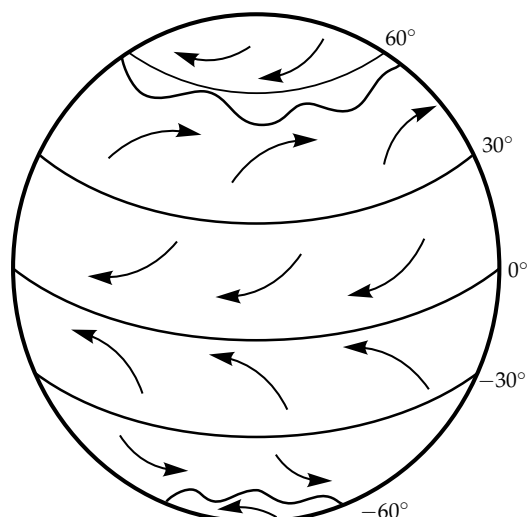
3.12. ábra. A Föld felszínén uralkodó zonális szelek sematikus rajza
