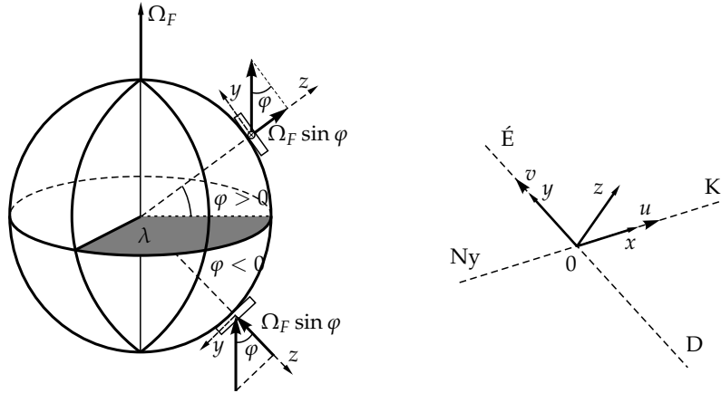
3.2. ábra. A forgási szögsebességvektor komponensei a két féltéken (bal oldali rajz), a Földet gömbként közelítve. A lokális rendszer (jobb oldali rajz), amelyben a z irány a helyi függőleges.
