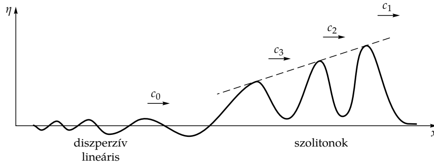
9.3. ábra. Általános kezdeti kidudorodásból kialakuló jobbra haladó hullámvonulat elegendően hosszú idő eltelte után (a függőleges skála torzított). A sort a legnagyobb szoliton vezeti, a többiek (mind más magasságú) nagyságrendben követik, és a kis amplitúdójú hullámvonulat zárja. Ez egyre jobban szétfolyik, és lemarad a szolitonoktól. Az utóbbiak burkolója (szaggatott vonal) mindig egyenes.
