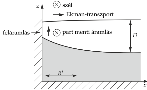
13.2. ábra. Part menti feláramlás a parttal párhuzamosan fújó szél esetén az északi féltekén. A redukált sekélyfolyadék-egyenlet szellemében az alsó réteg olyan vastag, hogy abban az áramlás sebessége elhanyagolható.
