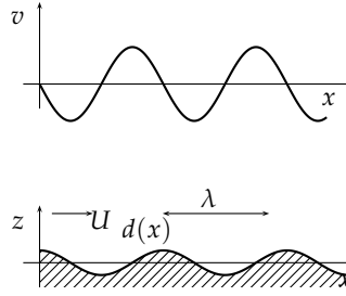
3.14. ábra. Zonális áramlás és periodikus domborzat kapcsolata kvázi-geosztrofikus közelítésben. Az áramlás a hegységrendszer (alsó kép) felett stacionárius Rossby-hullámot kelt a vízszintes síkban. A felső kép a v sebesség helyfüggését mutatja a k > k_c ( \lambda < \lambda_c ) esetben.
