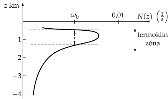
12.4. ábra. A Brunt–Väisälä-frekvencia tipikus mélységfüggése tengerekben. A legnagyobb frekvenciák a termoklin zónába esnek. Adott \omega_0 frekvenciájú, viszonylag gyors belső hullámok csak a termoklin zóna azon alrétegében alakulhatnak ki, ahol |\omega_0| \leq N(z) (szaggatott vonallal jelölt sáv).
