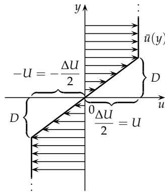
10.9. ábra. Véges vastagságú nyírási réteg két ellenkező irányba mozgó folyadéktömbbe ágyazva, amelyek között a sebességkülönbség \Delta U
