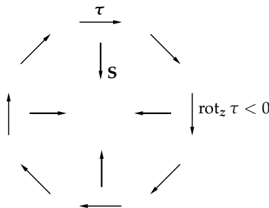
4.10. ábra. Anticiklonális nyíráseloszlás és az Ekman-transzport az északi féltekén
