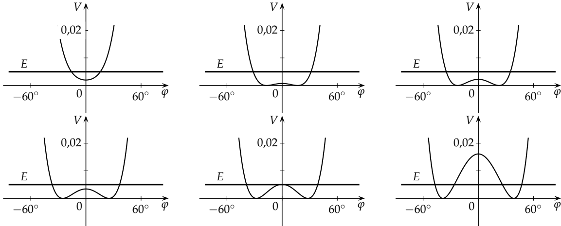
3.4. ábra. A V(\varphi) potenciál alakjának változása csökkenő N értékekre, N > 1 -től kezdve. A választott értékek az előző ábra \varphi_0 -jaihoz tartozó N(\varphi_0) impulzusnyomatékok, ugyanabban a sorrendben. A kritikus eset annak felel meg, hogy az origóhoz tartozó maximum eléri a E = u_0^2/2 értéket.
