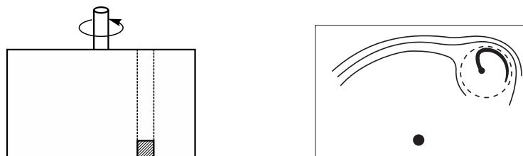
1.8. ábra. a) A Taylor-kísérlet oldalnézeti képe: forgatott edény aljára kis korongot helyezünk. A pontozott vonal a korong felett elhelyezkedő folyadékoszlopot jelöli. b) Az együtt forgó rendszerben felülről megfigyelt áramlás sematikus rajza: a lassan mozgó festékcsíkok kívülről megkerülik a korong alapú hengert (szaggatott vonal). A henger belsejéből induló csepp a henger belsejében marad. A fekete pont a forgástengely.
