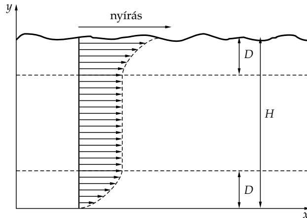
4.1. ábra. A forgatott folyadékbeli alsó és felső Ekman-réteg és a bennük kialakuló sebességeloszlás sematikus képe. A felszínen nyíróerő hat, és a folyadék belsejében áramlás van jelen. D az Ekman-réteg vastagsága.
