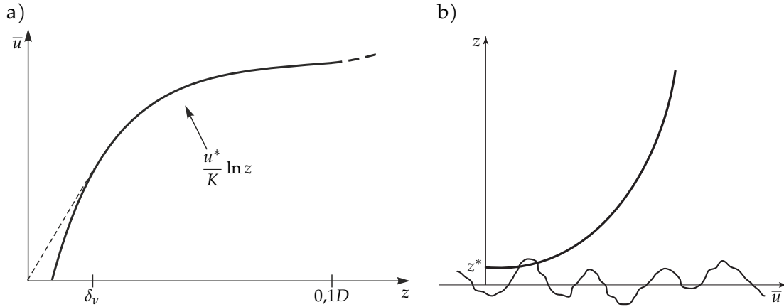
7.2. ábra. a) A logaritmikus sebességprofil sima felület esetén: a vízszintes átlagsebesség \bar{u}(z) nagyságának magassághoz tartozó függése a turbulens határrétegben. A \delta_v vastagságú viszkózus alrétegben a logaritmikus függés lineárisba vált át (szaggatott vonal). A fal menti rétegben kívül az univerzális logaritmikus alak érvényét veszti, amit a hosszú szaggatott görbe jelez. b) Durva felület (szabálytalan görbe) esetén viszkózus alréteg nem alakulhat ki. z^* az a magasság, ahol a tipikus sebesség eltűnik, értéke a felület érdességét jellemzi. A profil (7.32) alakú, itt a z(\bar{u}) függvényt ábrázoljuk.
