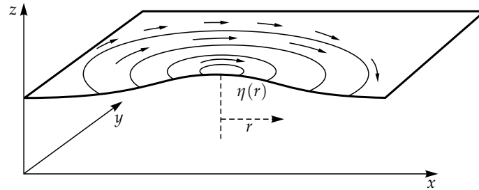
2.5. ábra. A forgásszimmetrikus \eta(r) , r -rel csökkenő felszíni alak g/(2\Omega)|d\eta(r)/dr| nagyságú, negatív körüljárású, anticiklonális geosztrofikus áramlást tart fenn \Omega > 0 esetén. A behorpadó felülethez ugyanekkor ciklonális áramlás tartozik.
