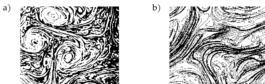
7.5. ábra. Kétdimenziós turbulencia jellegzetes tartományai. a) Nagy örvények b) Az örvények közötti szálas, nyírási mintázat (P. Tabeling (2002) alapján)
