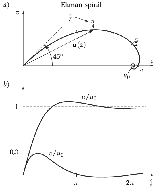
4.3. ábra. Áramlás az alsó Ekman-rétegben az északi féltekén a folyadék belsejében uralkodó u_g = u_0, v_g = 0 geosztrofikus áramlás mellett, a (4.26) összefüggés alapján. a) A különböző magasságokban kialakuló \mathbf{u} sebességvektorok. A spirál mellé írt számok a \delta egységekben mért z magasságot mutatják. A z/\delta = \pi magasságban tűnik el felfelé haladva először a v komponens. b) Az u és v sebességkomponensek magassághatárolásának függése. A határrétegbeli sebesség a z = D = \pi\delta szinten (a határréteg peremén) jó közelítéssel megegyezik a folyadék belsejében jelenlevő geosztrofikus sebességgel.
