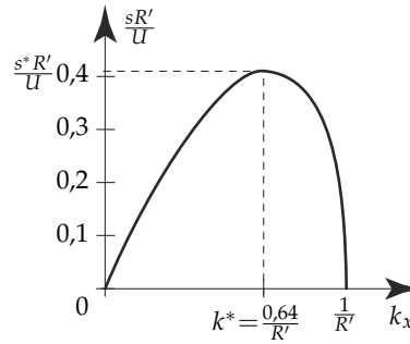
6.17. ábra. A baroklin instabilitás s instabilitási rátája kétrétegű közegben f -sík-közelítésben. Az instabilitási tartomány és a leggyorsabban növekvő hullám k^* hullámszáma nem függ a termikus áramlás sebességétől.
