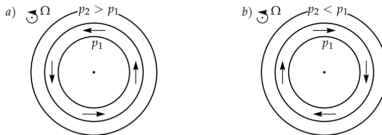
1.10. ábra. Forgásszimmetrikus nyomáseloszlás hatására kialakuló geosztrofikus áramlás alacsony (a) és magas (b) nyomású központ körül \Omega > 0 esetén. Nyomásminimum körül (a) ábra) az áramlás ciklonális, a maximum körül (b ábra) anticiklonális. Negatív forgásirányhoz negatív ciklonális örvénylés tartozik.
