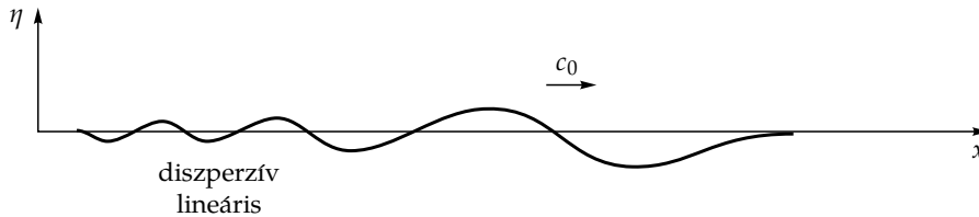
9.4. ábra. Általános kezdeti behorpadásból kialakuló hullámvonulat. Szolitonot nem tartalmazhat, csak kis amplitúdójú, szétfolyó hullámok jelennek meg, amelyek közül csak a leghosszabb terjed c_0 sebességgel.
