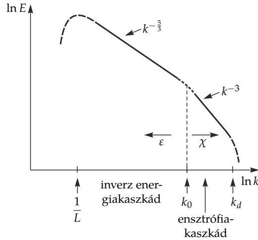
7.7. ábra. A kétdimenziós turbulencia energiaspektruma. k_0 és k_d \sim (\chi/\nu^3)^{1/6} az energiabetáplálási, illetve a disszipációs hullámszám. Az energiakaskád k^{-5/3} hatványviselkedése az 1/L < k < k_0 , az enztrófiakaskádot jellemző k^{-3} alak pedig a k_0 < k < k_d tehetetlenségi tartományban érvényes.
