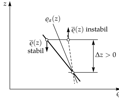
12.19. ábra. A \bar{\rho}(z) sűrűségprofil stabilitásának feltétele összenyomható közegben: a sűrűségnek felfelé haladva az adiabatikus profilnál (vékony vonal) gyorsabban kell csökkennie (vastag vonal). A szaggatott vonal instabil rétegzettséghez tartozik.
