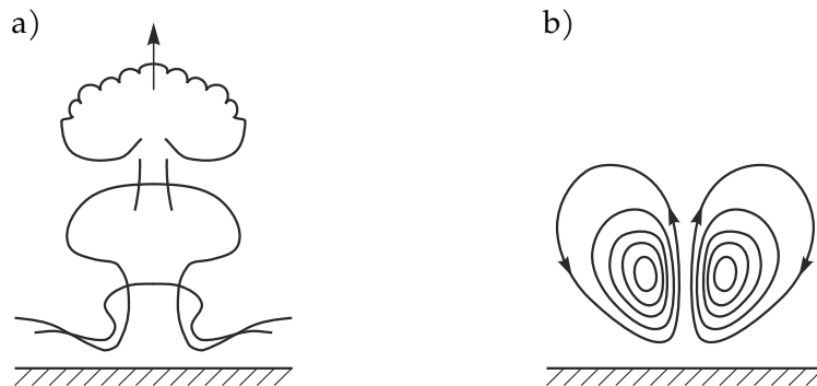
5.22. ábra. Termik szerkezete. a) A felszállás három fázisa (a vonal a hideg–meleg határfelületet mutatja). b) Áramvonalak az (x, z) síkmetszeten, adott pillanatban
