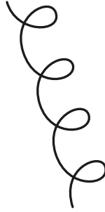
3.6. ábra. Tengeri folyadéktömeg mozgása sematikus ábrázolásban a néhányszor 10 km-es skálán közel állandó nyomás esetén, amikor a mozgás egy lassú északnyugatra irányuló áramlás és a tehetetlenségi körmozgás eredője. Közepes szélességeken (3.28)-nak megfelelően egy teljes hurok bejárás ideje kb. 0,7 nap.
