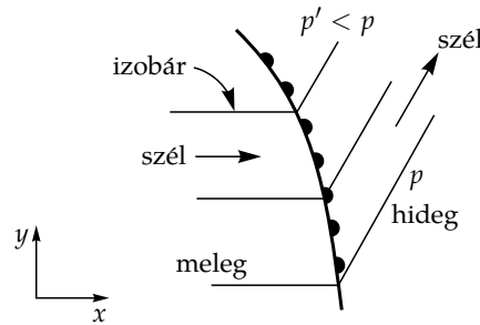
6.8. ábra. Felszíni nyomáseloszlás légköri front mentén az északi féltekén. A felszíni sebesség-ugrás következtében az izobárok megtörnek . Az ábra egy nyugatról érkező melegfront (vonal kis félkörökkel) körüli közel geostrofikus viszonyokat mutató sematikus rajz.
