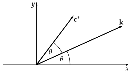
2.8. ábra. A zárt felszínű Rossby-hullámok \mathbf{c}^* csoportsebességének iránya a \mathbf{k} hullámszámvektorhoz képest
