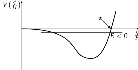
9.11. ábra. A cnoidális hullámhoz rendelhető potenciálmozgás képe, ahol V(x) = 3(-\alpha x^2 + x^3)/2 . Az ilyen hullámokban E < 0 .
