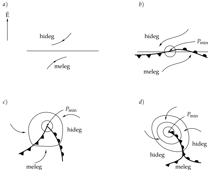
6.15. ábra. A mérsékelt övi ciklonok kialakulásának sematikus rajza az északi féltekén, felszíni viszonyok. (a) Kiindulási állapot: a poláris front (egyenes vonal) nem mozog. (b) Kis perturbáció: a meleg feláramlás miatt létrejövő ciklonális mozgás a nyugati oldalon mozgó hidegfrontot (kis háromszögekkel jelölt görbe), a keletin pedig mozgó melegfrontot (kis félkörökkel jelölt görbe) hoz létre. (c) A közép stádium: a frontvonalak begömbülnek, a hidegfront kezdi utolérni a meleget (a ciklon középpontja a termikus szél miatt kelet felé mozog). (d) A végállapot (okklúziós fronttal): a meleg levegő az alacsony nyomású központ körül mindenütt a felső légrétegekbe szorult, az instabilitás hajtóereje megszűnt.
