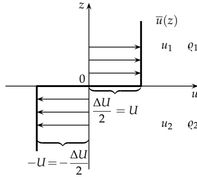
5.14. ábra. Az \bar{u}(z) alapáramlás sebességprofilja (vastag vonal). Az elválasztó felület kezdeti alakja a z = 0 sík, \chi = 0 . Az 1 és 2 indexek a felső, illetve alsó közegre vonatkoznak.
