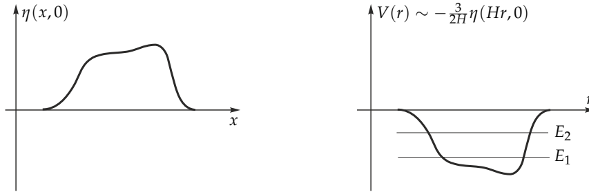
9.5. ábra. A H vízmélységhez tartozó kezdeti felszíni alak (bal oldal) és a kvantummechanikai sajátérték-probléma (jobb oldal) kapcsolata. A kezdeti felszínelak ellentettjével arányos potenciálgödör kötött állapotainak sajátenergiái határozzák meg a szolitonok számát és adatait a (9.20)–(9.23) összefüggések szerint.
