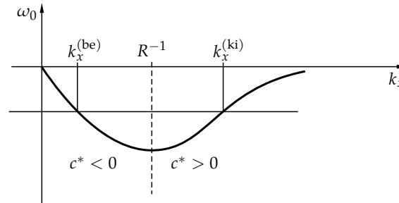
3.11. ábra. Planetáris hullámok diszperziós relációjából leolvasható, hogy észak–déli partvonallal ütközve a beeső és visszavert hullám csoportsebessége csak úgy lehet ellenkező előjelű, ha a bejövő és kimenő hullámszámok az R^{-1} Rossby-hullámszámot közrefogják.
