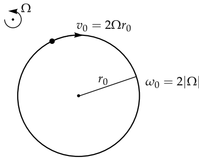
1.2. ábra. Tehetetlenségi körmozgás a forgatott rendszer bármely pontja körül kialakulhat, ha a mozgó testre csak a Coriolis-erő hat. A körbefordulás iránya pozitív \Omega esetén negatív.
