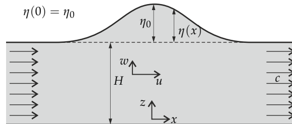
9.9. ábra. Balra, c sebességgel haladó szoliton és áramlása a vele együtt mozgó koordináta-rendszerből nézve
