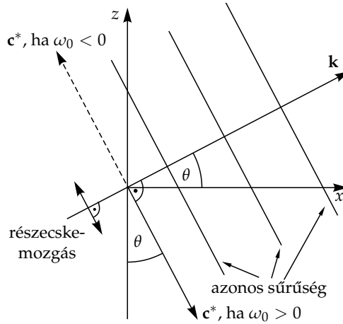
5.4. ábra. A c^* csoportsebesség és k hullámszámvektor viszonya belső hullámban. Az energia mindig k -ra merőlegesen terjed. Az, hogy jobbra vagy balra, a frekvencia előjelétől függ. A részecske-mozgás a hullámszámvektorra merőleges síkban történik.
