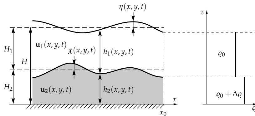
5.9. ábra. A kétrétegű közelítésben két élesen elkülönülő, homogén és összenyomhatatlan sekély folyadékréteggel modellezzük a közeget. A belső és a külső felszín is szabadon mozoghat. A vízszintes sebesség mindkét rétegben független a magasságtól.
