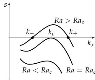
5.17. ábra. A s mennyiség sematikus függése a k_x hullámszámtól különböző Ra Rayleigh-számok esetén
