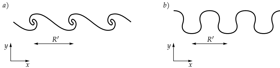
6.14. ábra. A baroklin instabilitás következtében megjelenő nagy amplitúdójú baroklin hullámok sematikus alakjai (felülnézet) a több belső Rossby-sugárnyi skálán. (a) Begyűrődő hullámok (a Kelvin–Helmholtz-hullámokhoz hasonló szerkezet). (b) Meanderező áramlás
