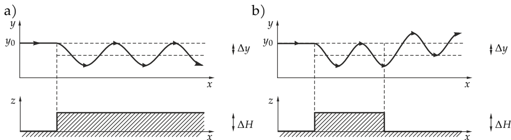
10.3. ábra. A domborzat hatása nyugatról érkező áramlásokra. A rajzok alján a domborzat, felül az áramlás felülnézeti képe látható. a) Lépcső. b) Véges domborzati elem. Ha a domborzat periodikusan ismétlődik, a domborzat hullámhossza is hatással van a kialakuló hullámzásra (3.10. fejezet).
