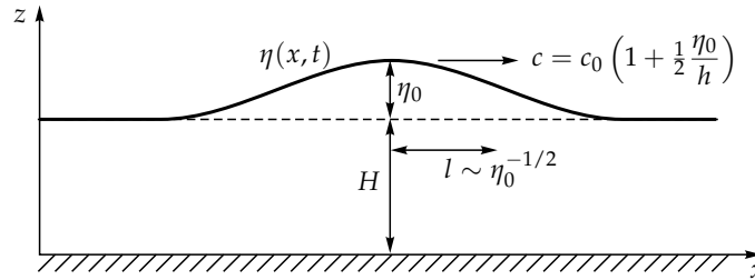
2.16. ábra. Szolitonok jellemző alakja és paraméterei. A szoliton nem szinuszhullám, a felületváltozás mindenütt kiemelkedés, \eta sehol nem vált előjelet.
