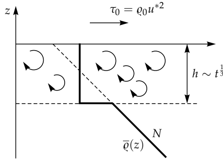
14.4. ábra. Az óceáni keveredési réteg h vastagsága a szélnyírás hatására nő, mert a turbulens örvények által okozott besodródás révén egyre mélyebb szintekig homogenizálódik a közeg. A szaggatott vonal arra utal, hogy kezdetben az egész folyadék egyenletesen rétegzett. Később az N Brunt–Väisälä-frekvencia csak a határrétegen kívüli tartományt jellemzi.
