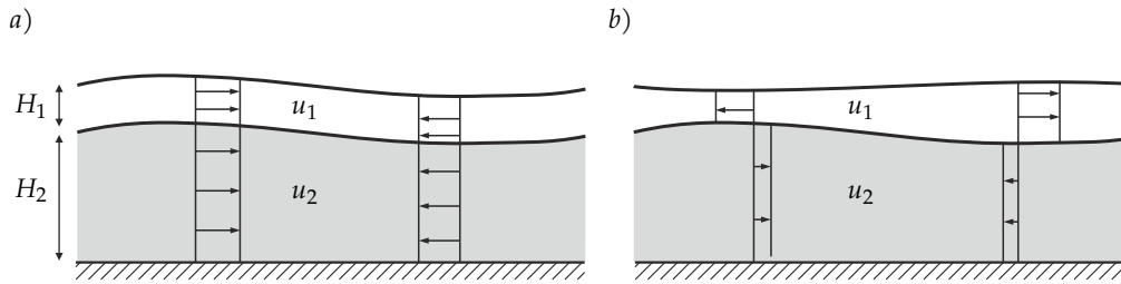
5.10. ábra. Kis amplitudójú lineáris hullámok kétrétegű folyadékban. a) Barotróp módus: mindkét réteg hasonlóan mozog. b) Baroklin módus: mindkét réteg ellentétes irányban áramlik, és az elválasztó felület hullámzása sokkal erősebb a felszínénél.
