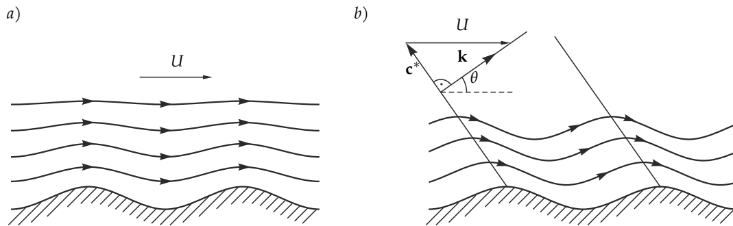
5.5. ábra. Periodikus domborzat háttéráramlásban stacionárius sebességteret alakíthat ki. A kritikus sebességnél gyorsabb áramlás esetén a mozgás erőssége a magassággal csökken (a). Ennél lassabb áramlásban csillapítatlan belső hullámok keletkeznek, amelyek az áramlás irányában és felfelé terjednek (b). A relatív mozgás csoportsebessége merőleges a terjedési irányra ( \tan(\theta) = k_z/k_x ), de a háttéráramlás sebességével képzett eredő párhuzamos vele, ahogy a felső betétraajz mutatja. A hegységrendszerek fölött kialakuló Rossby-hullámokkal (3.14. ábra) szemben a hullámzás itt a függőleges síkban történik, és bármilyen előjelű háttéráramlásban kialakulhat.
