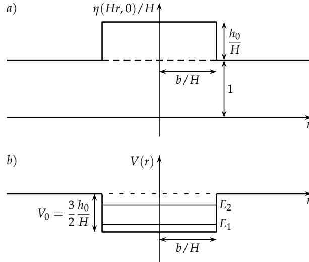
9.7. ábra. A kezdeti derékszögű felszíni kiemelkedés dimenziótlal alakja (a) és az azzal kapcsolatos kvantummechanikai probléma dimenziótlal potenciálgödre (b)
