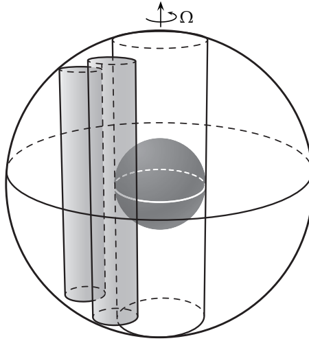
8.1. ábra. A külső magban zajló áramlás két Taylor-oszlop berajzolásával illusztrált sematikus képe. A fekete gömb a belső magot jelzi, körülötte az érintő henger, a külső gömb a mag és a köpeny elválasztó felülete.
