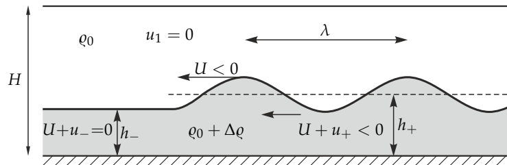
12.10. ábra. A belső torlókullám mozgó hidraulikus ugrás. Az ábra álló koordináta-rendszerben mutat hullámzó (unduláris) belső torlókullámot. Az alsó közeg, amelybe a vízlépcső behatol, nyugalomban van, a vízlépcső alatt a közeg balra áramlik U + u_+ < 0 sebességgel (a sebességek különbsége az energiavesztés következménye). A szaggatott vonal a nem hullámzó bore magasságára utal.
