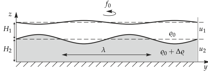
6.2. ábra. Belső (baroklin) Poincaré- (tehetetlenségi gravitáció-) hullám kétrétegű közegben. A mozgás a tehetetlenségi körmozgás és a g' redukált gravitációs térben kialakuló belső hullámzás kombinációja. A külső felszín változásánál jóval erősebb a belső felszíné.
