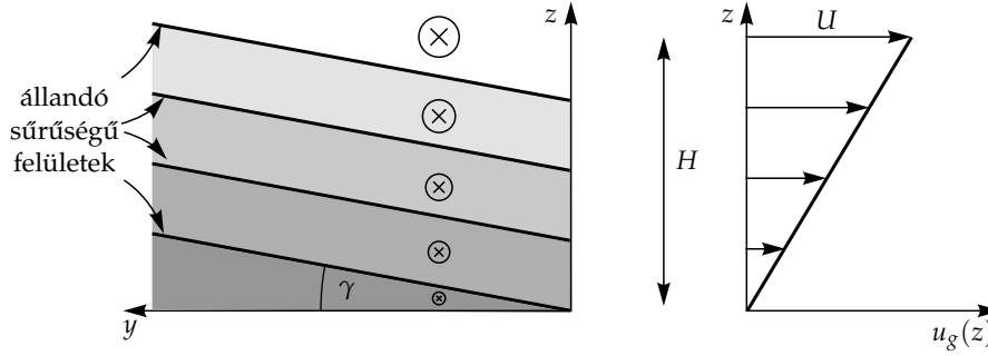
6.11. ábra. A termikus áramlás a ferdén elhelyezkedő sűrűségfelületekhez tartozó geosztrofikus áramlás. Ha az emelkedés a pólus irányában történik, függőlegesen felfelé haladva egyre erősebb keletre mutató áramlást (nyugati szelet) tapasztalunk.
