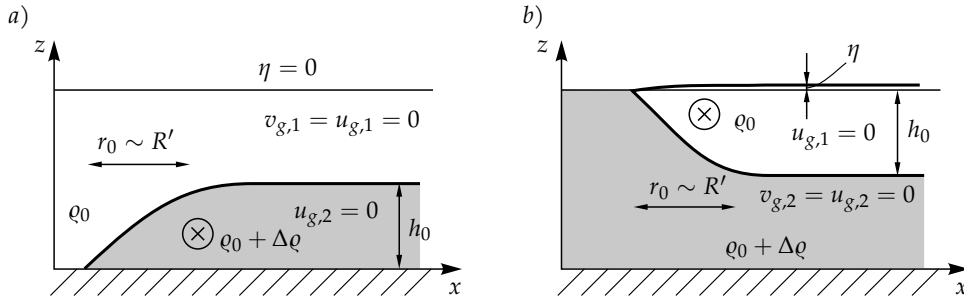
6.9. ábra. Az r_0 távolságon exponenciálisan lecsengő függvénnyel leírt frontok geosztrofikus egyensúlyban az északi féltekén. (a) Hidegfront (levegő vagy folyadék) az aljzaton. (b) Melegfront a folyadék felszíne alatt. Ez egyben a Golf-áramlat modelljének tekinthető, annak az amerikai partvonallal párhuzamosan futó szakaszában. A pólus felé irányuló áramlás a front melletti r_0 vastagságú tartományban jelentős.
