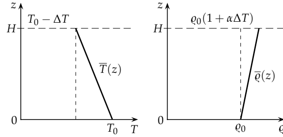
5.16. ábra. Az alapállapotú hőmérséklet- és sűrűségprofil, amely áramlással nem társul. Ez az állapot válik instabillá az Ra_c kritikus Rayleigh-számnál, ahol beindul az áramlás.
