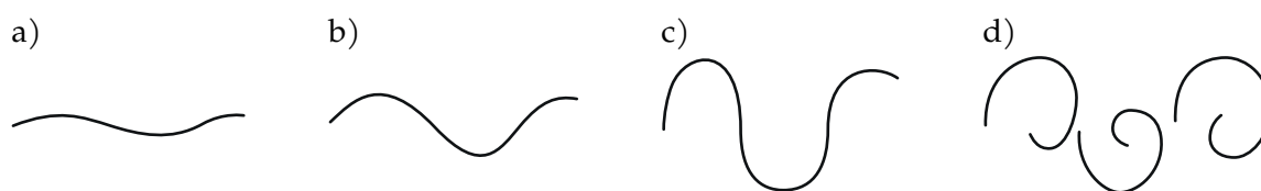
6.20. ábra. A baroklin instabilitás következtében kifejlődő tipikus szennyeződési (festéktörjedési) mintázat a forgóhengeres kísérlet turbulens tartományában. Az a)–d) rajzok egy megfestett folyadékvonal alakjának időbeli változását mutatják sematikusan. Az a), b) fázisok az instabilitás kezdetére utalnak, a c) állapot nagy amplitúdójú, instabillá váló hullámra, a d) pedig hullámtörésre, amely szabálytalan ciklonális, anticiklonális örvényszerű rajzolatok kialakulására vezet.
