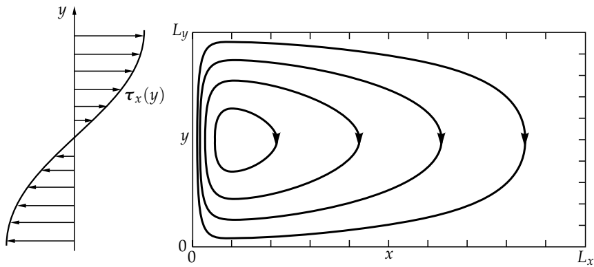
11.3. ábra. A Stommel-modell áramlási képe a 4.13. ábrához is használt nyíráseloszlással
