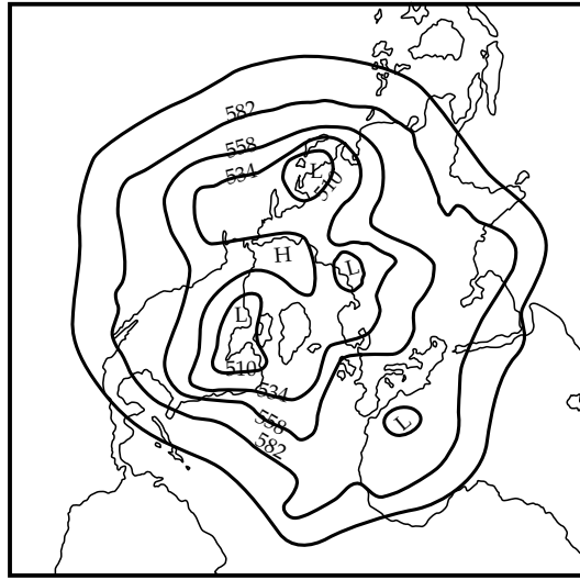
3.10. ábra. Planetáris hullám tipikus rajzolata szintvonalakban közepes magasságokban. A hullám jelenléte a sarkot körülölelő szintvonalak jelenlétében és azok meanderező jellegében mutatkozik meg.
