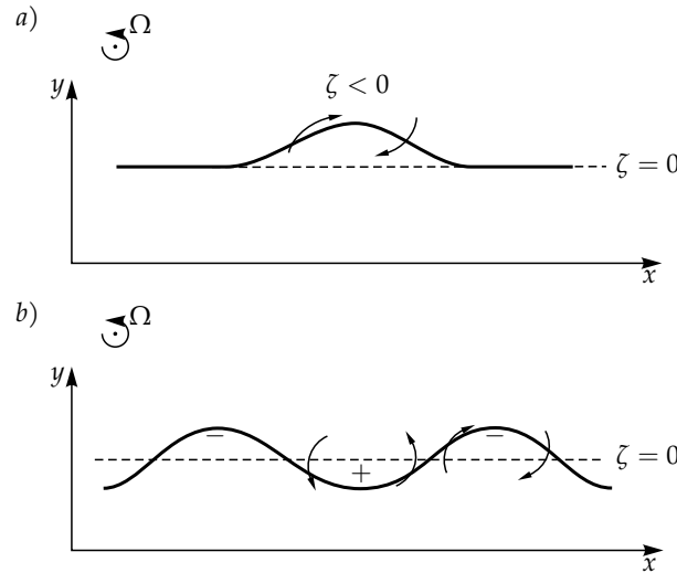
2.7. ábra. A Rossby-hullámok kialakulási mechanizmusa az (x, y) síkban pozitív forgatási irány esetén, y irányban emelkedő aljzat felett. a) Az eredetileg x irányú, zérus örvényességű folyadékvonalon kialakított kis y irányú kitüremkedés a potenciális örvényesség megmaradása következtében negatív köráramlást hoz létre, amely a púpot balra tolja. b) Egy hullámalak felváltva hoz létre negatív és pozitív örvényességet a hullám maximális, illetve minimális kitérésének megfelelően, és mindkét hatás a negatív x irányba történő elmozduláshoz vezet.
