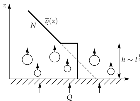
14.5. ábra. A földfelszín gyors nappali felmelegedése következtében a planetáris határréteg alulról fűtött közegnek tekinthető, amelyben a konvekció dominál. A felszálló termikek hatására egyre magasabb szintekig homogenizálódik az eredetileg közel egyenletesen rétegzett közeg. A planetáris határréteg h vastagsága ezért nő időben.
