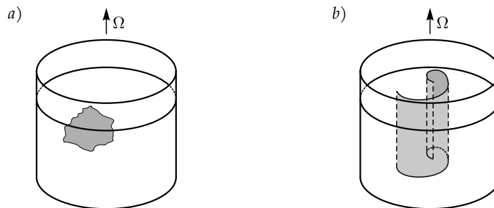
1.7. ábra. A Taylor–Proudman-tétel kísérleti megnyilvánulása. a) Gyorsan forgatott edénybeli folyadékba felülről festéket juttatunk. b) Függőleges festékfüggönyök alakulnak ki.
