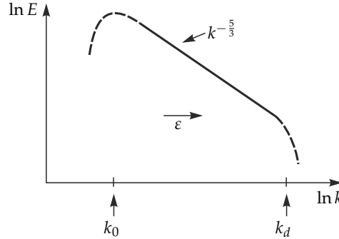
7.4. ábra. A háromdimenziós turbulencia energiaspektruma. k_0 és k_d \sim (\varepsilon/\nu^3)^{1/4} az energiabetáplálási és a disszipációs hullámszám. A k^{-5/3} hatványviselkedés a k_0 < k < k_d tehetetlenségi tartományban érvényes.
