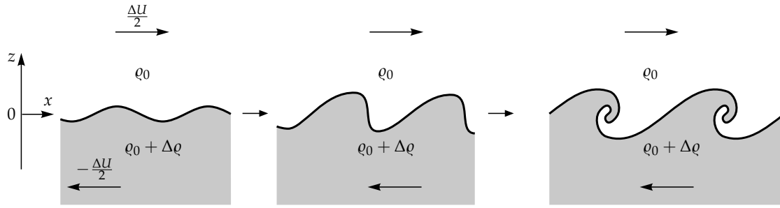
5.13. ábra. A két folyadékot elválasztó felület időfejlődése a relatív sebességkülönbség hatására kialakuló Kelvin–Helmholtz-instabilitás következtében. A megfigyelt átmeneti mintázat periodicitása a \lambda_c kritikus hullámhossz nagyságrendjébe esik. A valódi hullámtörés is a KH-instabilitás mechanizmusa szerint zajlik, csak ott a levegő és a víz közötti sűrűségkülönbség nem kicsi. A végállapot mindig turbulens áramlás.
