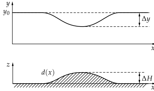
10.1. ábra. Domborzati kidudorodás (alsó ábra) hatása zonális áramlások vízszintes síkbeli pályájára helyfüggő Coriolis-paraméter esetén (felső ábra) geosztrofikus közelítésben az északi féltekén. A pálya független attól, hogy az áramlás keletről vagy nyugatról érkezik.
