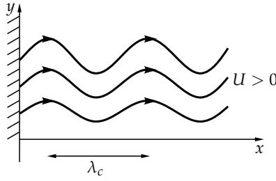
10.6. ábra. Az óceán nyugati partvonalától U átlagsebességgel eltartó áramlás az északi féltekén. A hullámhossz \lambda_c = 2\pi\sqrt{U/\beta} .
