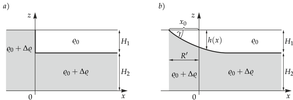
6.10. ábra. A geosztrofikus egyensúly beállása kezdetben függőleges elválasztó felület esetén. (a) A meleg közeg a pozitív félegyenes mentén állandó H_1 vastagságú rétegből indul. (b) A végálapotot exponenciális függvény írja le, amely az R' belső Rossby-sugáron cseng le az eredeti H_1 mélységig. A front is éppen R' távolságot mozdul el. A geosztrofikus egyensúlyi front meredeksége |\gamma| \approx H_1/R' .
