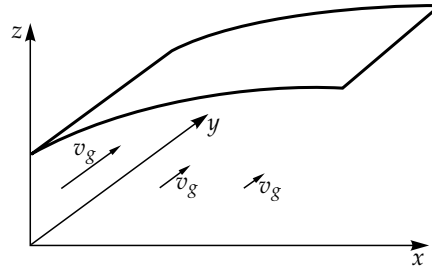
2.4. ábra. Az x irányban növekvő \eta(x) felszíni alak következtében kialakuló v_g = (g/2\Omega)d\eta(x)/dx nagyságú, pozitív y irányú geosztrofikus áramlás \Omega > 0 esetén
