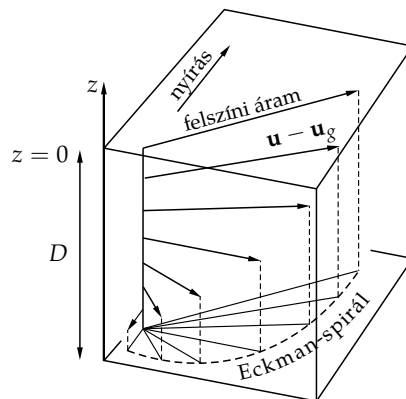
4.6. ábra. A felső Ekman-réteg az északi féltekén: a határrétegbeli sebességeltérés vektorának sematikus magasságfüggése
