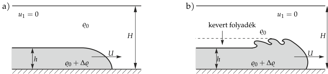
12.11. ábra. Gravitációs áramlat sematikus képe. a) Keveredésmentes, ideális eset keskeny sűrű réteggel. b) A Kelvin–Helmholtz-instabilitás (5.13. fejezet) fej kialakulására vezet, amely mögött jól kevert folyadékréteg marad vissza. A fej előredudorodása a viszkozitás következménye.
