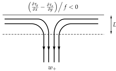
4.11. ábra. A felső határrétegben történő Ekman-pumpálás a határrétegből a folyadék belsejébe irányuló függőleges áramlás, amelynek erőssége a szélnyírás rotációjával arányos. w_+ ennek az áramlásnak a sebessége a felső határréteg alsó peremén. Leáramláshoz anticiklonális szélnyírás (az északi féltekén \text{rot}_z \tau < 0 ) tartozik, feláramláshoz ciklonális szélnyírás (az északi féltekén \text{rot}_z \tau > 0 ).
