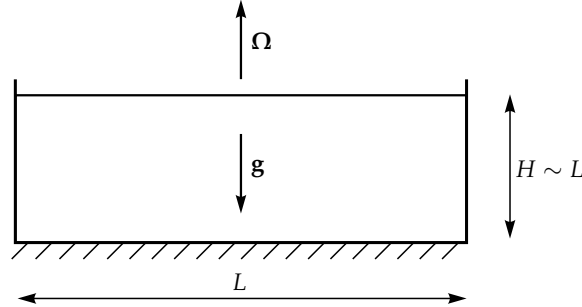
1.6. ábra. Folyadék függőleges tengely körül forgatott edényben. A H átlagos mélység összemérhető a L szélességgel. Ez utóbbi tekinthető egyben az áramlás jellemző vízszintes méretének. Az elrendezés a Föld sarkvidékei környékén vagy a laboratóriumban megvalósuló esetnek felel meg, hiszen \mathbf{g} a forgástengely irányába esik.
