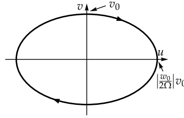
2.13. ábra. A sebességvektor mozgása tehetetlenségi gravitációhullámban ellipszispálya mentén történik, amely a hullám haladási irányában (jelen esetben az x tengely) nyújtott. A körüljárási anticiklonális.
