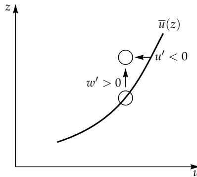
7.1. ábra. A sebességfluktuációk korrelációja negatív a határrétegben. Az \bar{u}(z) átlagos sebességprofil mellett az x irányban áramló közegben a w' > 0 függőleges sebességfluktuáció okozta elmozdulás után a folyadékelem a helyi átlagsebességnél lassabban mozog, a környező folyadéket lassítja, és u' < 0 .
