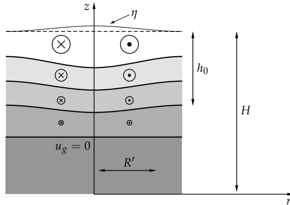
13.1. ábra. Óceáni áramlat közel geosztrofikus meleg gyűrűinek sematikus (a z tengely körül forgásszimmetrikus) sűrűség- és sebességeloszlása, f_0 > 0 . A gyűrű vízszintes mérete belső Rossby-sugár nagyságrendű. Kétrétegű közegben ennek a 6.5b. ábra felel meg.
