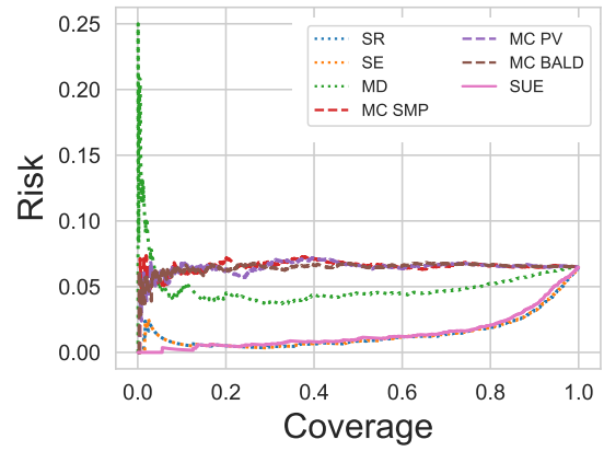
(a) Twitter
