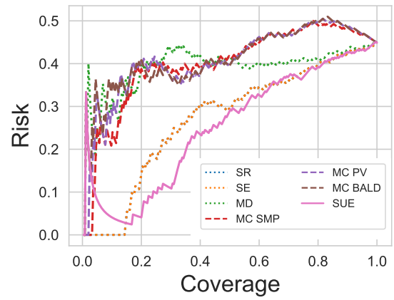
(b) MRPC
