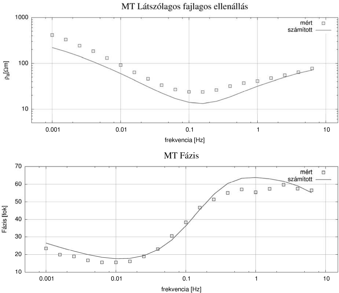
9. ábra. A magnetotellurikus görbék illeszkedése a 116 km-nél levő szondázási pontnál a 8. ábrán bemutatott inverzió esetében
