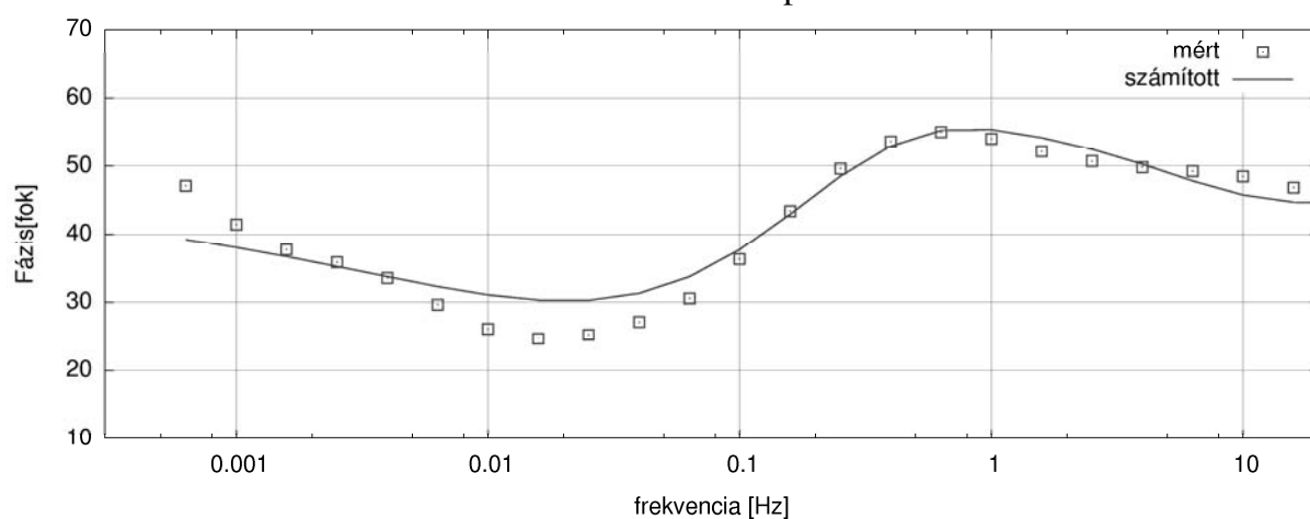
13. ábra. A magnetotellurikus görbék illeszkedése a CEL-7 18 km-es pontjánál
