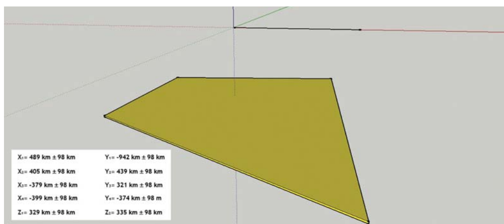
12. ábra Az optimalizálással meghatározott modell elhelyezkedése Descartes-féle koordináta-rendszerben, amikor a paraméterek Laplace-féle eloszlásúak, a szélsőérték-keresés simplex módszerrel történt. Az ábra táblázatos formában megadja a meghatározott paraméterek értékét és a paraméterek maximális hibáit
