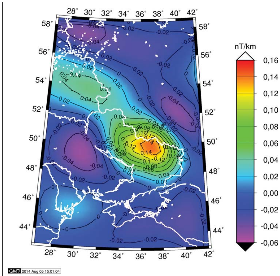
8. ábra A kurszki totális mágneses anomáliák (1. ábra) vertikális irányú gradiense a CHAMP méréseiből levezetve, 324 km magasságban, Albers-féle vetületben ábrázolva. Az izovonalak egysége nT/km, értékükük 0,02 nT/km Figure 8 Vertical gradient of the Kursk magnetic anomalies (Fig. 1) computed from the CHAMP data with a contour interval 0.02 nT/km (Albers' projection) anomaly range is given by 11 color levels
