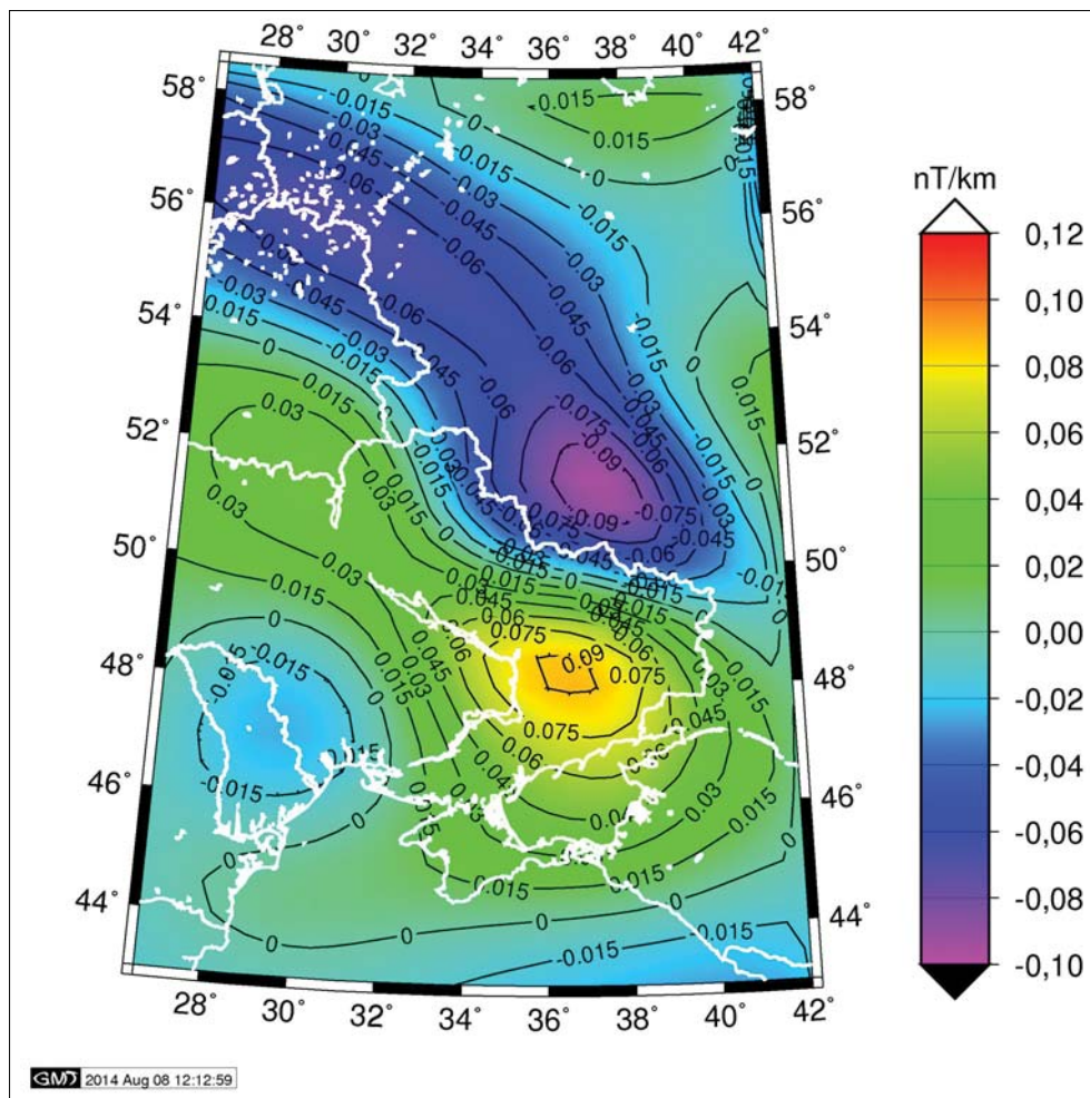
6. ábra A kurszki totális mágneses anomáliák (1. ábra) északi irányú gradiense a CHAMP méréseiből levezetve, 324 km magasságban, Albers-féle vetületben ábrázolva. Az izovonalak egysége nT/km, értékükük 0,015 nT/km Figure 6 North gradient of the Kursk magnetic anomalies (Fig. 1) computed from the CHAMP data on an Albers' projection the contour interval is 0.015 nT/km, anomaly range is given by 11 color levels
