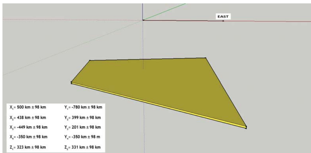
10. ábra Az optimalizálással meghatározott modell elhelyezkedése Descartes-féle koordináta-rendszerben, amikor a paraméterek Gauss-féle eloszlásúak, a szélsőérték-keresés simplex módszerrel történt. Az ábra táblázatos formában megadja a meghatározott paraméterek értékét és a paraméterek maximális hibáit
