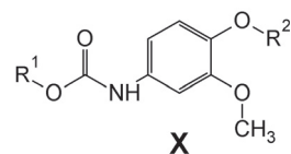
1. Ábra. Az X általános képletű molekulaváz.
