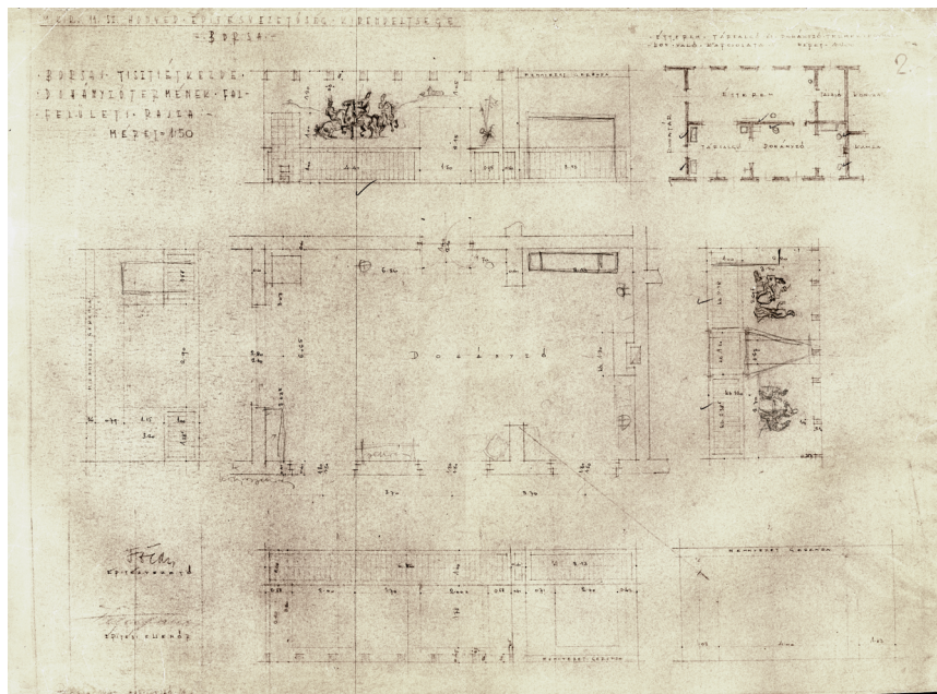
1. kép. A borsai határvadász-laktanya tiszti étkezdéje: az étterem, társalgó- és dohányzóterem alaprajza – kinagyítva a dohányzóhelyiség. Az épület falfelületi rajzaira Chiovini Ferenc leadott és jóváhagyott tervei, a Magyar Királyi 11. számú Honvéd Építésvezetőség Kirendeltsége számára, 1:50-es méretarányban (1942.08.16.) (487/658-as sorszámú tervdokumentáció, 2. oldal, forrás: Chiovini családi archívum)
