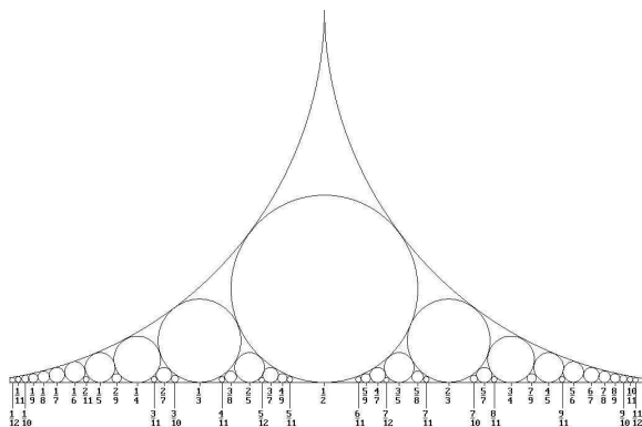
Ford-körök
