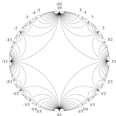
A Farey-gráf
