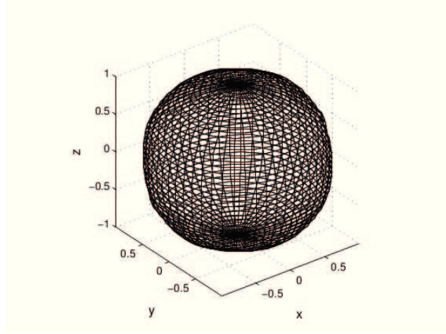
3. ábra. A 3. fejezetben bemutatott véletlen norma háromdimenziós gyenge kiterjesztéséből származtatott várható érték norma egységgyömbje ( n = 100 , \lambda_n = 100 , N = 500 ) paraméter beállítások mellett.
