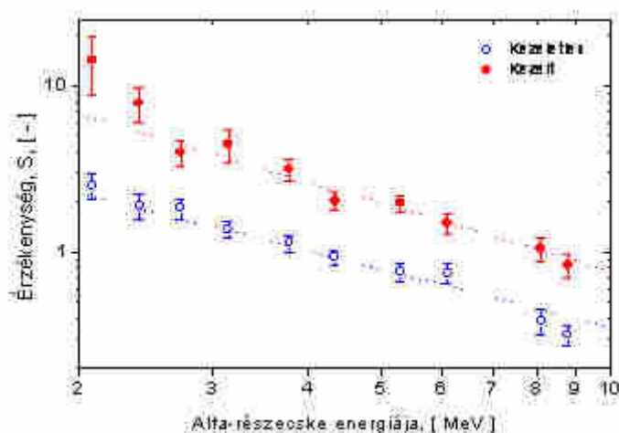
3. ábra. A TASTRAK PADC detektor alfa-részecske válaszfüggvénye kezeletlen és maratás előtt 45 percen át 100°C-os vízben való előkezelés esetén. (Maratás 70°C-on 5 órán át.)
