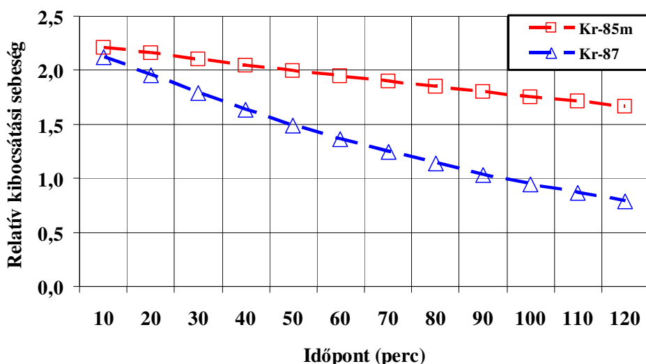
10. ábra A 4,45 órás felezési idejű ^{85\text{m}}\text{Kr} és az 1,27 órás felezési idejű ^{87}\text{Kr} kibocsátása a ^{85}\text{Kr} kibocsátására normálva, az első két órában
