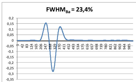
9. ábra. ^{133}\text{Ba} spektrum második deriváltja
