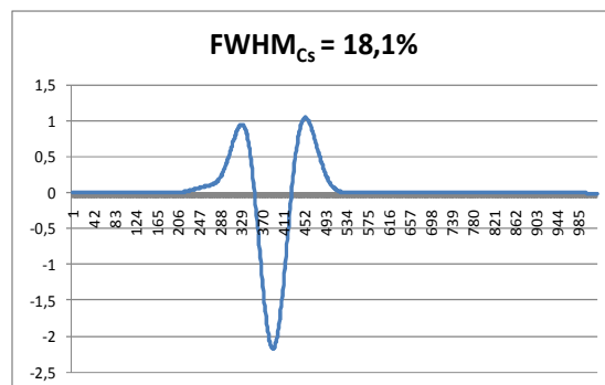
10. ábra. ^{137}\text{Cs} spektrum második deriváltja
