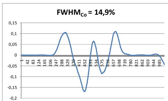
11. ábra. ^{60}\text{Co} spektrum második deriváltja
