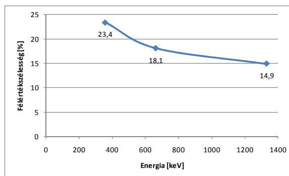
12. ábra. A félértékszélesség energiafüggése
