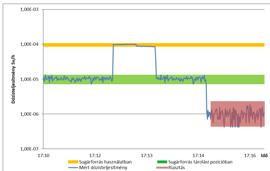
3. ábra Sugárkapu algoritmus alkalmazása sugárforrások felügyeletére. Forrás: [7]
