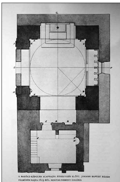
2. kép. A Bakócz-kápolna Pácz János féle alaprajza a bontás és az újjáépítés előtt (1823) (Horler 1987)
