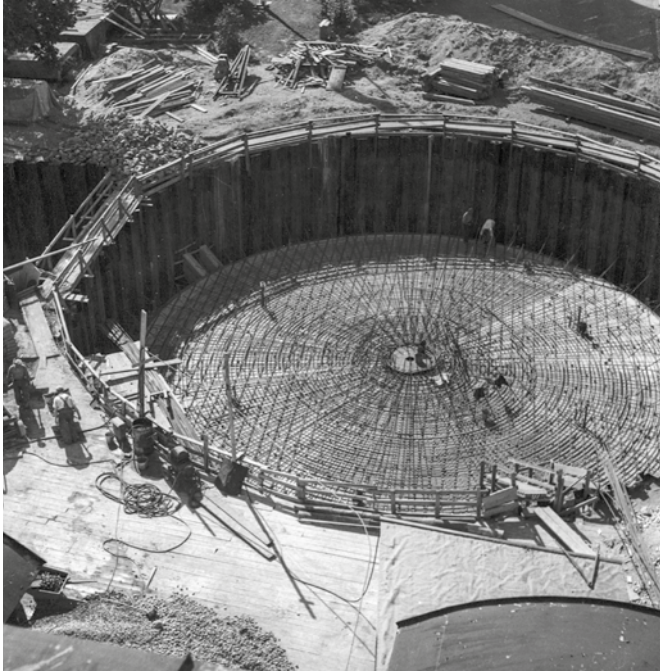
245. kép. A Központi Fizikai Kutatóintézet atomreaktorának építése az 1950-es években...
