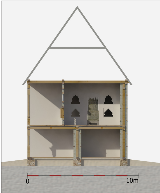
15. kép. A palotaépület rekonstruált keresztmetszete. Szolnok–Vár, 16. század második fele (3D modell: Szőke B.)
