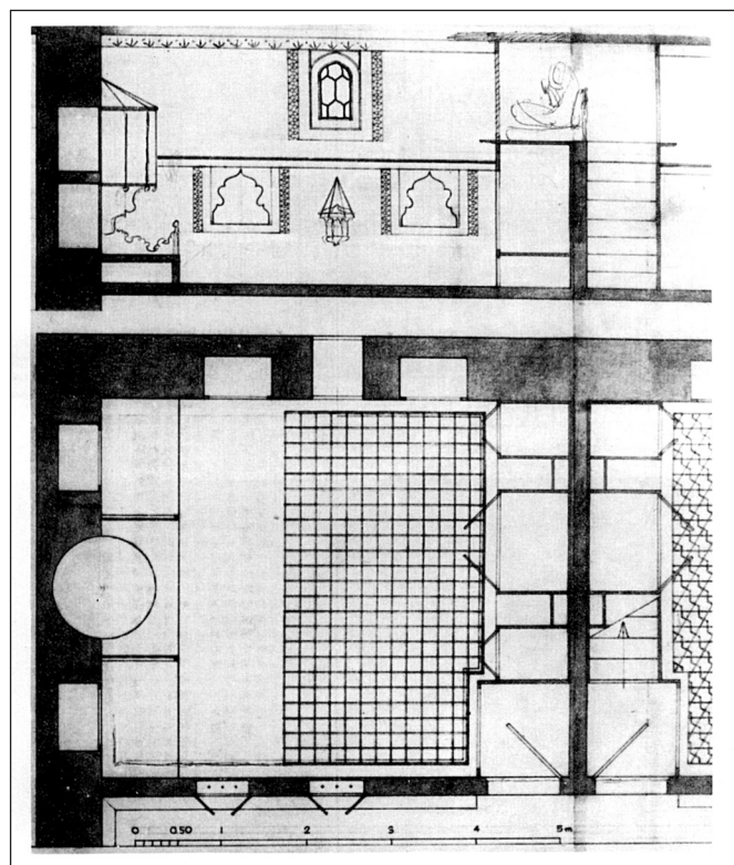
23. kép. A Sarayönü mahalléban álló épület egyik emeleti odájának metszete (fent) és alaprajza (lent). Bursza, Törökország, 16. század közepe (ELDEM 1984, 51)
