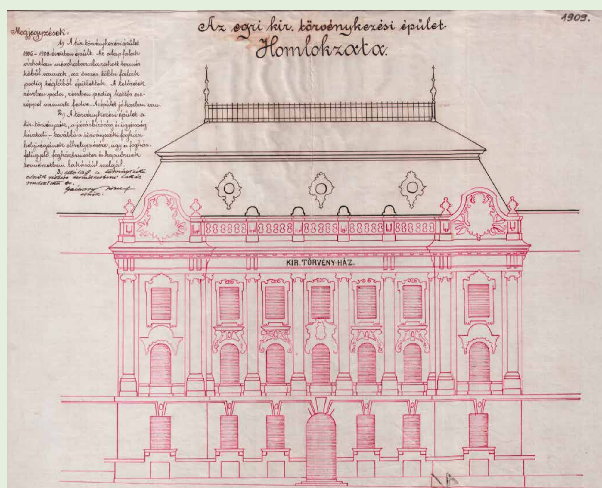
Az épület főhomlokzatának részlete a kiviteli terveken. (Egri Törvényszék Irattára)
