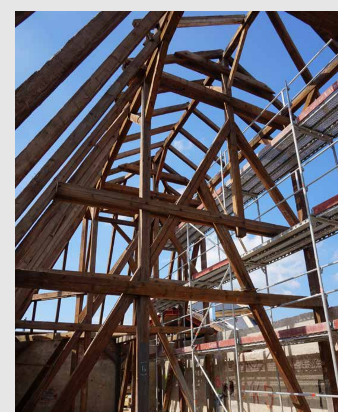
A Törvényszék tetőzetének átépítése. (Megyeri-Pálffi Zoltán fotója)
