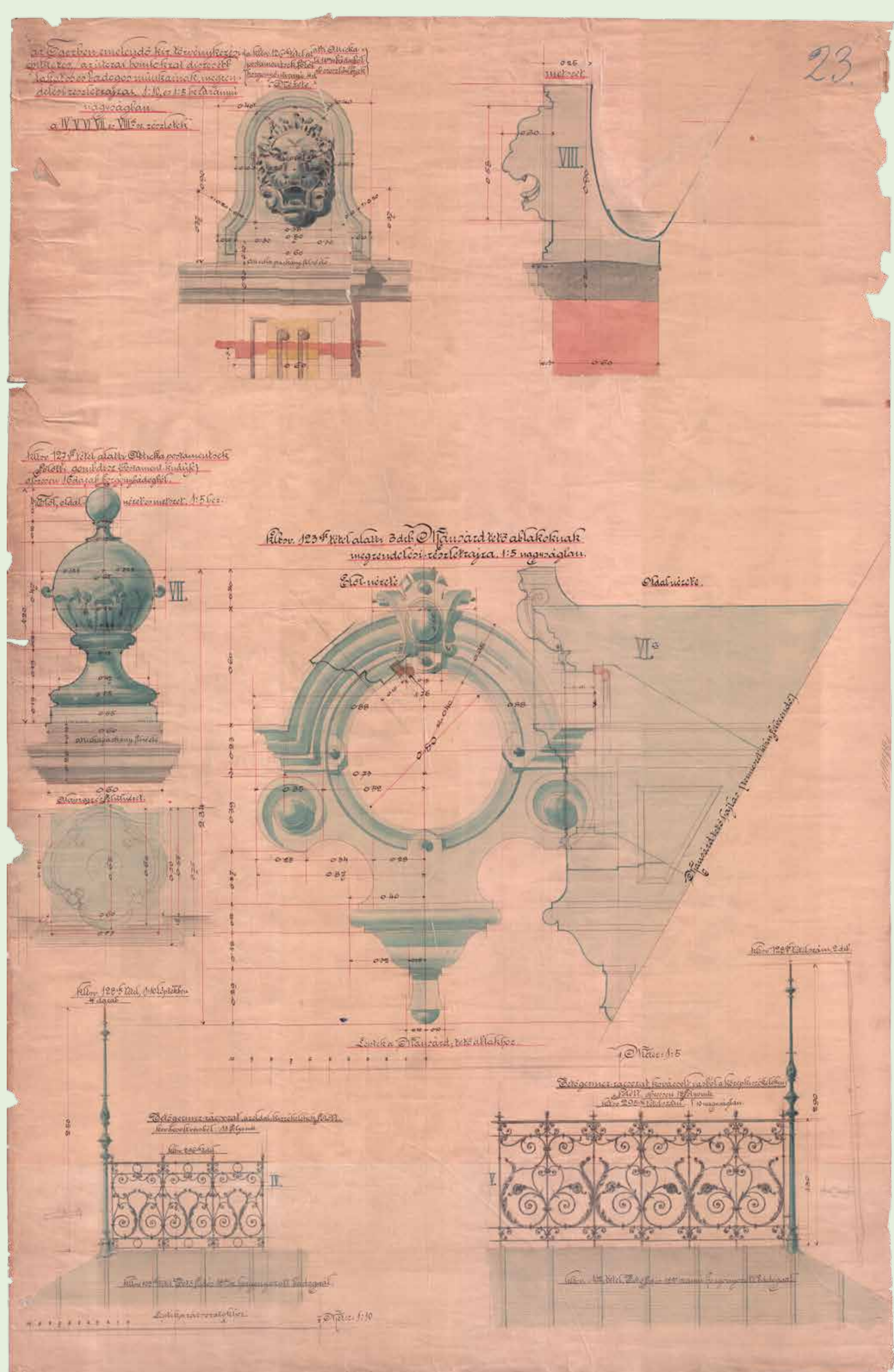
A Törvényszék tetődíszének eredeti részlettervei Wágner Gyulától. (Egri Törvényszék Irattára)
