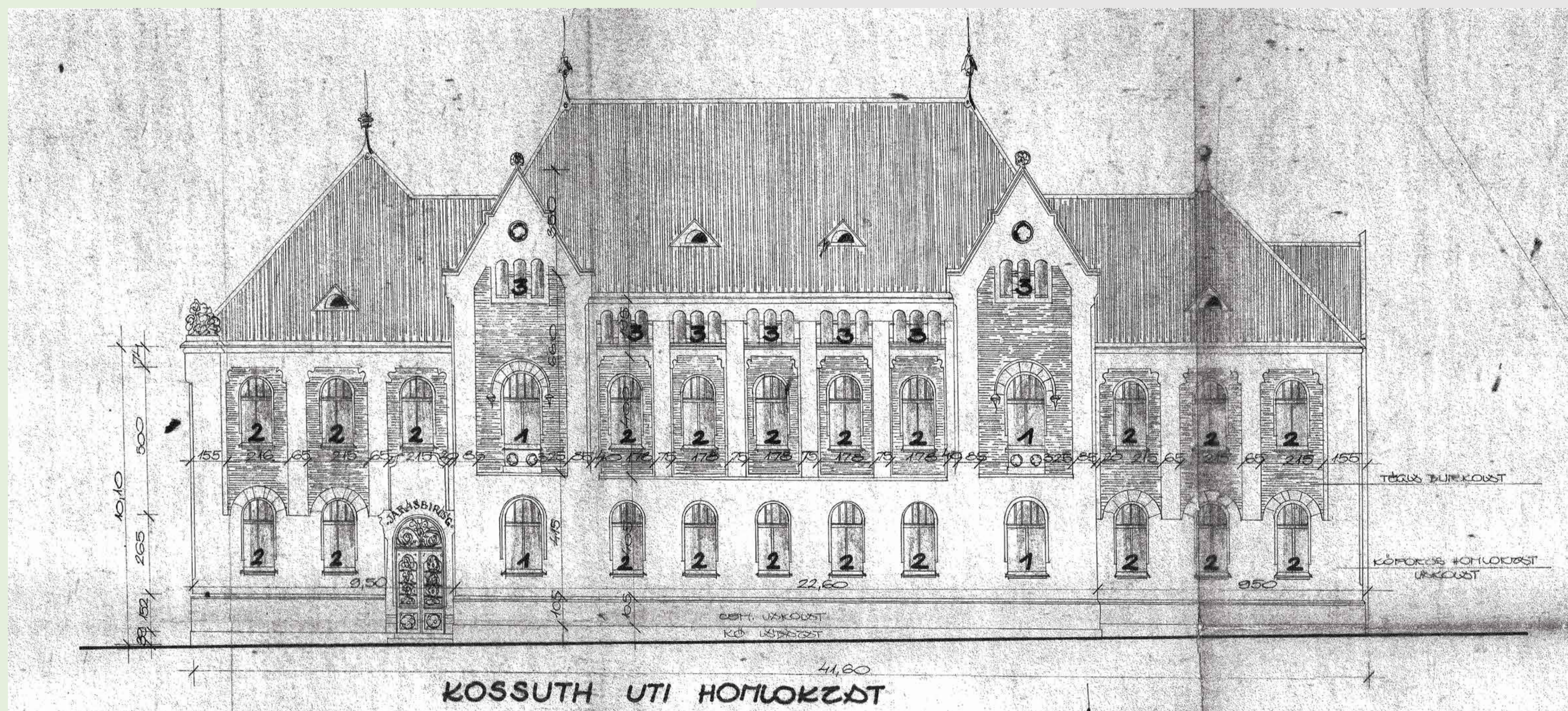
A Gyöngyösi Járásbíróság homlokzati felújítási terve 1973-ból. (Gyöngyösi Járásbíróság Irattára)
