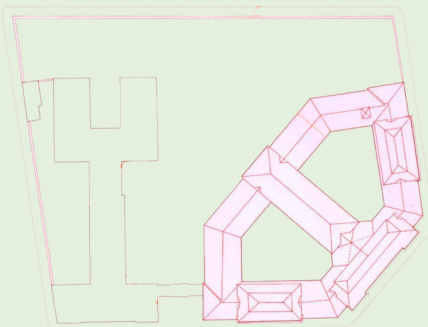
Helyszínrajz az egri igazságügyi épületkomplexumról. A telek baloldalán a törvényszéki fogház, a jobb oldalán a hátszögletű Törvényszék helyezkedik el. (OBH Műszaki Főosztály Irattára)
