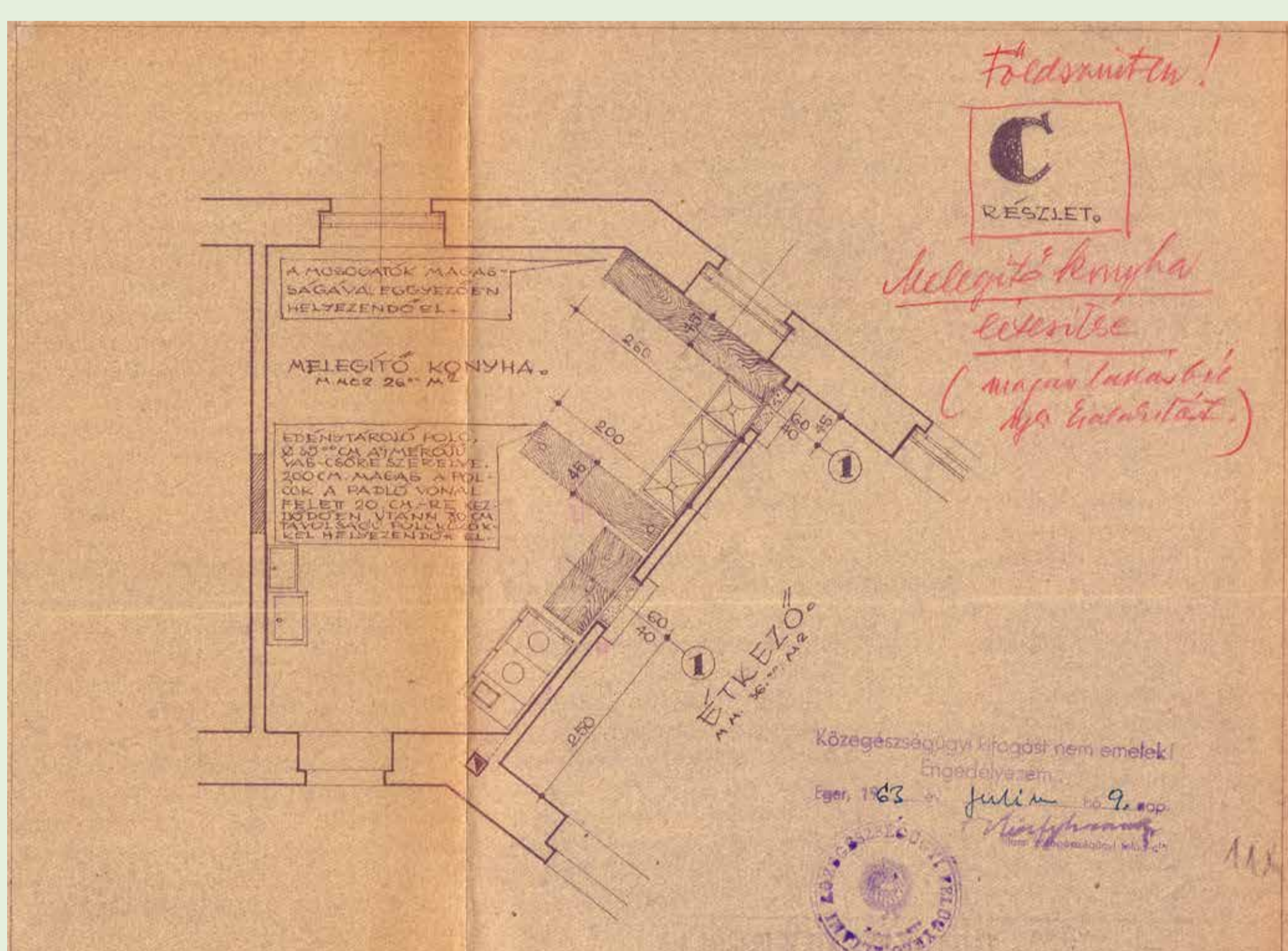
Melegítő konyha kialakításának 1961-ben készült terve a Törvényszék épületében. (OBH Műszaki Főosztály Irattára)
