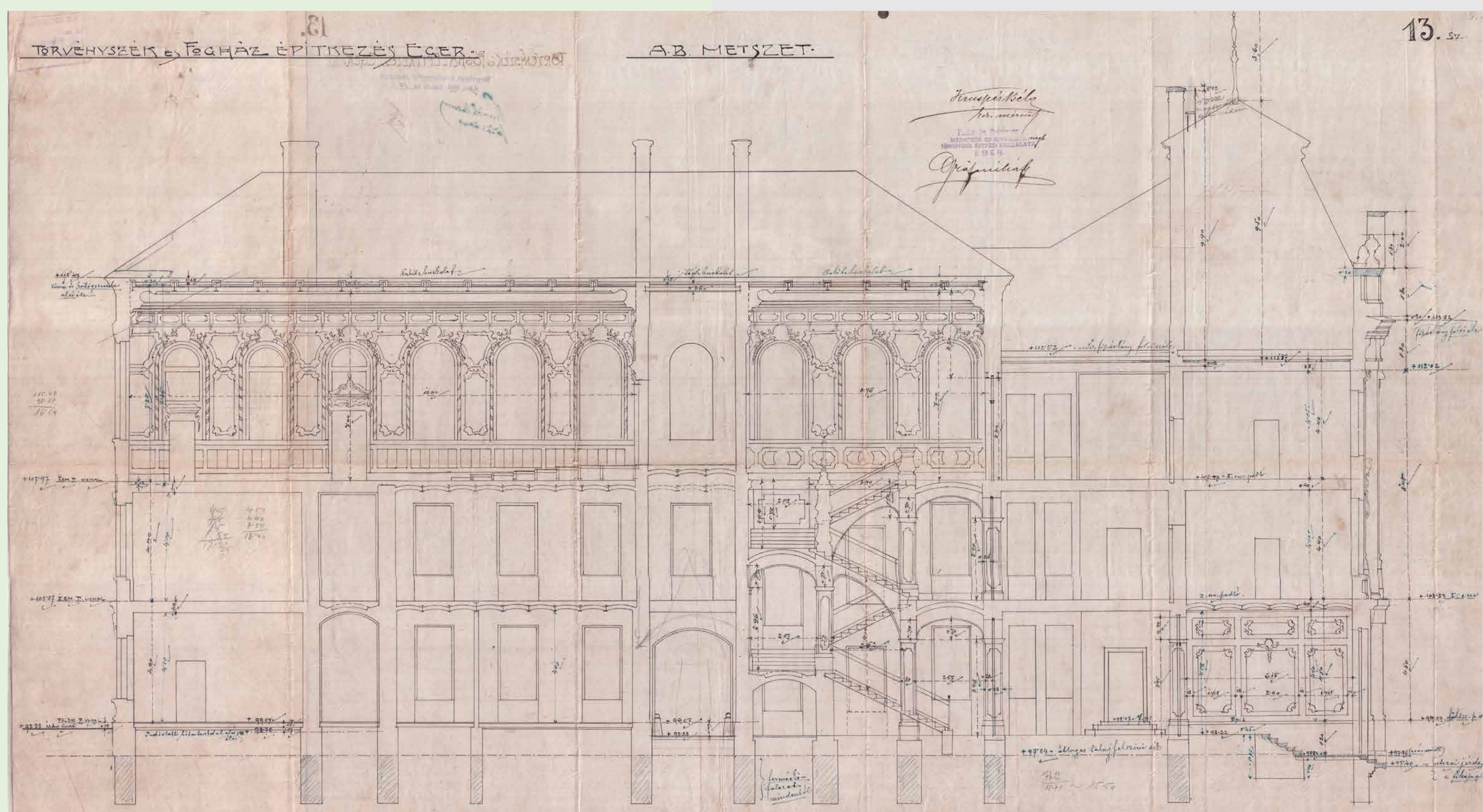
Az épület esküdtzéki terménél átfelvett metszeti rajza a kiviteli terveken. (Egri Törvényszék Irattára)
