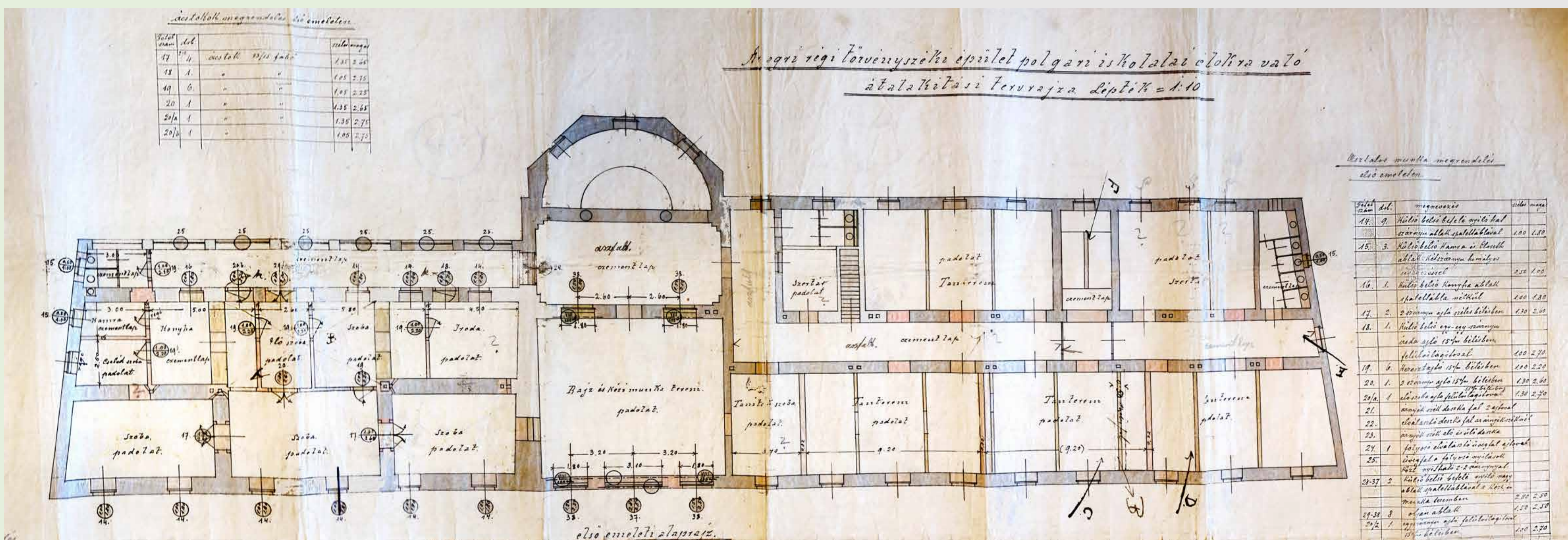
Az Oroszlán és az 1883-as járásbírósg épület átalakítási terve iskoláivá 1911-ből, miután a bíróságot átköltözték a Törvényházba. (MNL HML)
