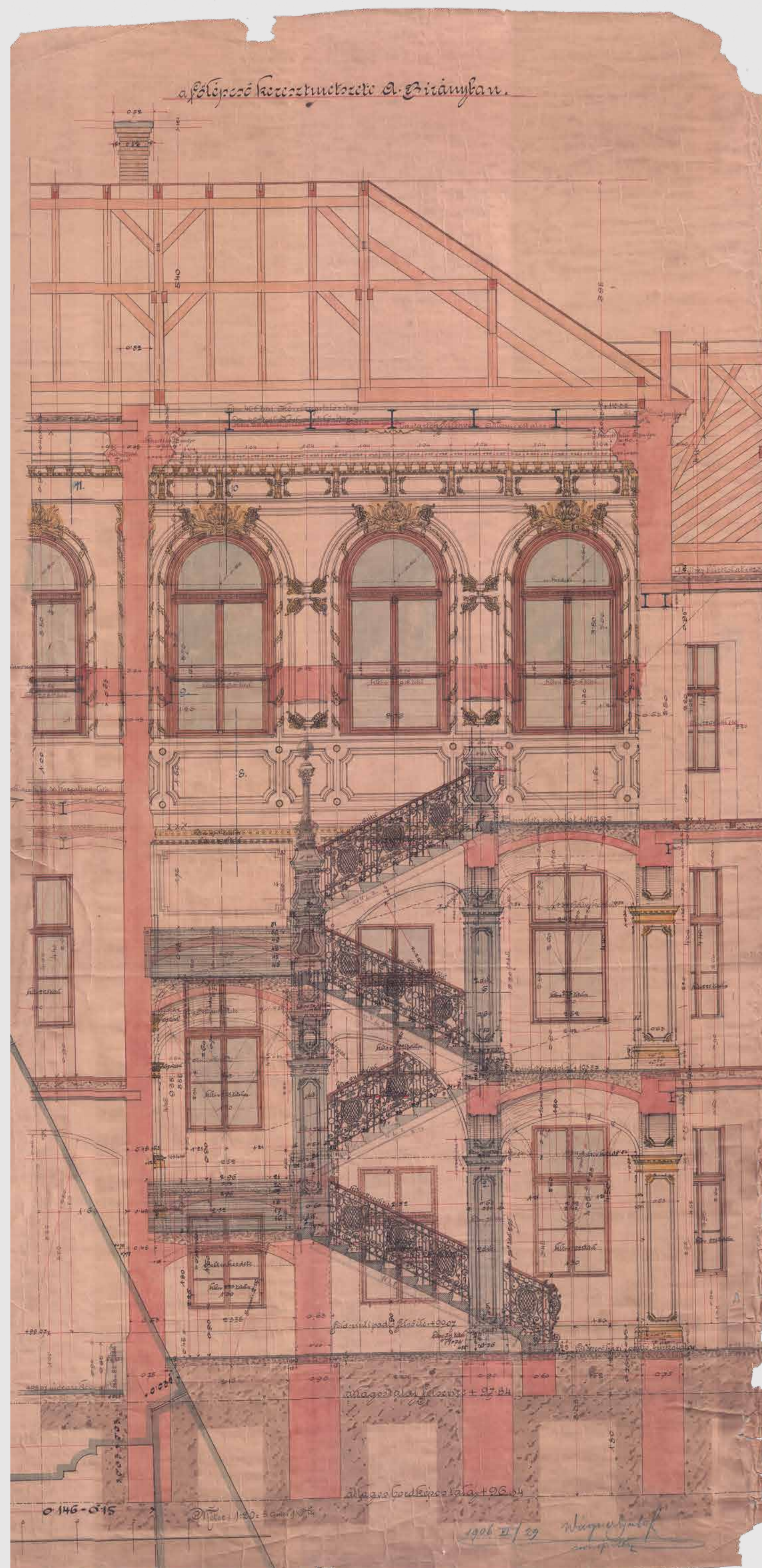
A Törvényszék díszlépcsőházának metszete Wágner Gyula eredeti tervén. (Egri Törvényszék Irattára)
