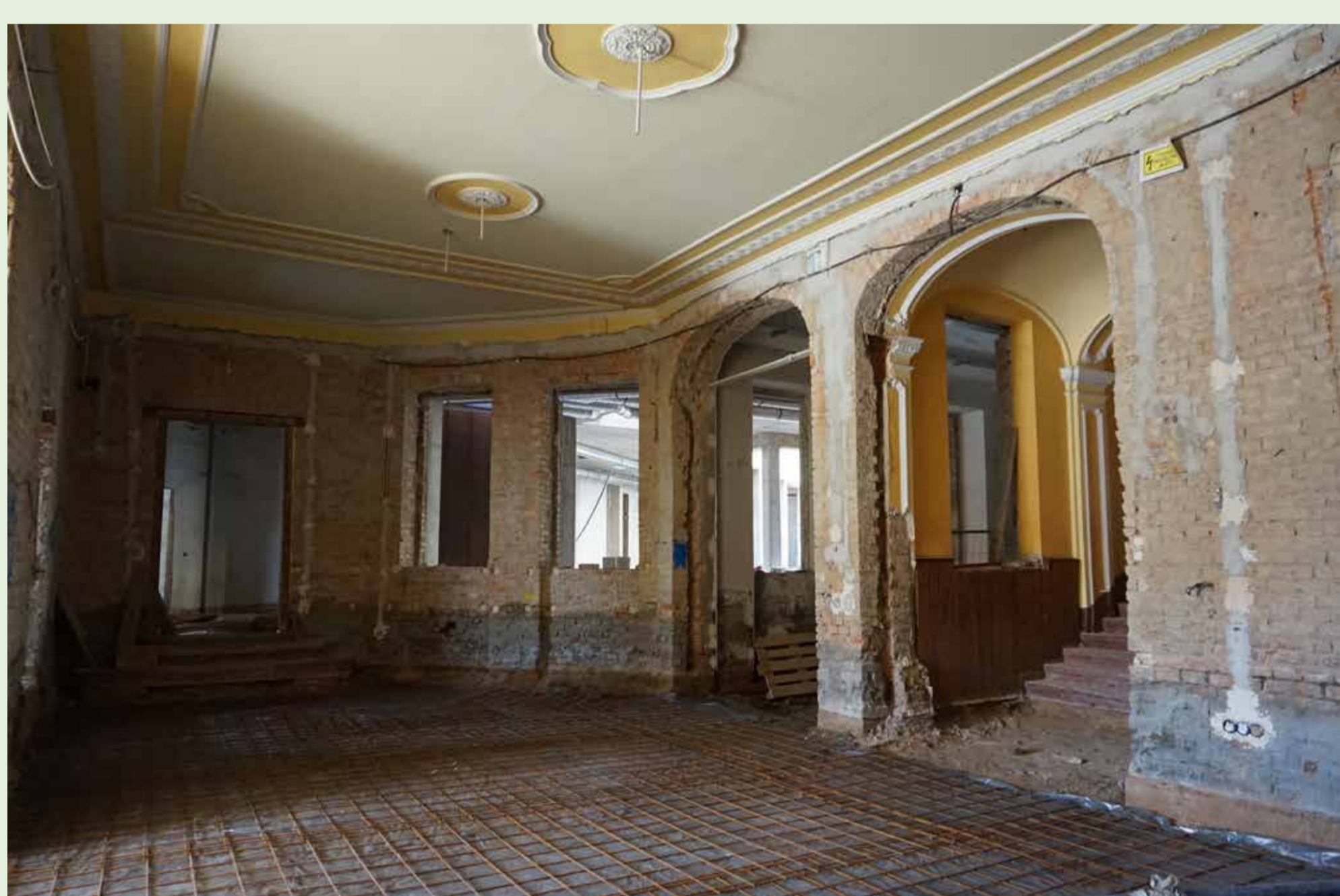
A Törvényszék előcsarnokának rekonstrukciós munkálatai. (Megyeri-Pálffi Zoltán fotója)
