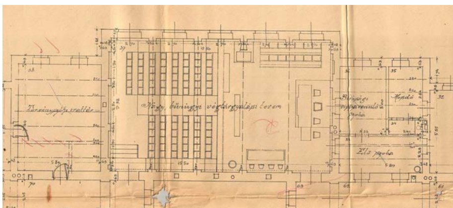
6. kép. A nagy tárgyalási terem alaprajza. Részlet az eredeti tervből.
