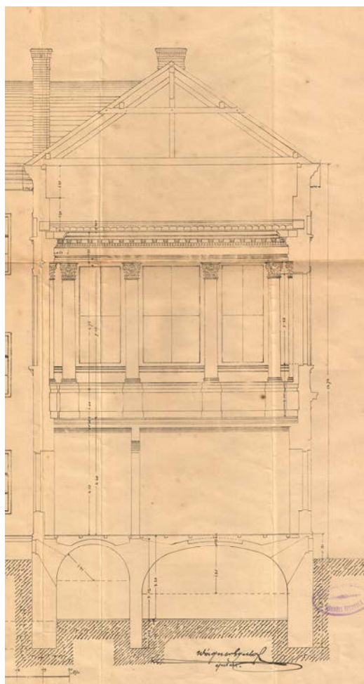
4. kép. A nagy tárgyalási terem metszete. Részlet az eredeti tervből.
