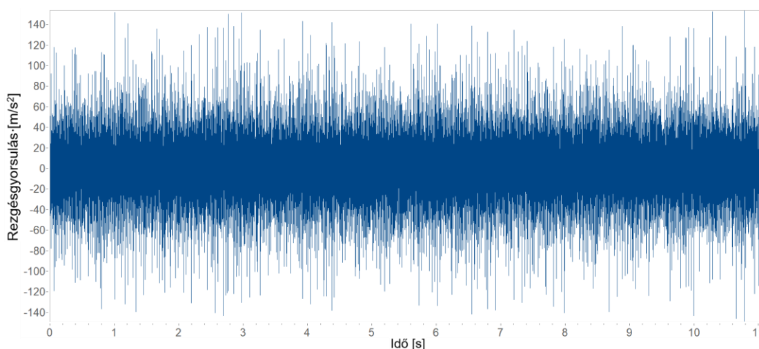
4. ábra: A hátsó markolatnál található y irányú rezgés
