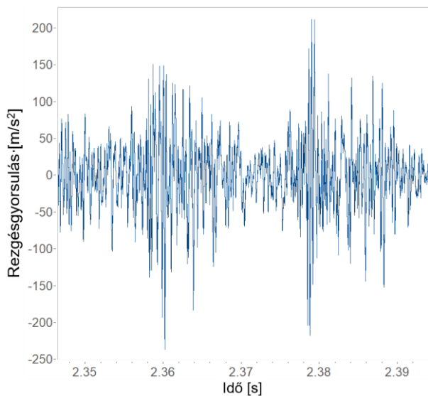
6. ábra: A vágópengék gyorsulása az excenteres mechanizmus működése közben y irány mentén
