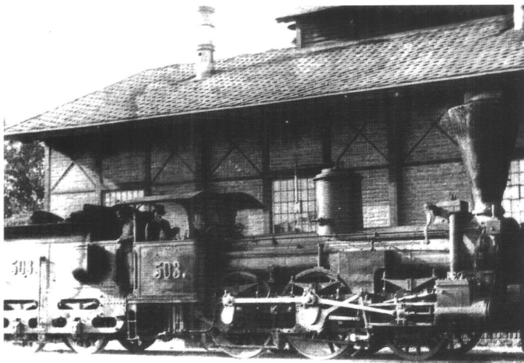
A Déli vasút egyik 1858-59-ben készült személyvonati mozdonya Ismeretlen fényképező
