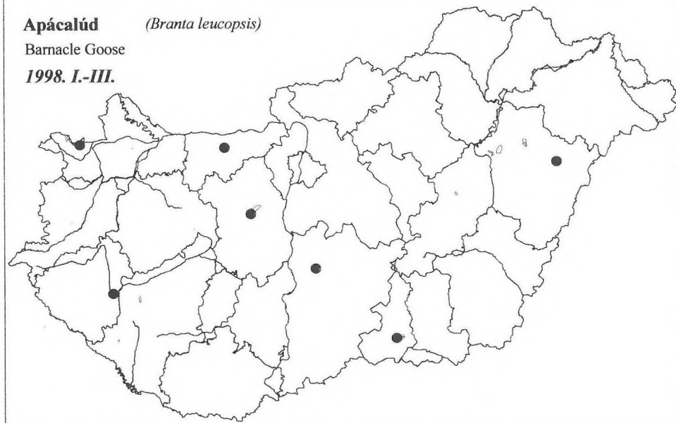
7. térkép: Az apácalúd előfordulása Magyarországon 1997/1998.
