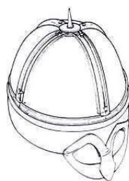
7. ábra A Gjermundhu-i (nyugati típusú) sisak szerkezete.
