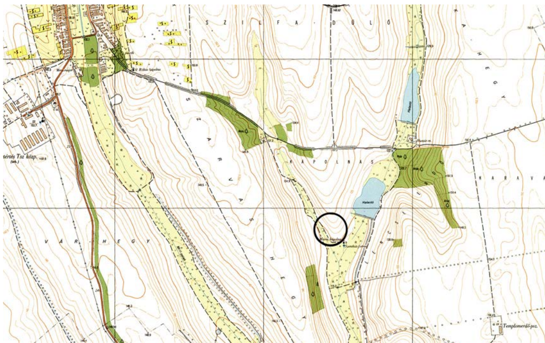
19. kép. Palotabozsok-Kirchegrund (1:10 000)
