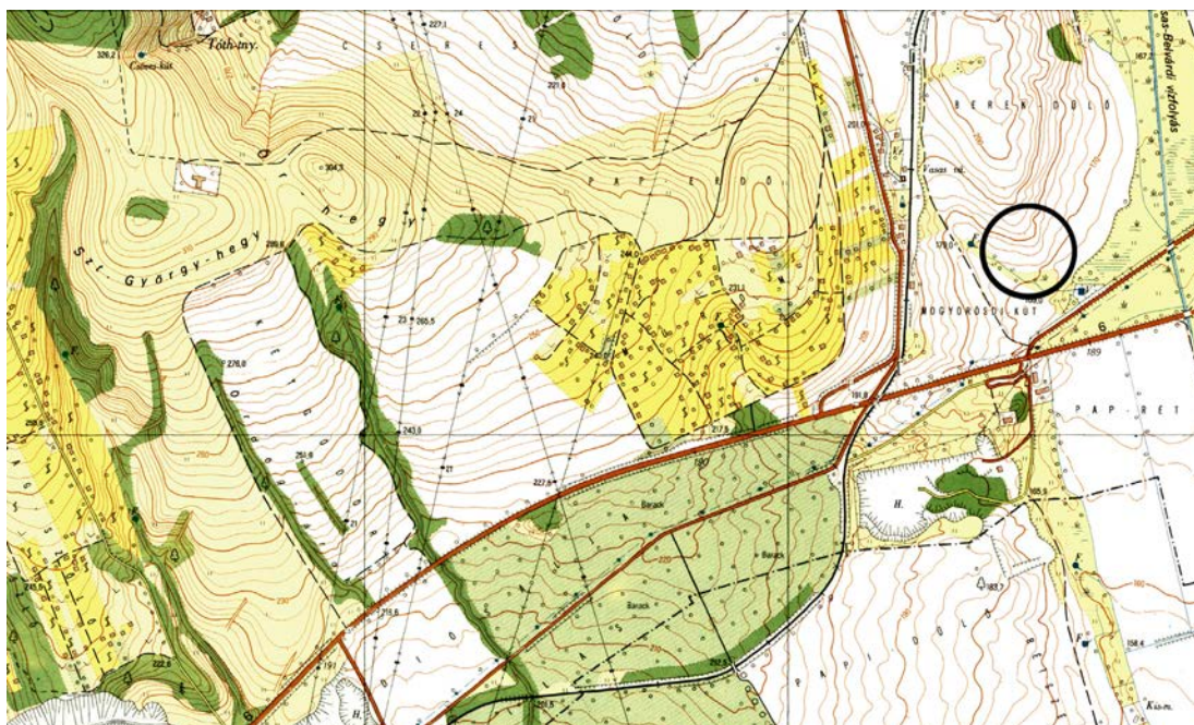
24. kép. Pécs-Somogy/Vasas (1:10 000)
