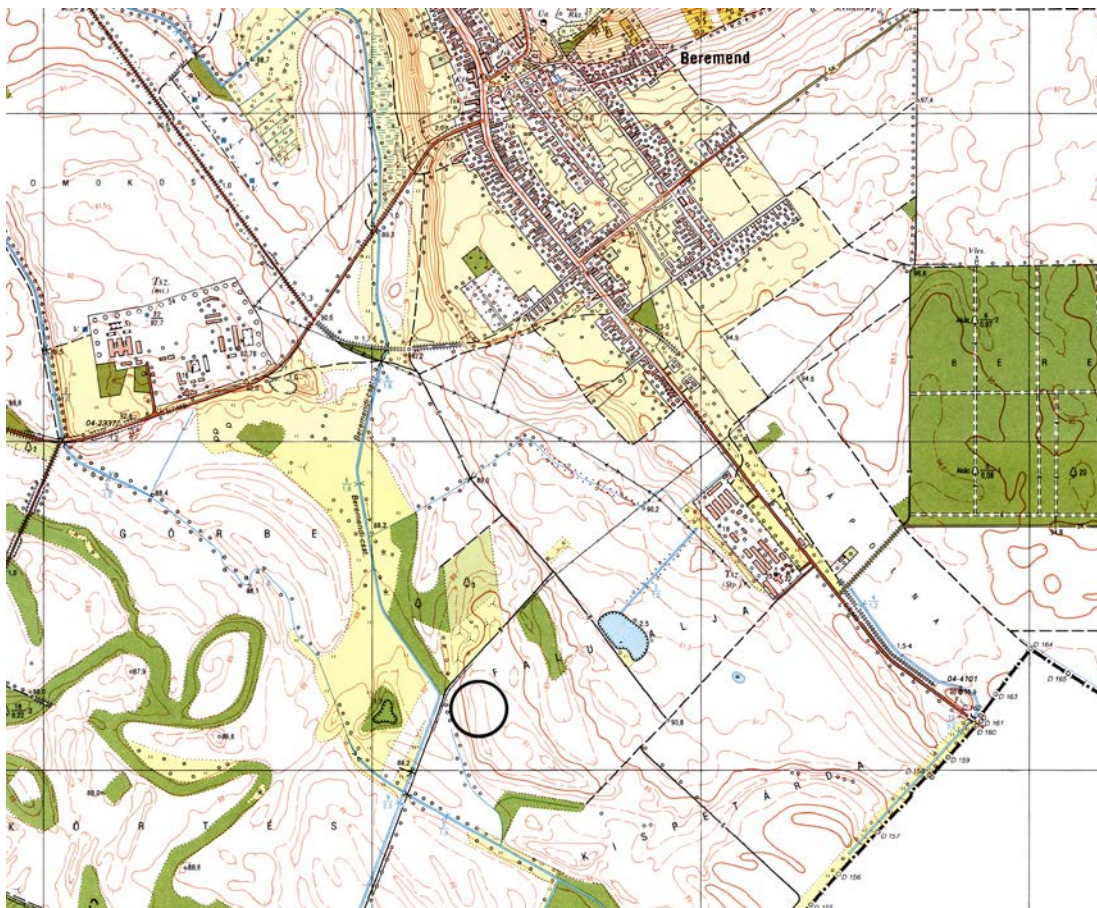
1. kép. Beremend-Homokbánya (1:10 000)
