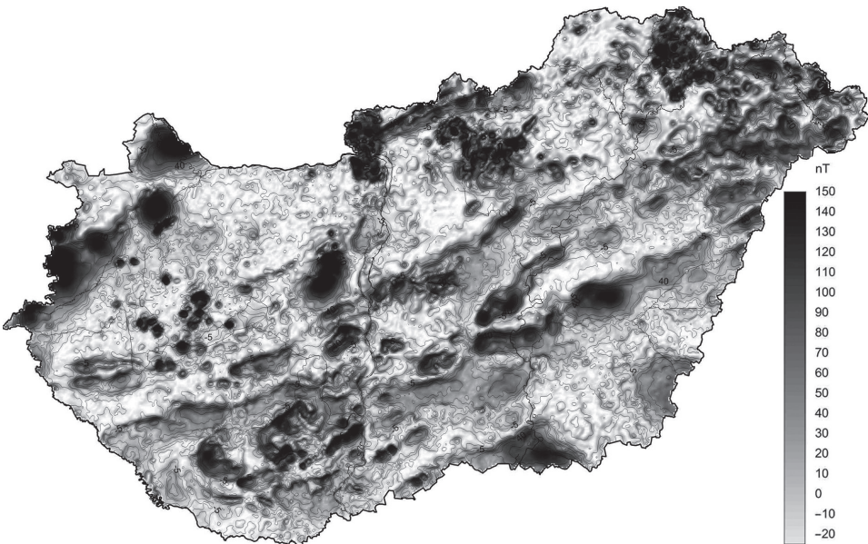
13. ábra. Mágnesesanomália-térkép (a szerző szerkesztése)
