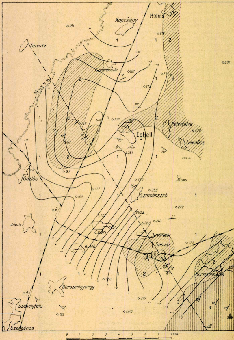
3. rajz. Egbell környékének geológiai térképe az isogammákkal.
