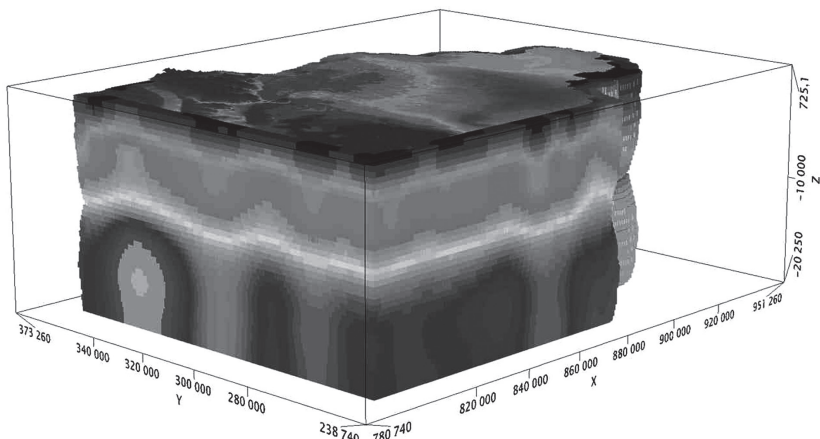
10. ábra. A relatív sűrűség háromdimenziós térrácsa, Nyírség (a szerző szerkesztése)
